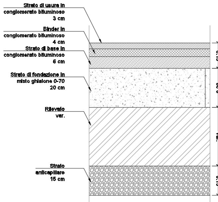
Figura 7 - Pavimentazione carrabile
