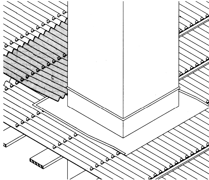
Fig.5 – Raccordo a camino
