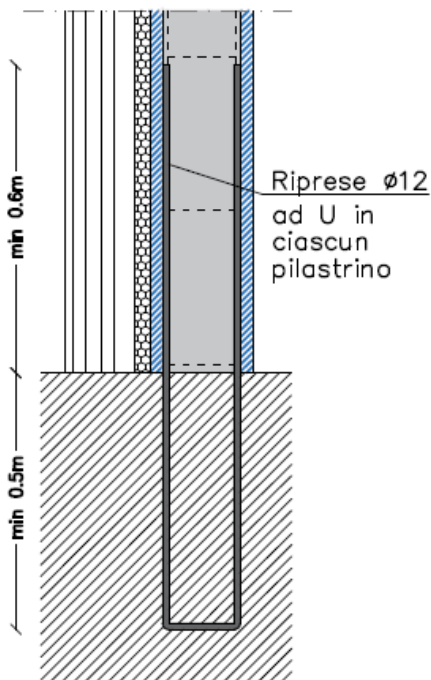
Tipologico riprese armature verticali
