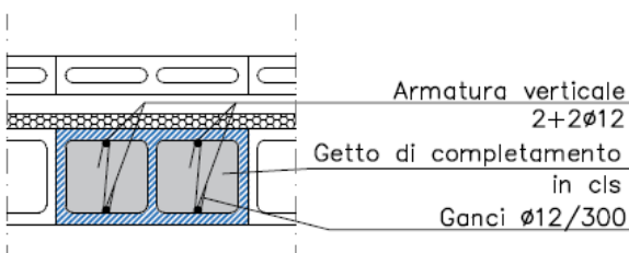
SEZIONE DD – Tipologico pilastro Muratura perimetrale
