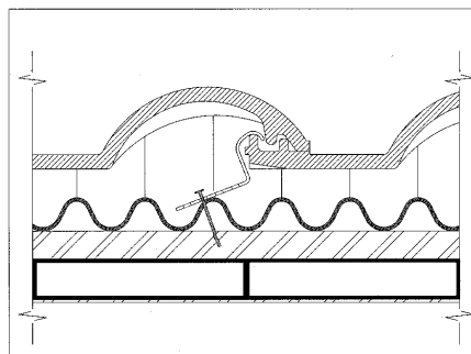
Fig.4 – Particolare tipologico del fissaggio della prima fila di tegole
