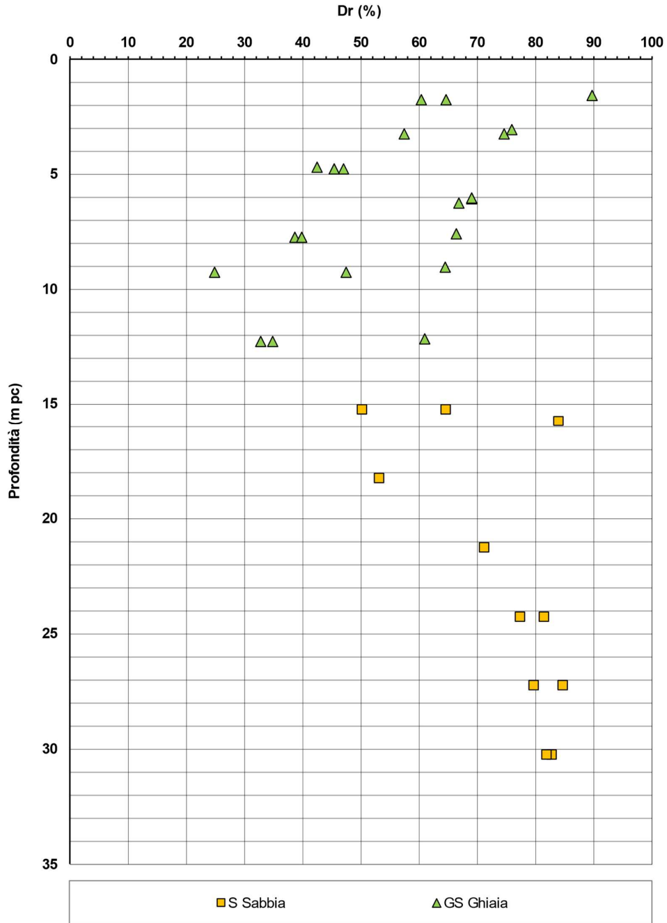
Figura 6 – Densità relativa da prove SPT tra pk 3+160 a pk 3+700
