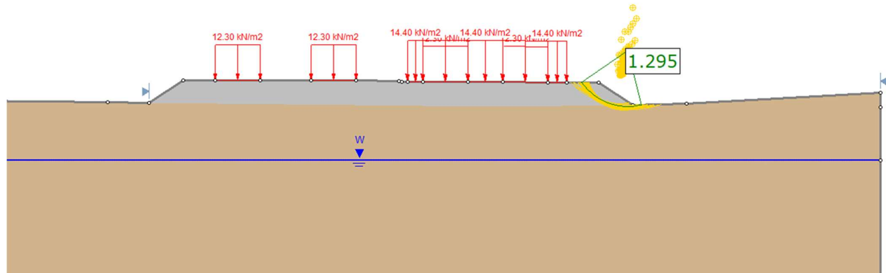
Figura 16 - Rilevato H=1.70 m (da pk 3+160 a pk 3+700) - Analisi SLU in campo sismico
