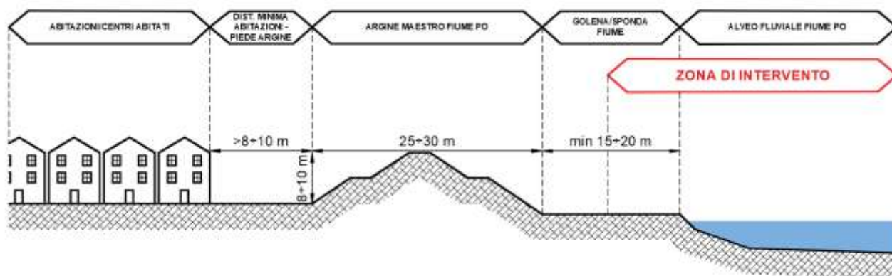
Figura 24 - Schema sezione argini maestri fiume Po
