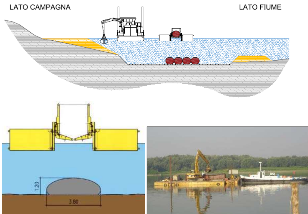
Figura 5 - Pontone con cassone apribile (sx) e treno di varo per posizionamento corretto (dx)
