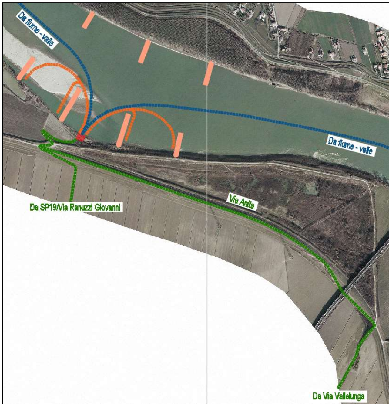
Figura 23 - Planimetria degli accessi all'area di cantiere INTERVENTO 15 – SPONDA DESTRA
