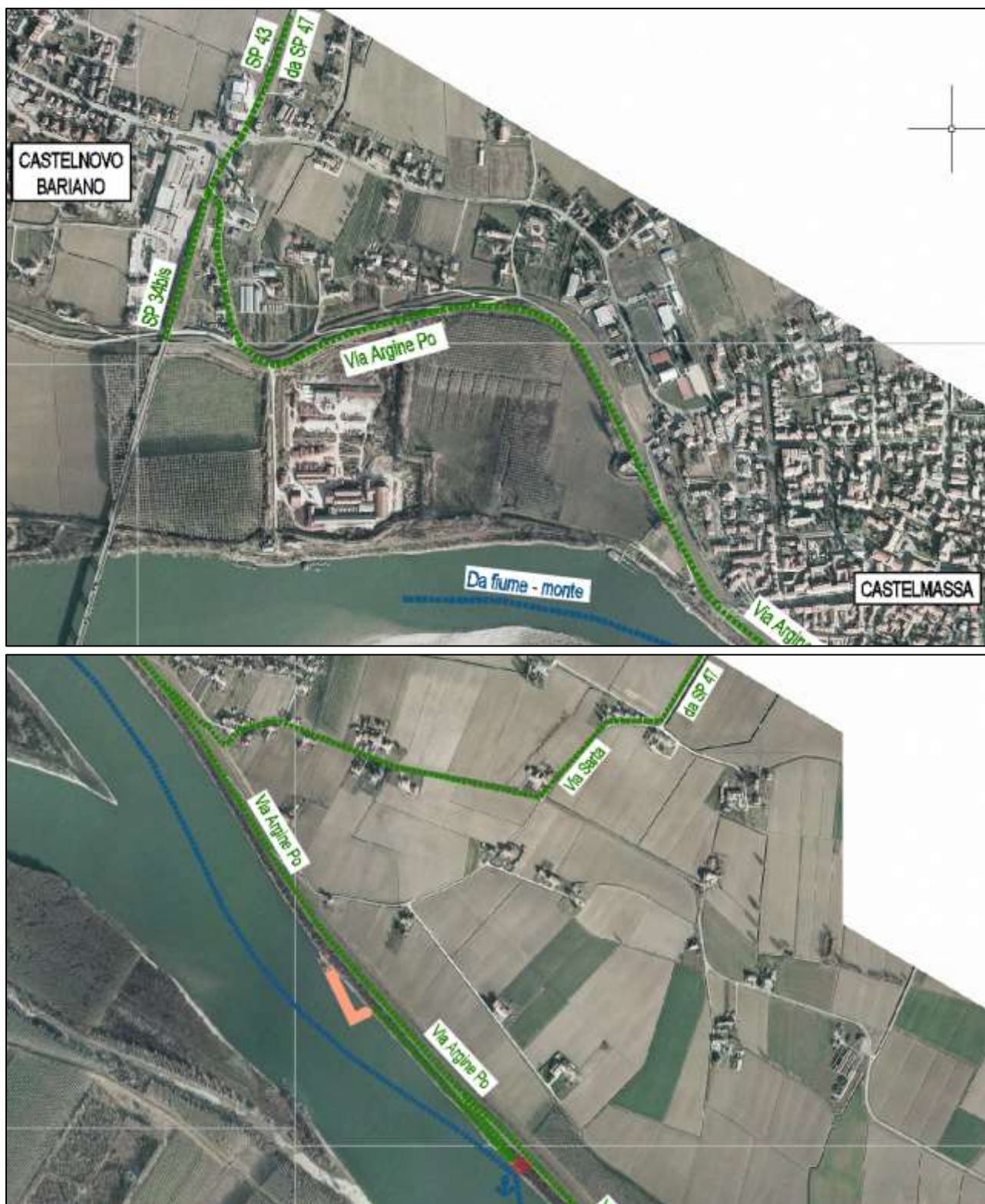
Figura 8 - Planimetria degli accessi all'area di cantiere INTERVENTO 2
