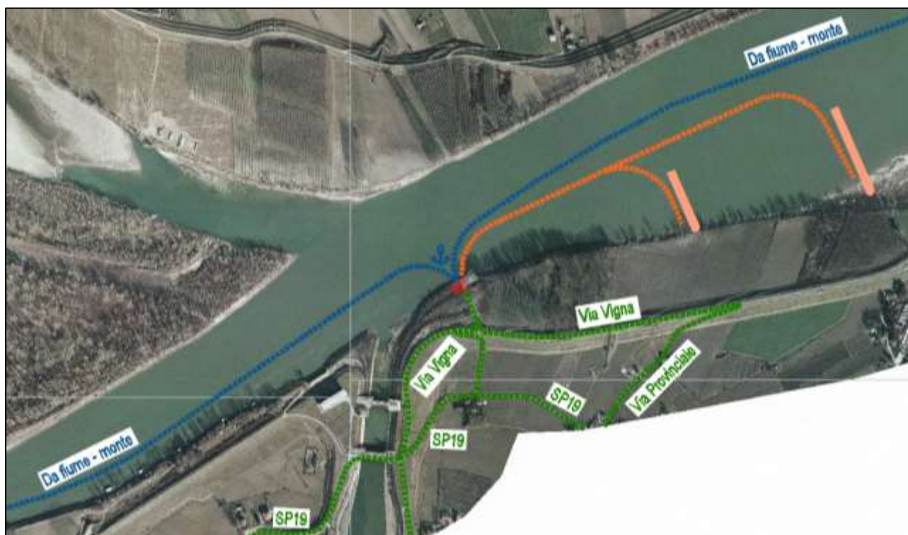
Figura 16 - Planimetria degli accessi all'area di cantiere INTERVENTO 9
