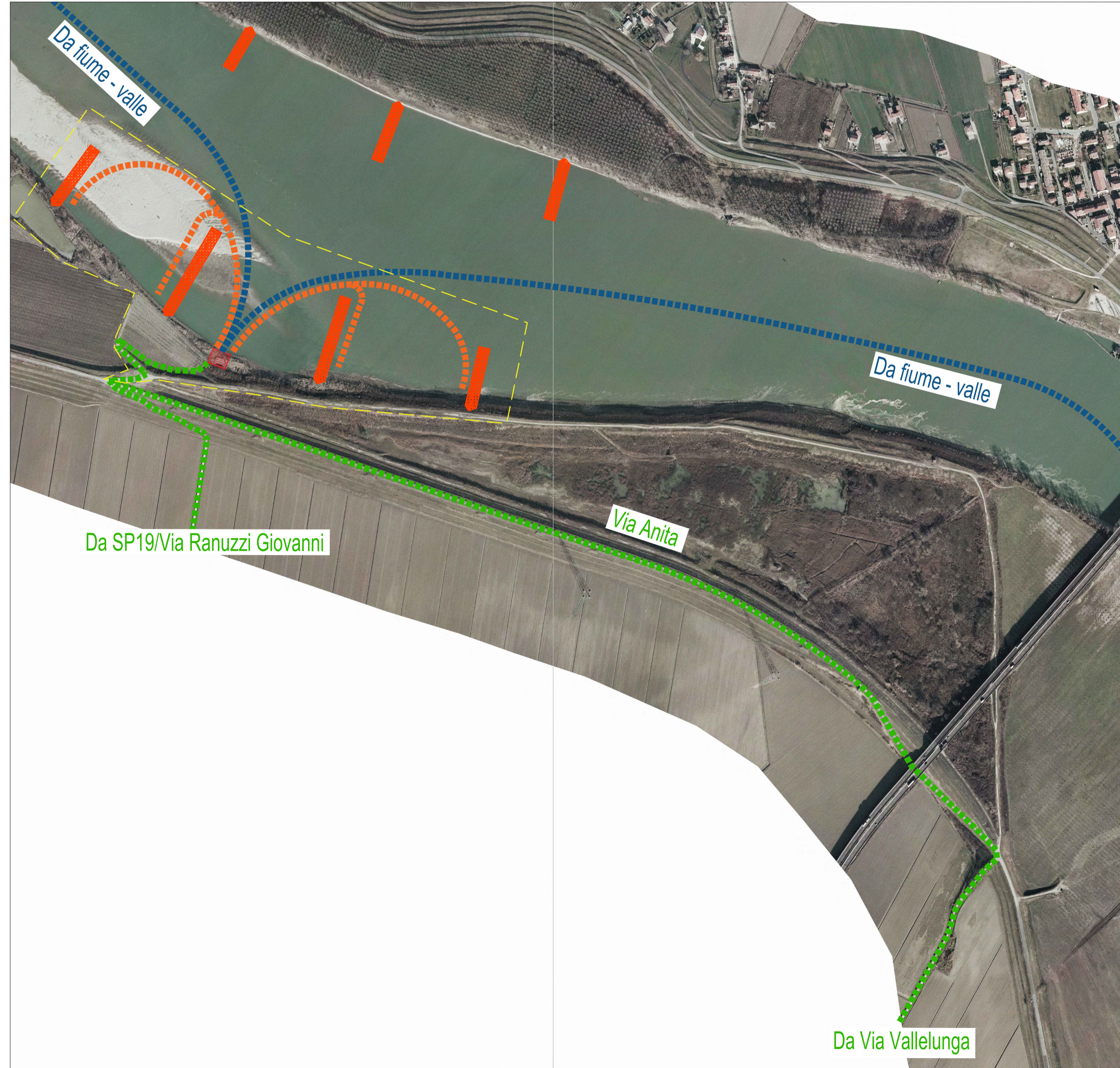
GRUPPO DI INTERVENTO N°15 - SPONDA DESTRA - PLANIMETRIA DI ACCESSO AL CANTIERE - SCALA 1:5000
