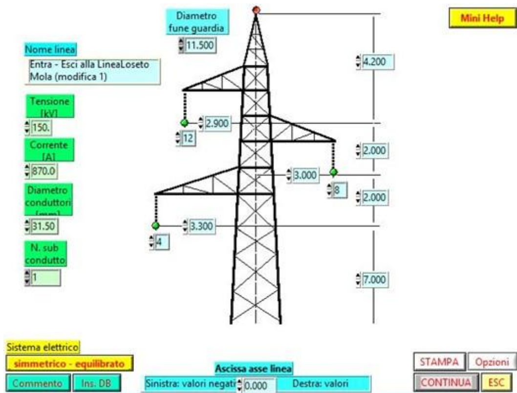
Figura 1: Sostegno con Configurazione a Triangolo
