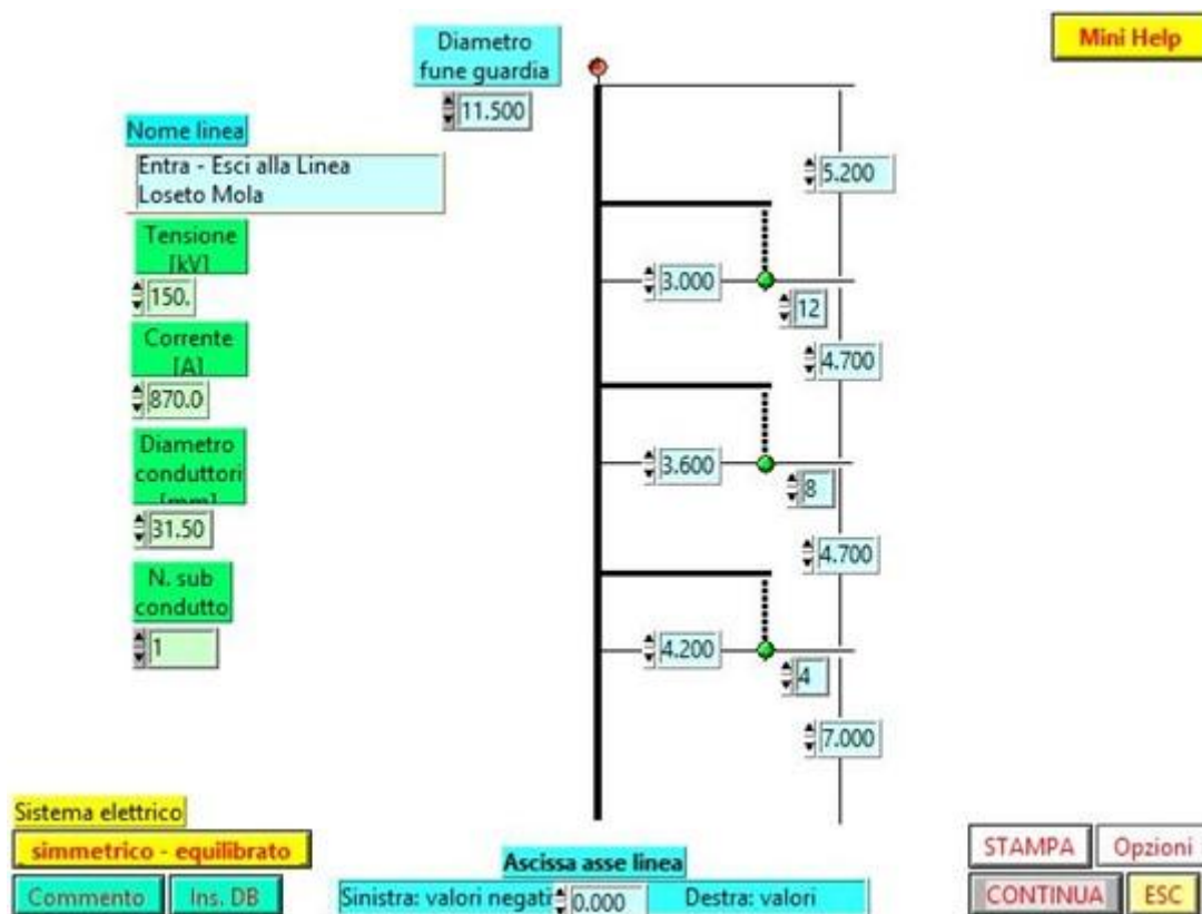
Figura 2: Sostegno con Configurazione a Bandiera
