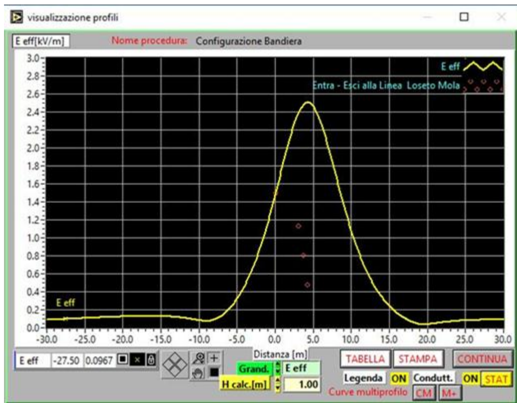
Figura 4 : Valutazione del Campo Elettrico ad 1 m dal suolo, Configurazione a Bandiera
