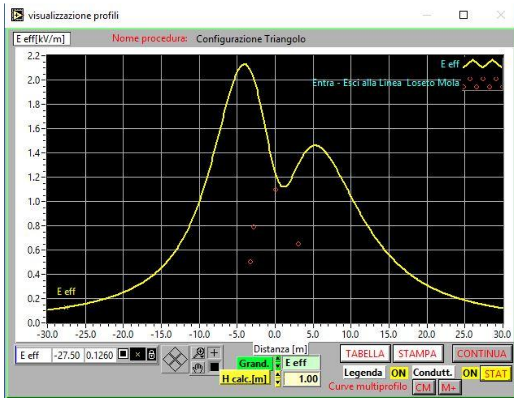
Figura 3 : Valutazione del Campo Elettrico ad 1 m dal suolo, Configurazione a Triangolo
