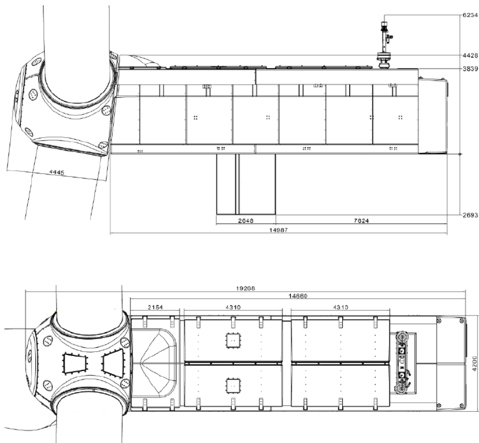
Figura 1- Schema aerogeneratore
