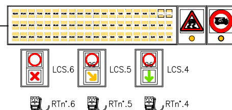
PANNELLO MESSAGGIO VARIABILE N° PMV03-A14S TANGENZIALE - MI DIREZIONE NORD
