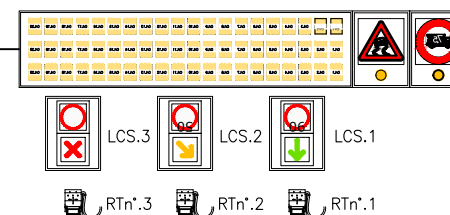
PANNELLO MESSAGGIO VARIABILE N° PMV11-TNG TANGENZIALE - MI
