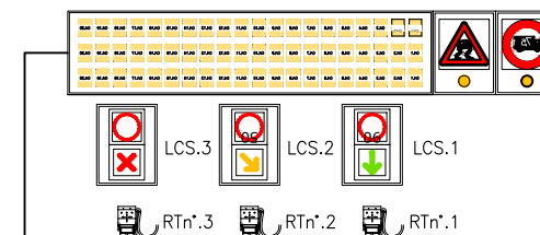
PANNELLO MESSAGGIO VARIABILE N° PMV08-TGS TANGENZIALE - TA
