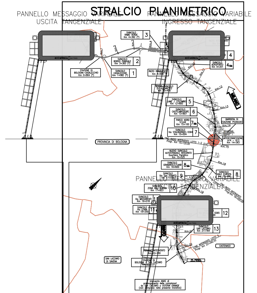
PANNELLO MESSAGGIO VARIABILE INGRESSO TANGENZIALE
