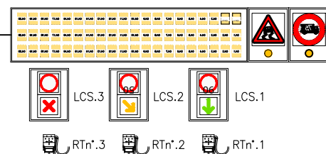
PANNELLO MESSAGGIO VARIABILE N°PMV02-TNG TANGENZIALE - MI
