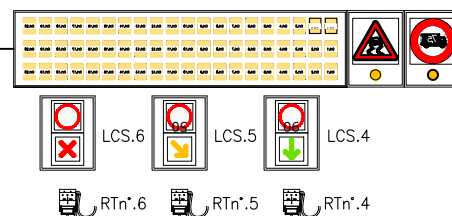
PANNELLO MESSAGGIO VARIABILE N° PMV10-TGS TANGENZIALE - TA DIREZIONE SUD
