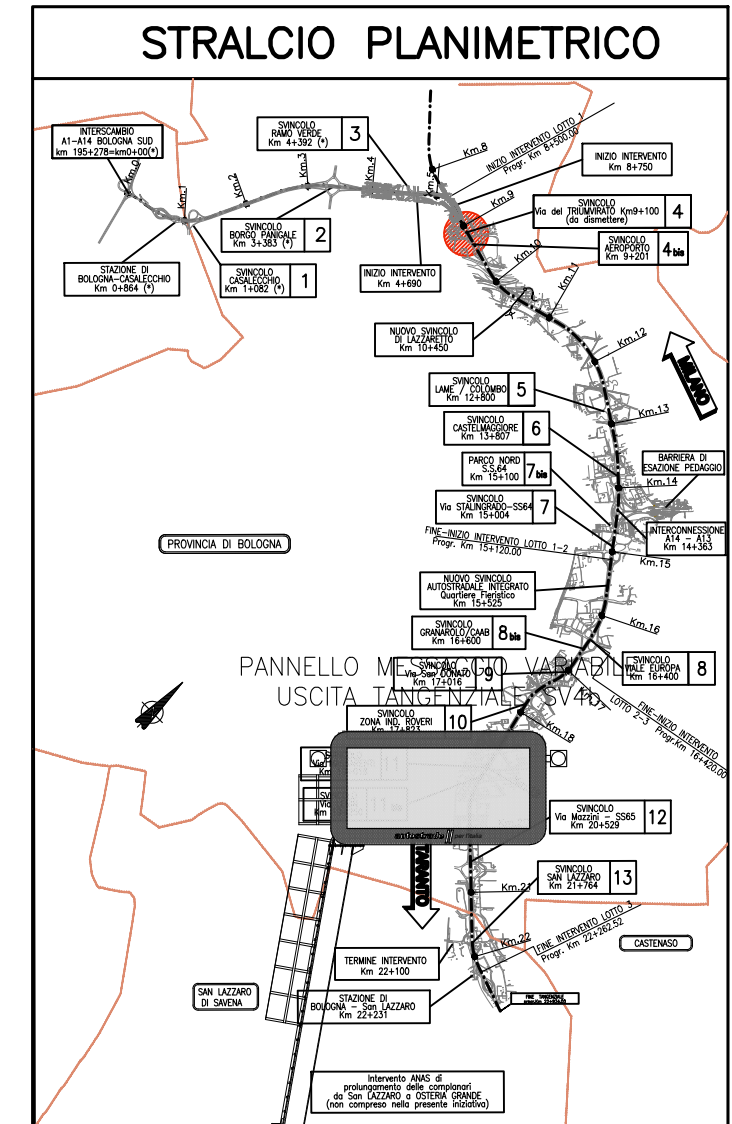
PANNELLO MESSAGGIO VARIABILE USCITA TANGENZIALE SV4b
