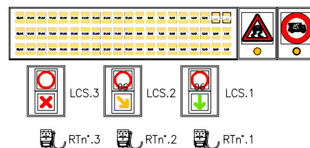
PANNELLO MESSAGGIO VARIABILE N° PMV10-TGS AUTOSTRADA - TA DIREZIONE SUD
