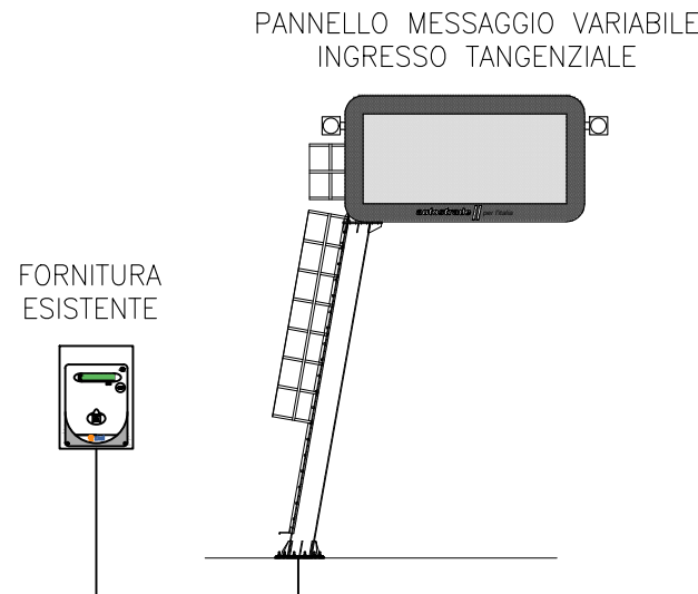
PANNELLO MESSAGGIO VARIABILE N° PMV11-TNG TANGENZIALE - MI
