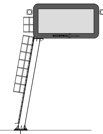
PANNELLO MESSAGGIO VARIABILE INGRESSO TANGENZIALE
