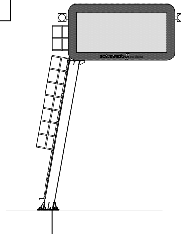
PANNELLO MESSAGGIO VARIABILE INGRESSO TANGENZIALE
