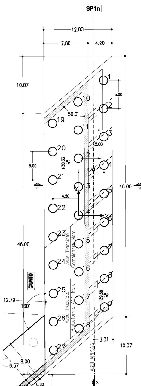
Figura 6 – Schema palificata spalla SP1 Nord
