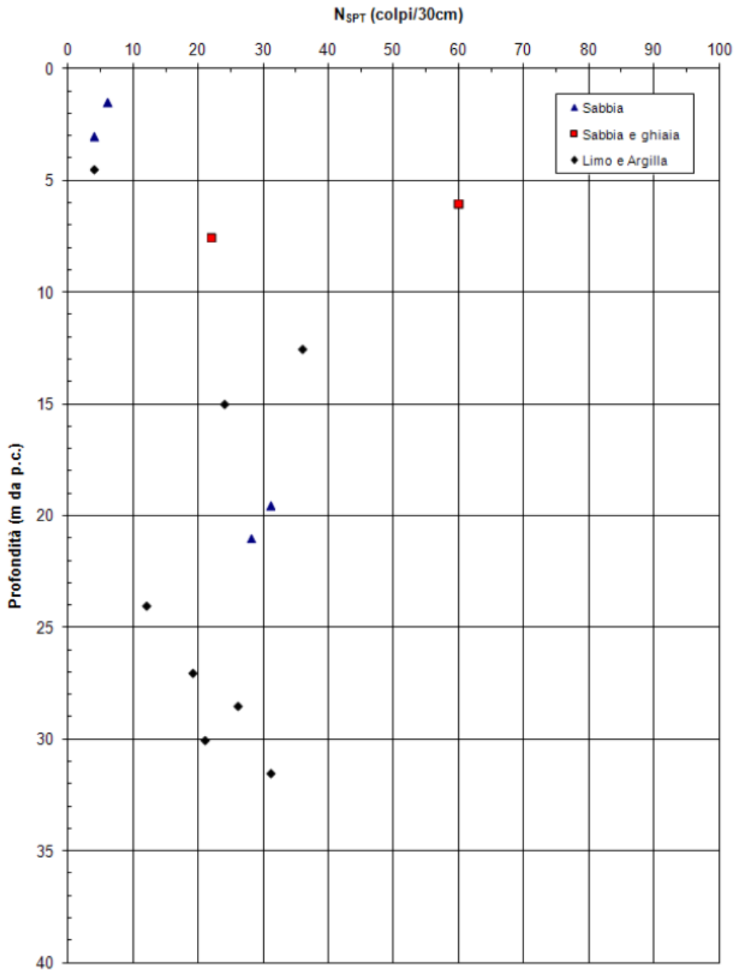
Figura 2 – N_{spt} (PB29)
