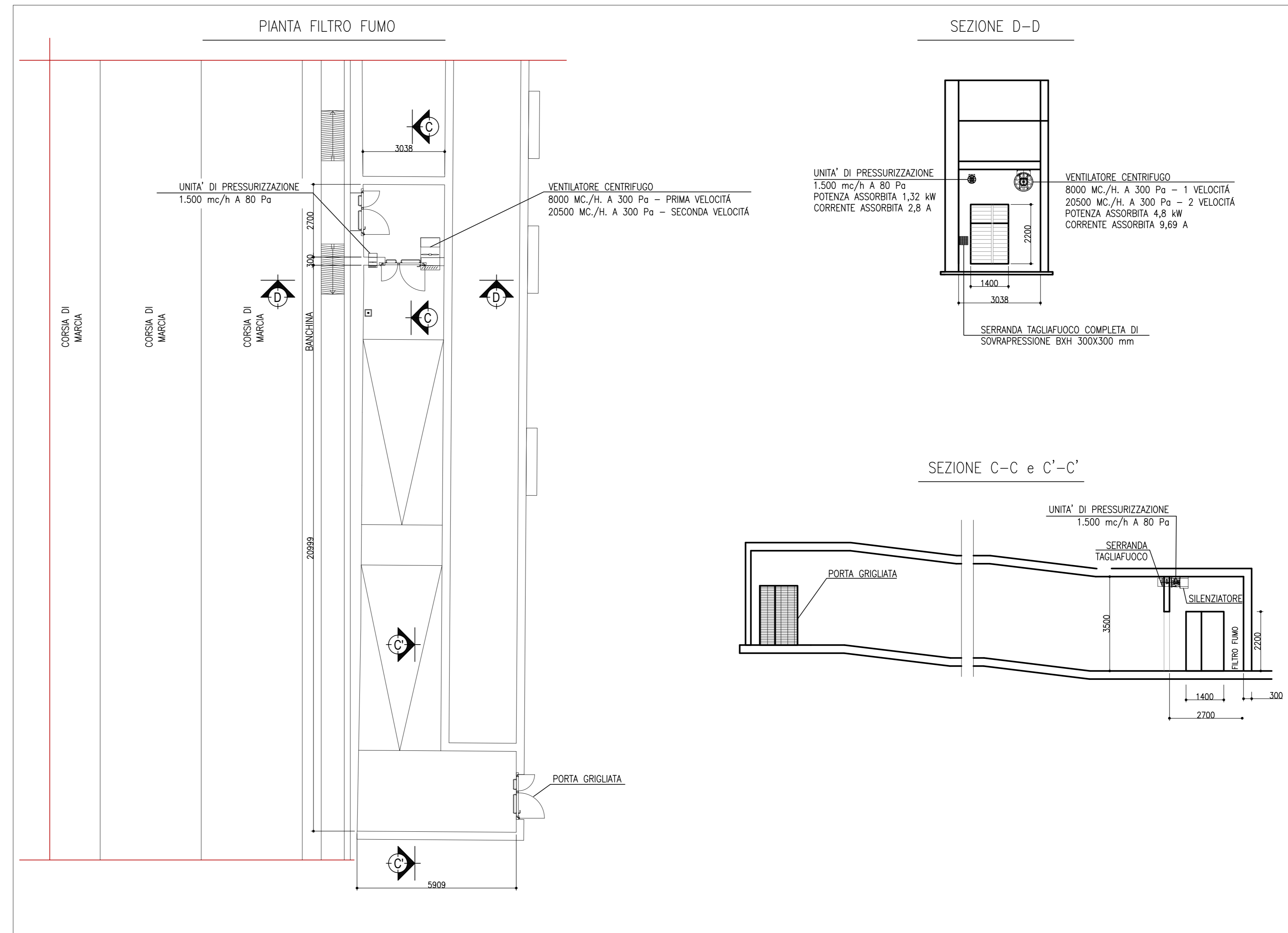
USCITA DI SICUREZZA – SCALA "3" PIANTA E SEZIONE SCALA 1:100
