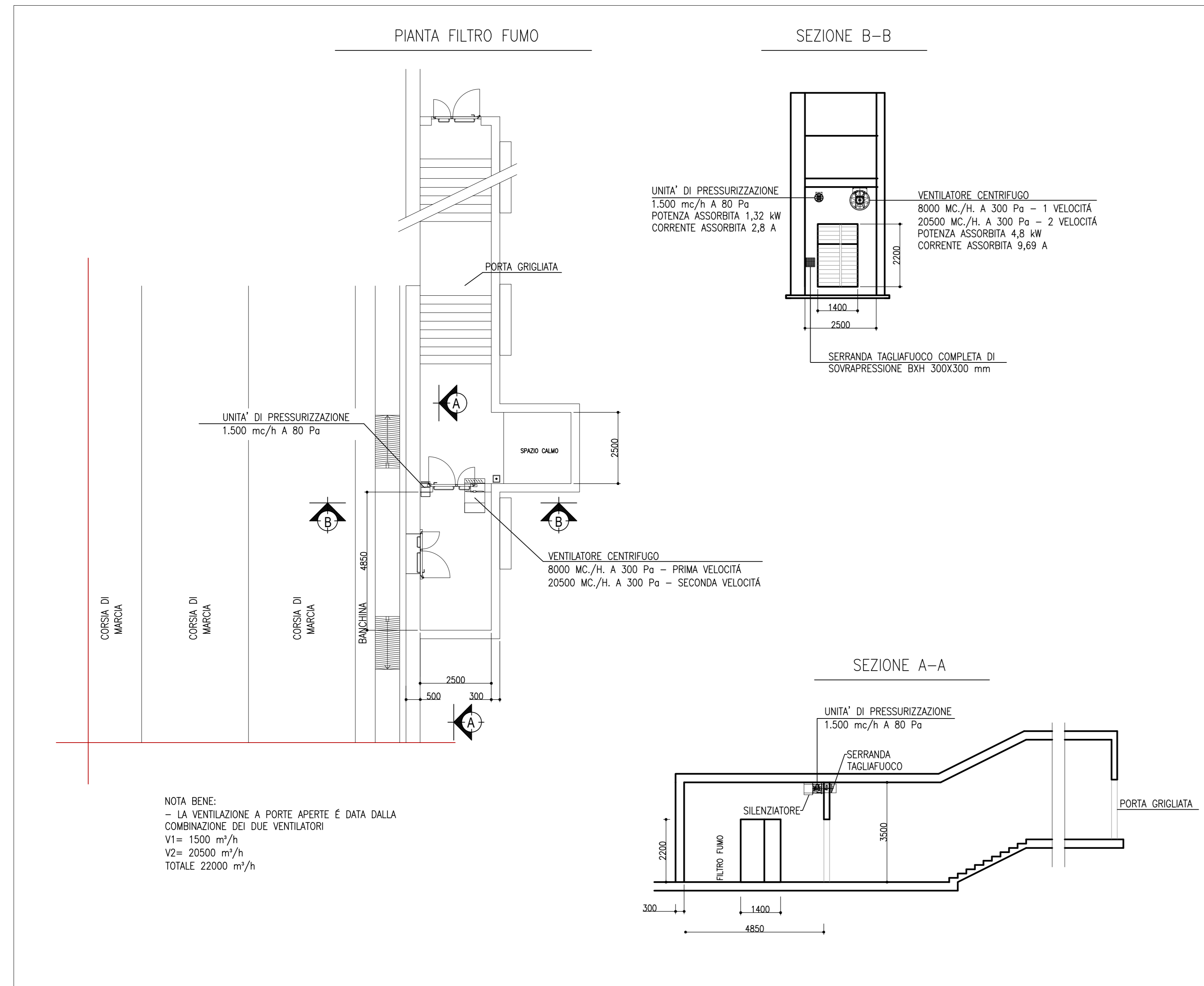
USCITA DI SICUREZZA – SCALA "2" PIANTA E SEZIONE SCALA 1:100
