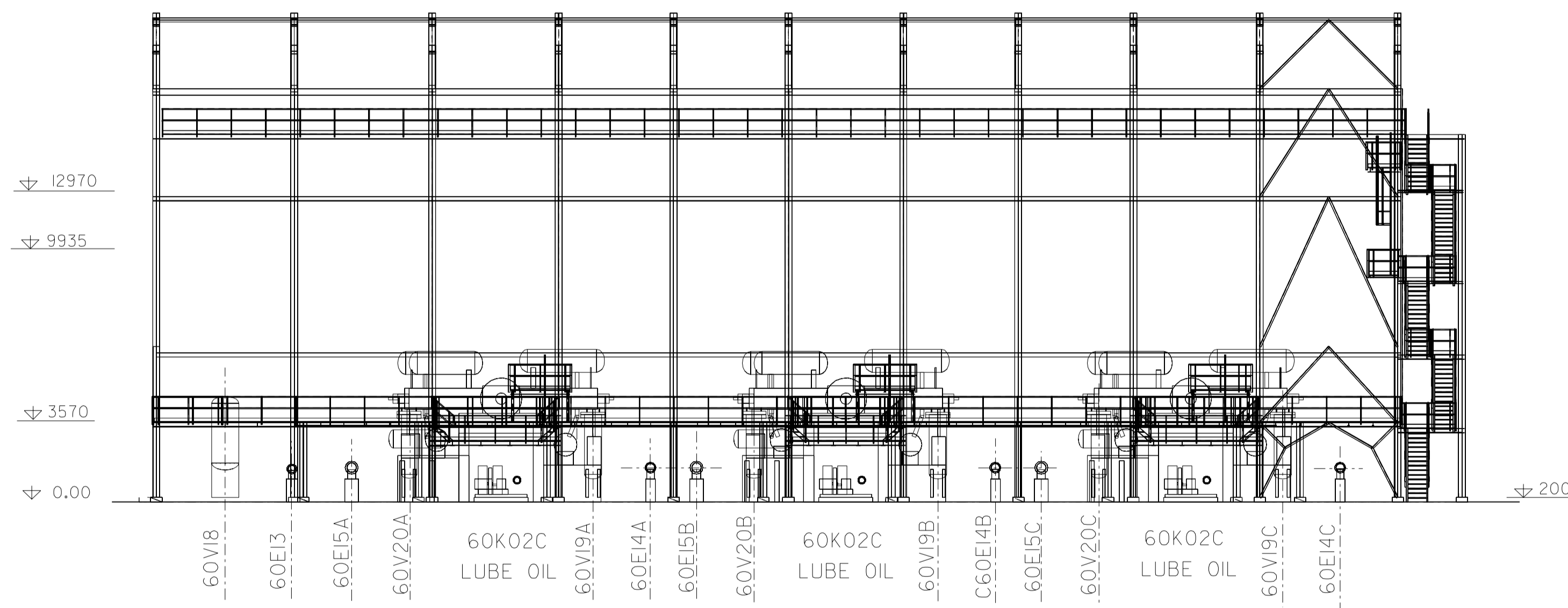
SEZIONE K-K
