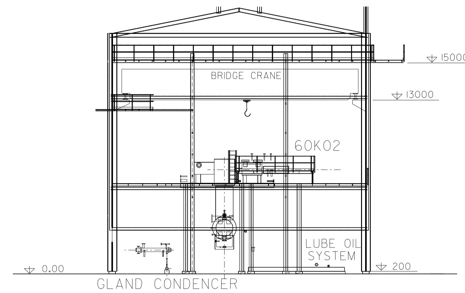
SEZIONE J-J
