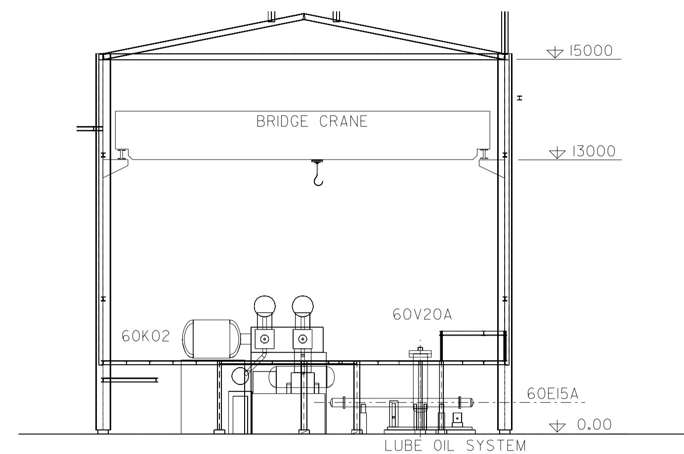
SEZIONE I-I
