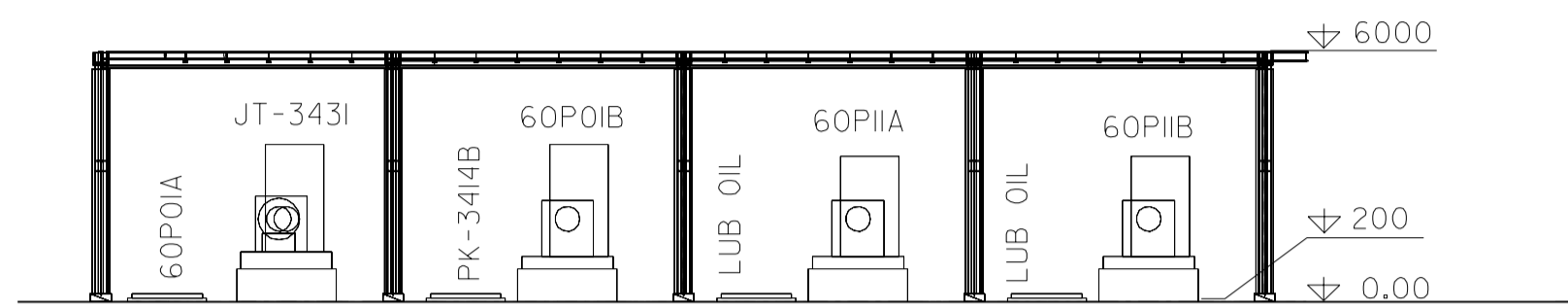
SEZIONE H-H
