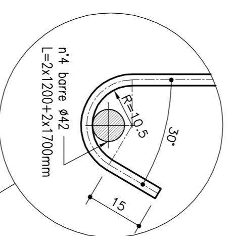
SEZIONE A-A
