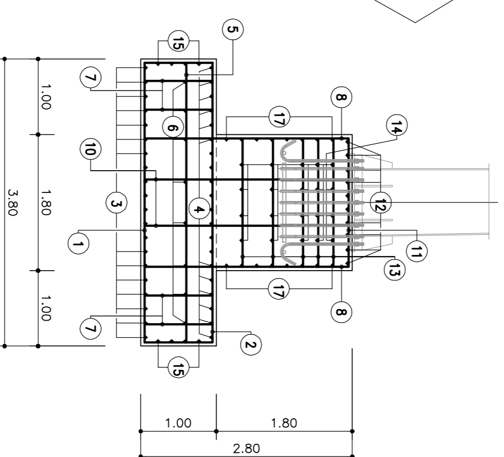
SEZIONE A-A
