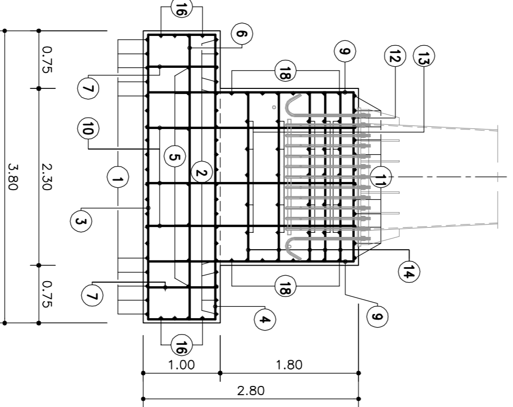
SEZIONE B-B
