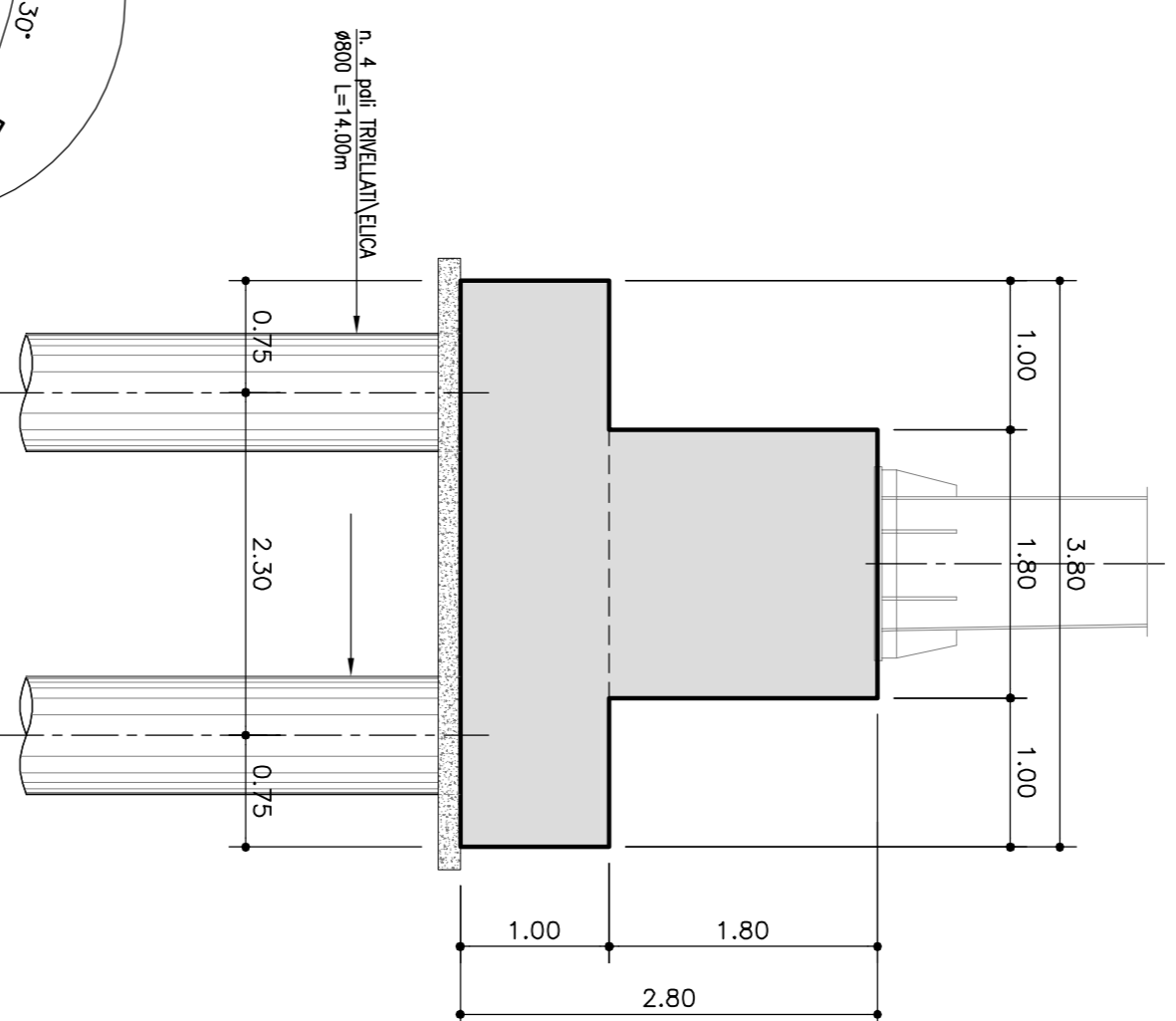
SEZIONE A-A
