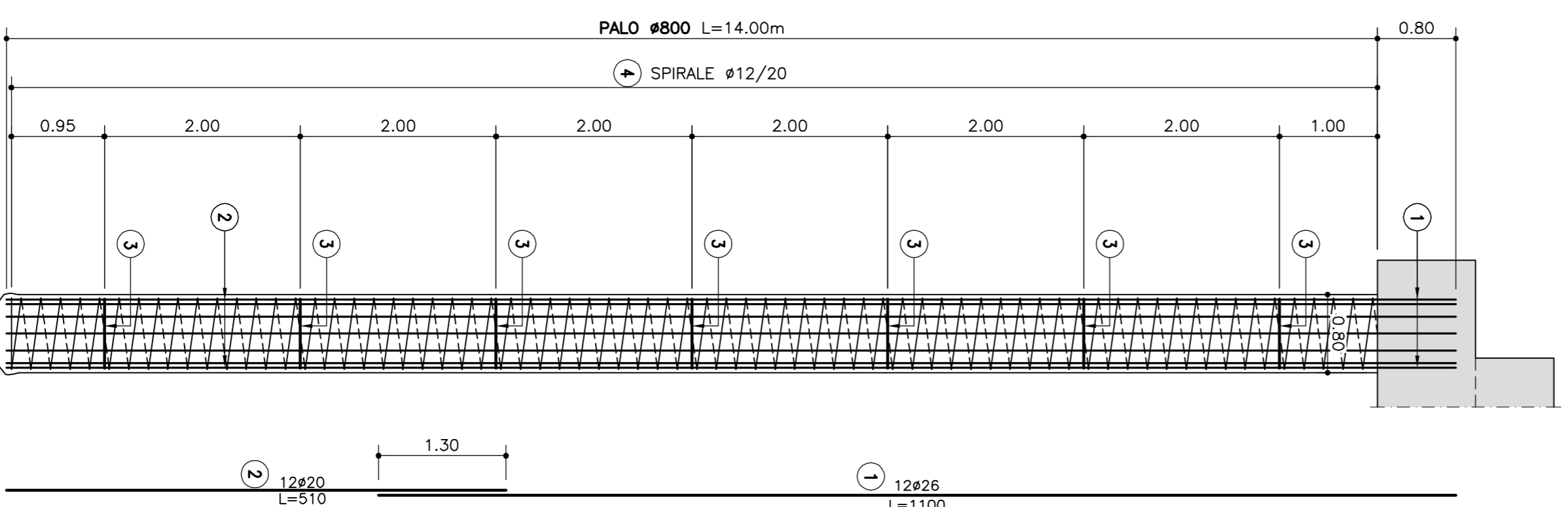
SEZIONE A-A
