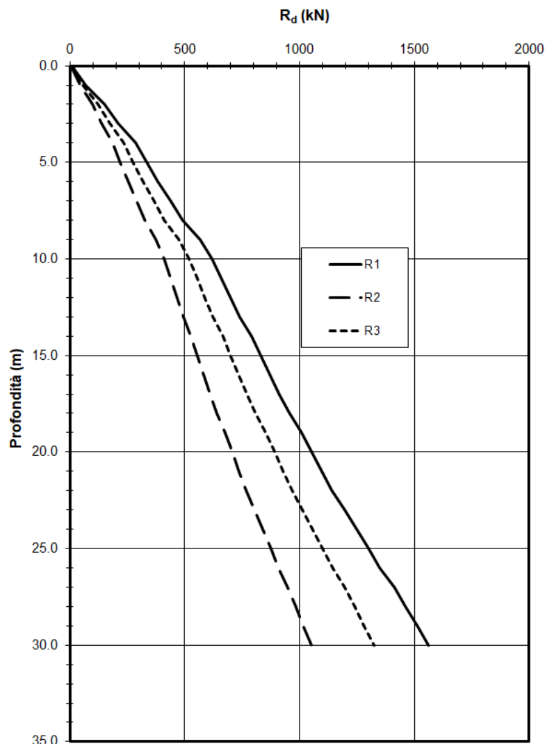
Figura 8-1: Resistenza del palo f 600 a compressione
