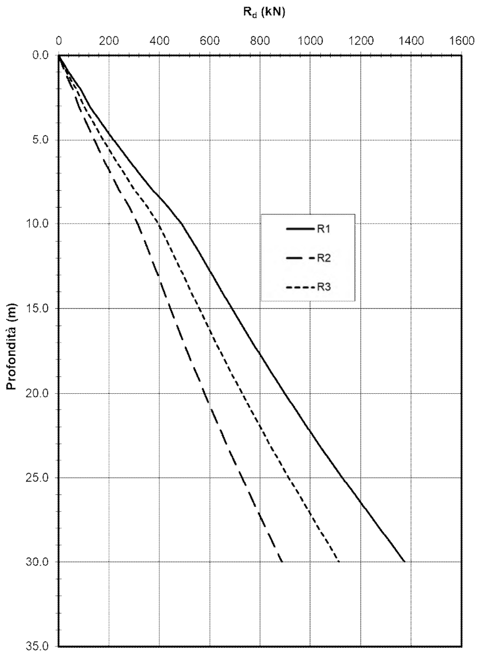
Figura 8-2: Resistenza del palo f 600 a trazione
