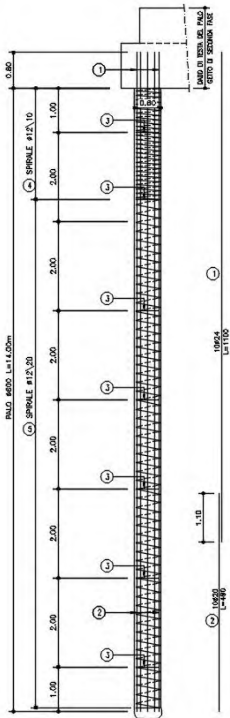
Figura 6-2: Armatura palo di fondazione
