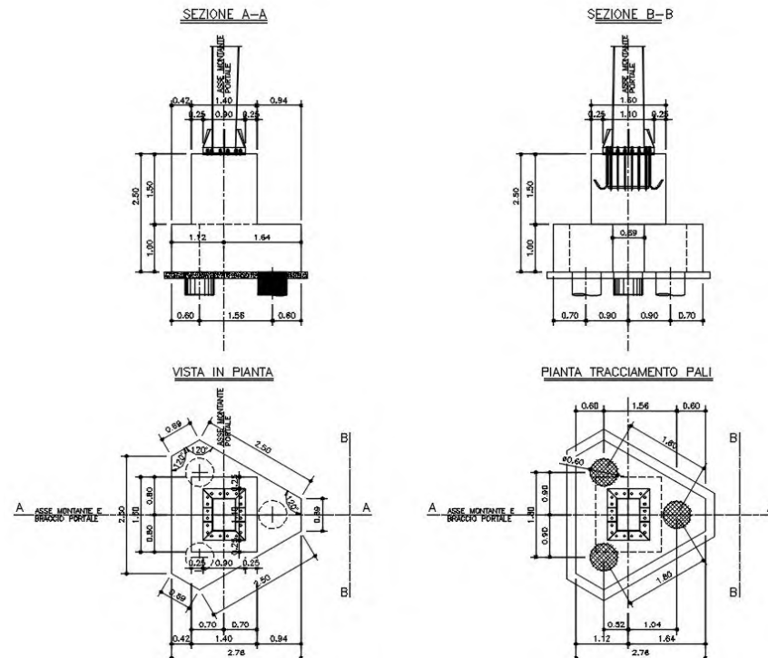
Figura 6-1: Carpenteria plinto di fondazione
