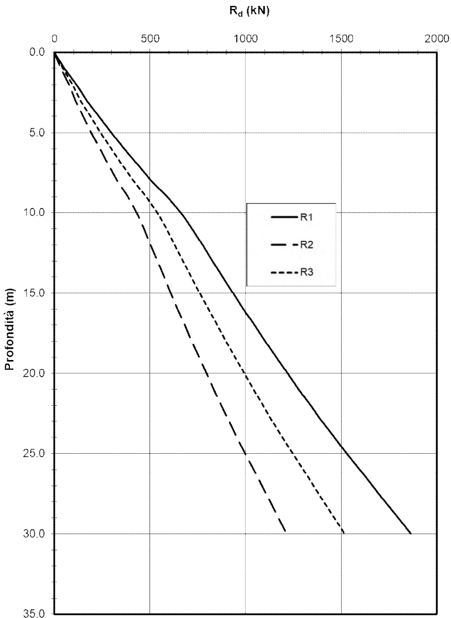
Figura 8-2: Resistenza del palo f 800 a trazione
