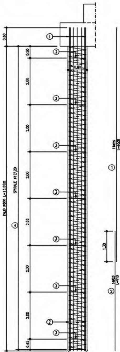
Figura 6-2: Armatura palo di fondazione
