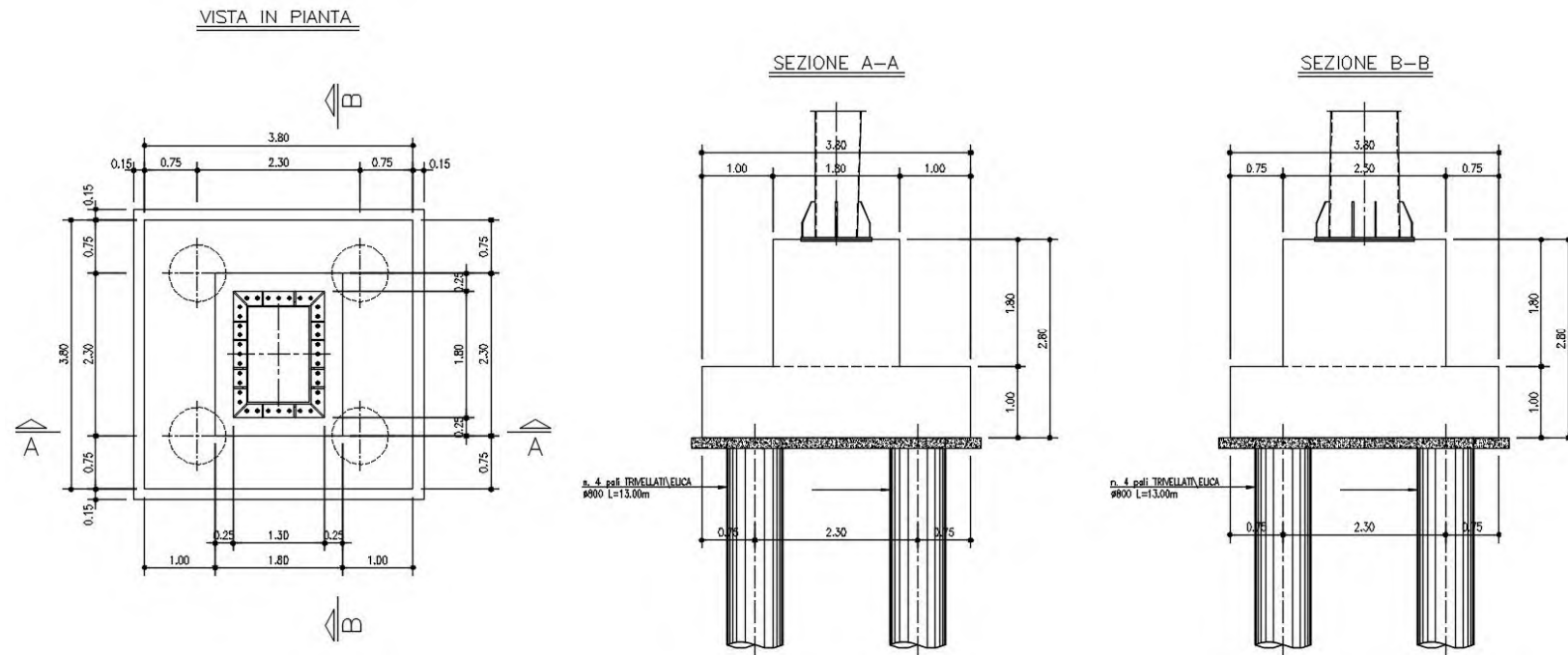
Figura 6-1: Carpenteria plinto di fondazione
