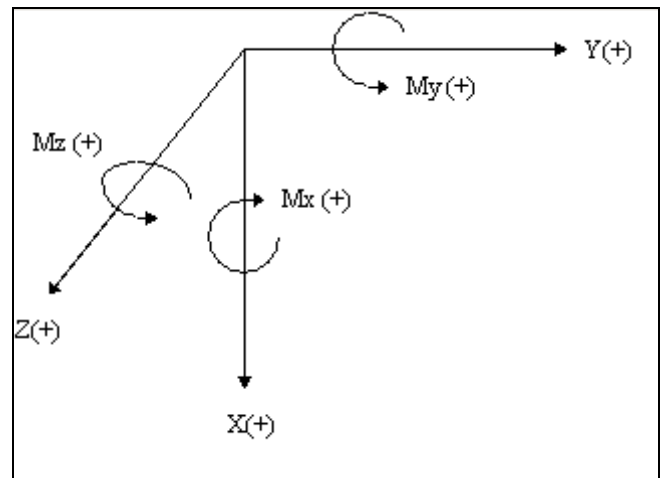
Figura 7-2: Convenzioni di segno del programma di calcolo GROUP
