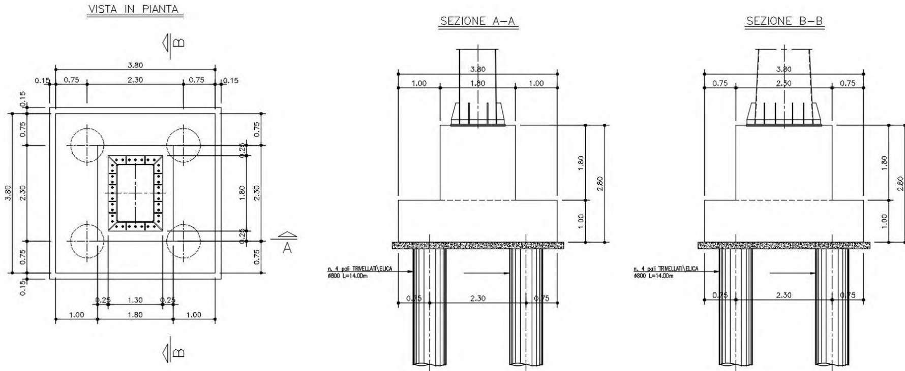
Figura 6-1: Carpenteria plinto di fondazione
