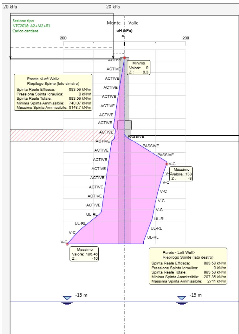
Figura 12-1. Riepilogo spinte fase 4 (sovraccarico cantiere) – combinazione A2+M2+R1
