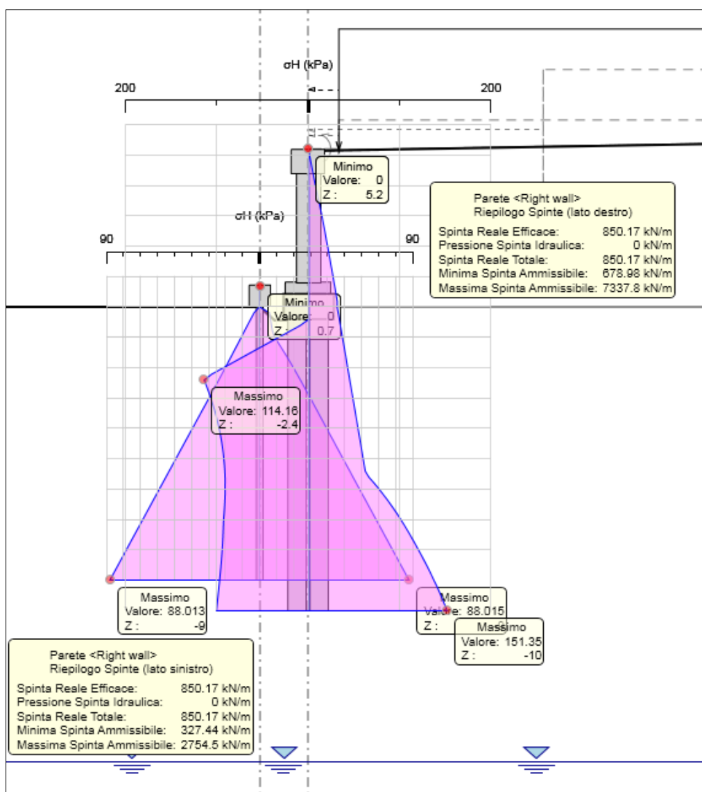
Figura 9-1. Riepilogo spinte fase 5 (traffico su ampliamento) – combinazione A2+M2+R1
