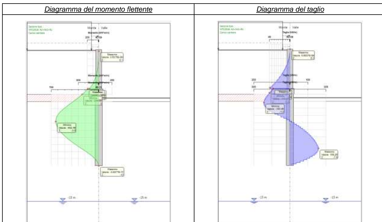
Figura 11-4. Sollecitazioni nelle strutture nella combinazione SLU A2+M2+R1 in presenza di sovraccarico
