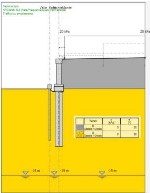
Figura 7-4 Carico esterno agente in presenza di traffico
