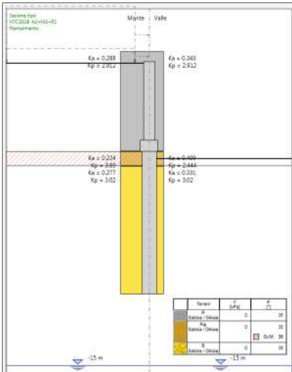
Figura 10-3 Coefficienti di spinta nella combinazione SLU-GEO
