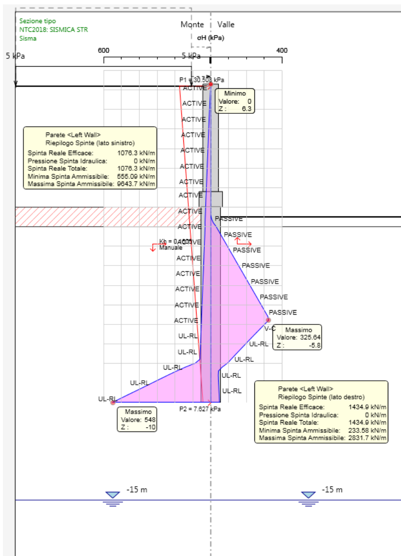
Figura 12-2. Riepilogo spinte fase 5(sisma) – combinazione SLV
