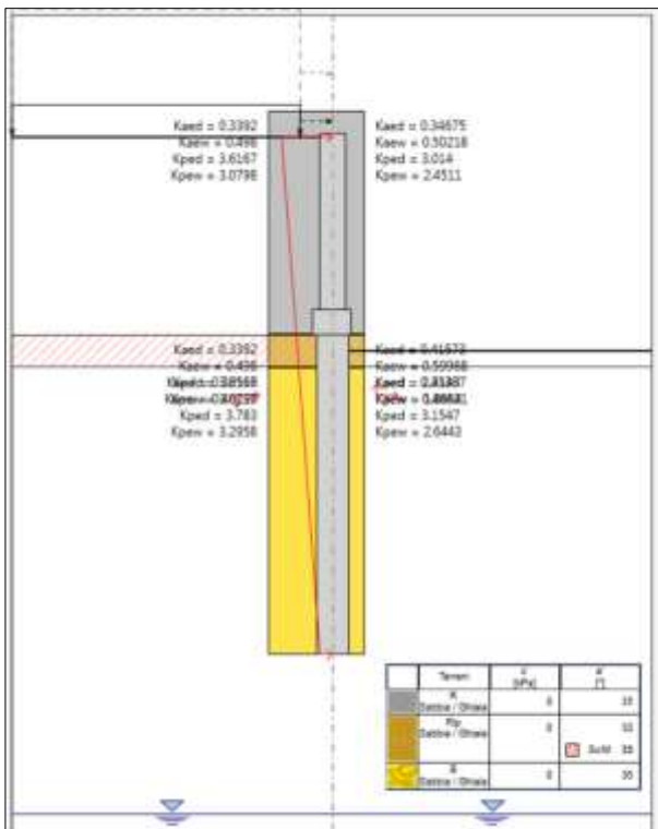
Figura 10-4 Coefficienti di spinta nella combinazione SLV
