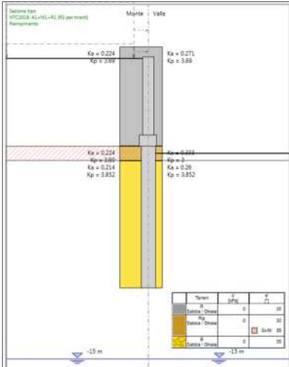
Figura 10-2. Coefficienti di spinta nelle combinazioni SLE e SLU-STR
