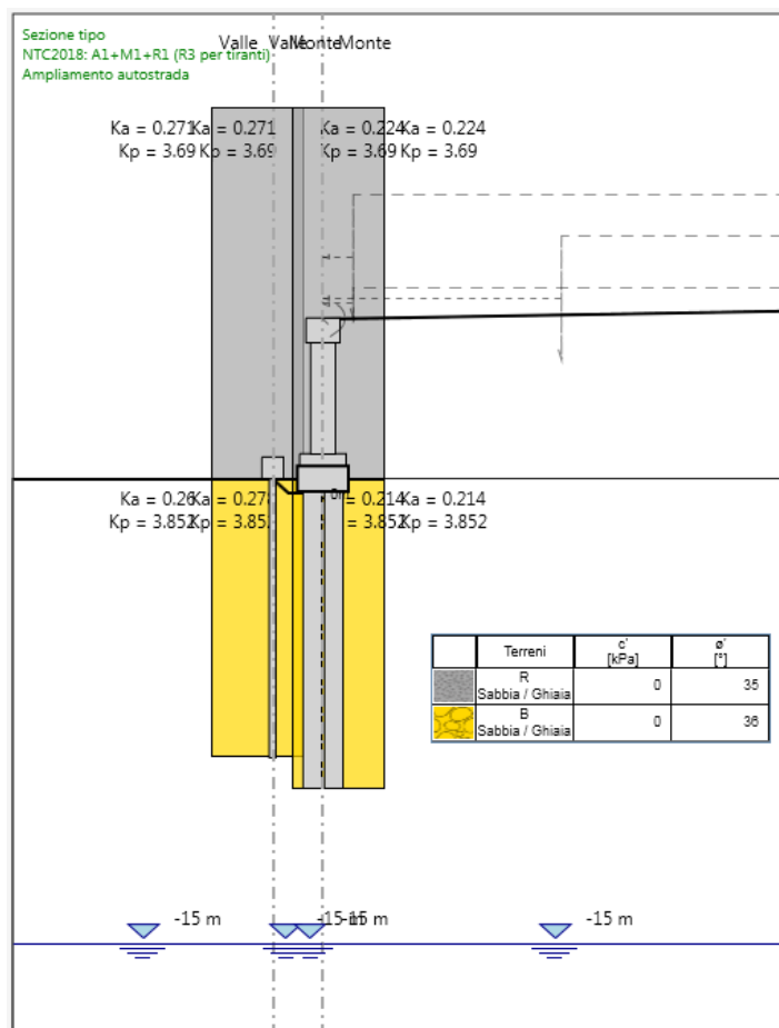
Figura 7-1. Coefficienti di spinta nelle combinazioni SLE e SLU-STR
