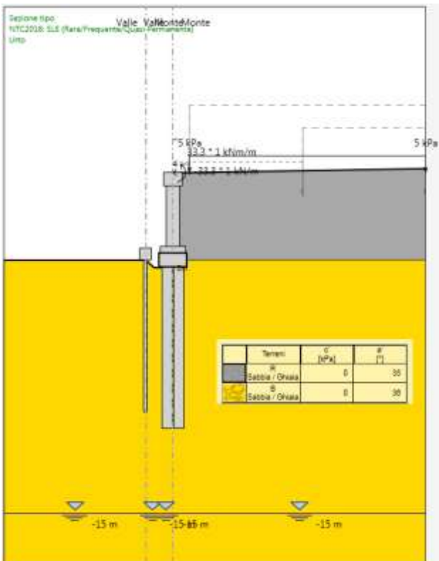
Figura 7-5 Carichi esterni agenti in condizioni eccezionali (urto)
