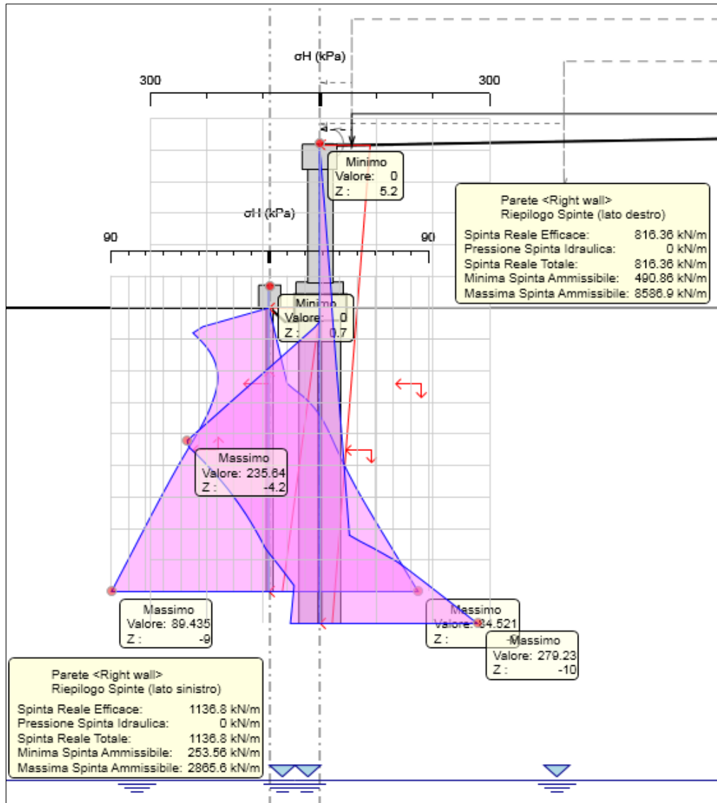
Figura 9-2. Riepilogo spinte fase 7 (sisma) – combinazione SLV
