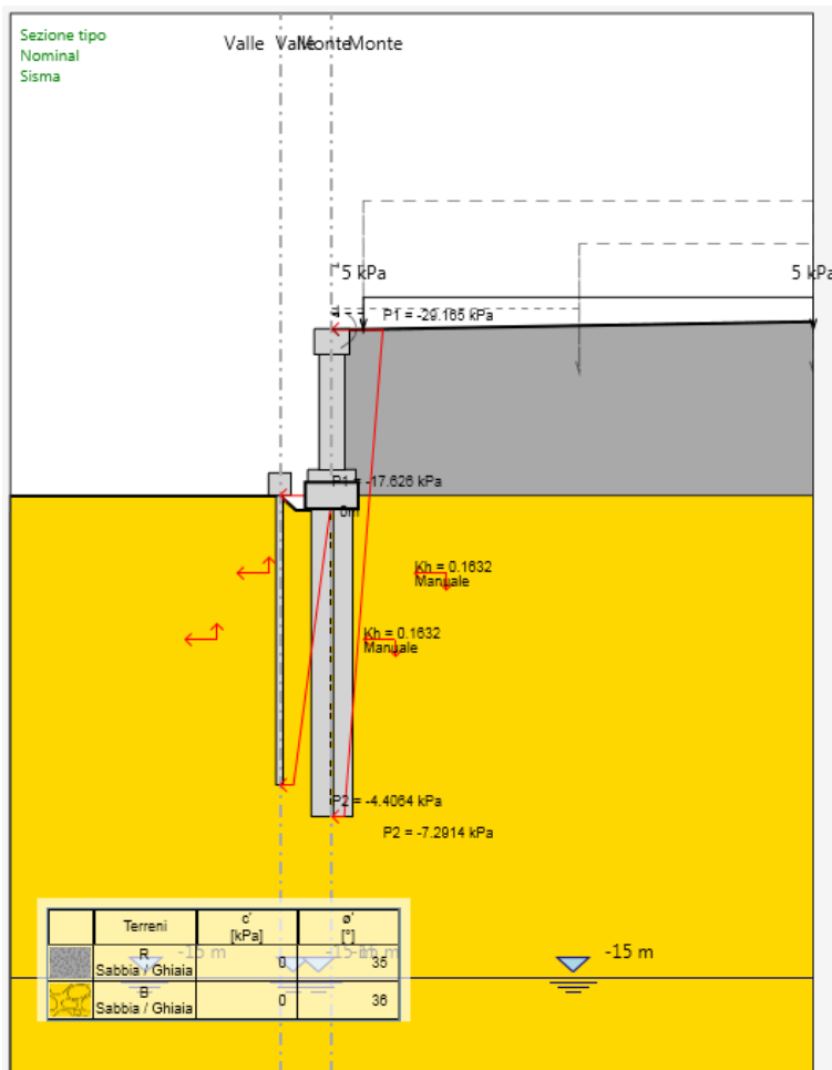
Figura 7-7. Diagramma di carico applicato al muro in condizioni sismiche
