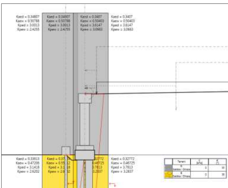
Figura 7-3 Coefficienti di spinta nella combinazione SLV
