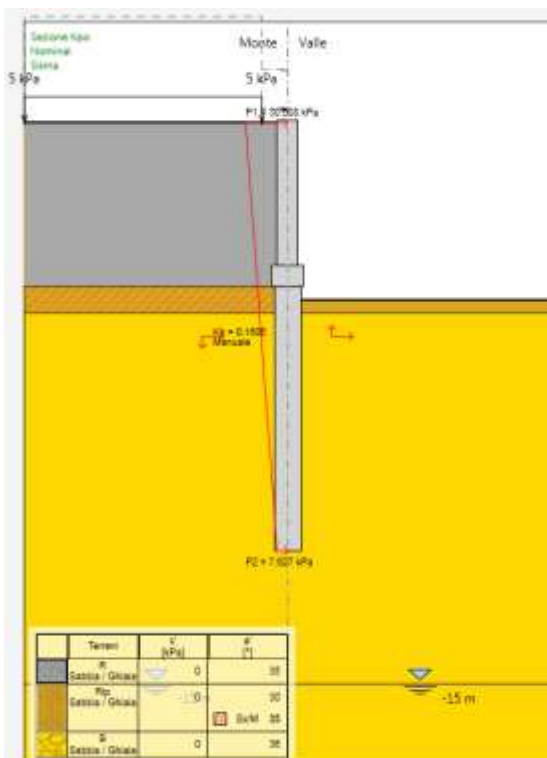
Figura 10-7. Diagramma di carico applicato al muro in condizioni sismiche
