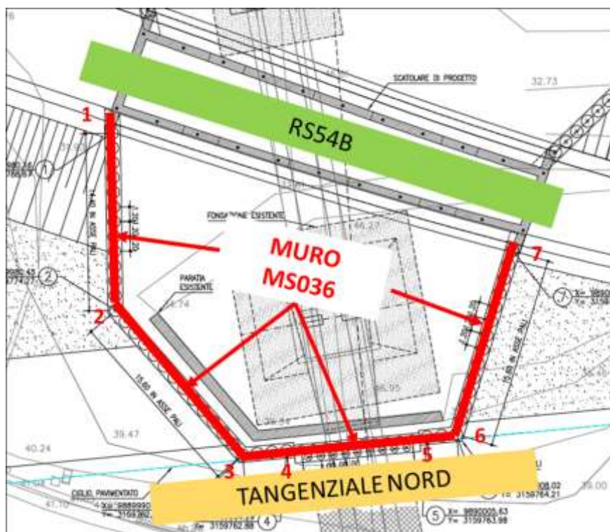
Figura 1-1. Schema Pianta Muro MS036
