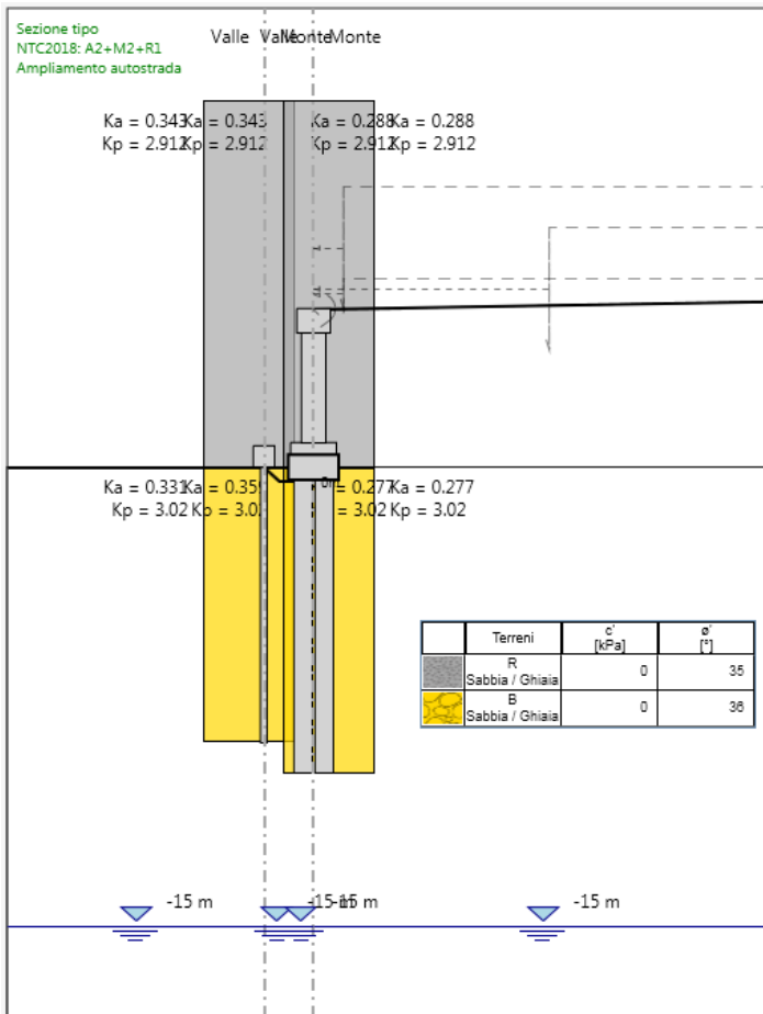
Figura 7-2 Coefficienti di spinta nella combinazione SLU-GEO
