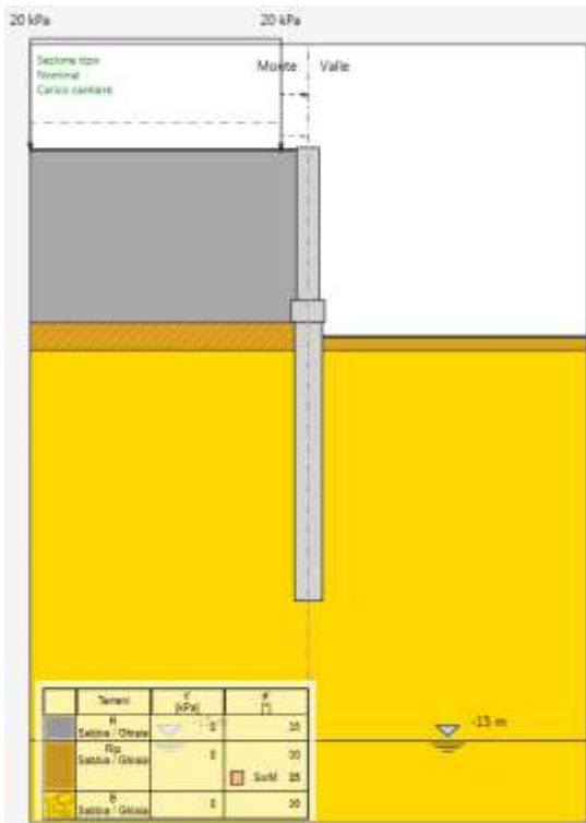
Figura 10-5 Carico esterno agente in presenza di traffico
