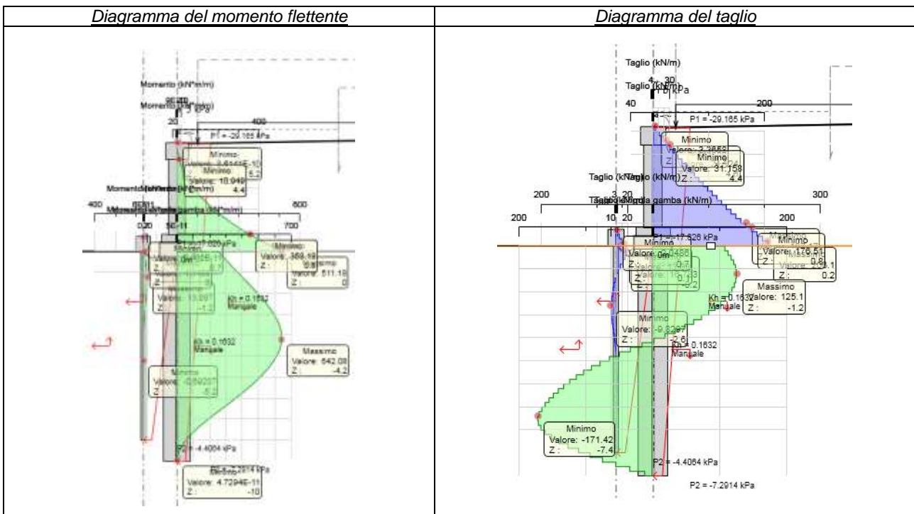
Figura 8-4. Sollecitazioni nelle strutture nella combinazione SLV (sisma)
