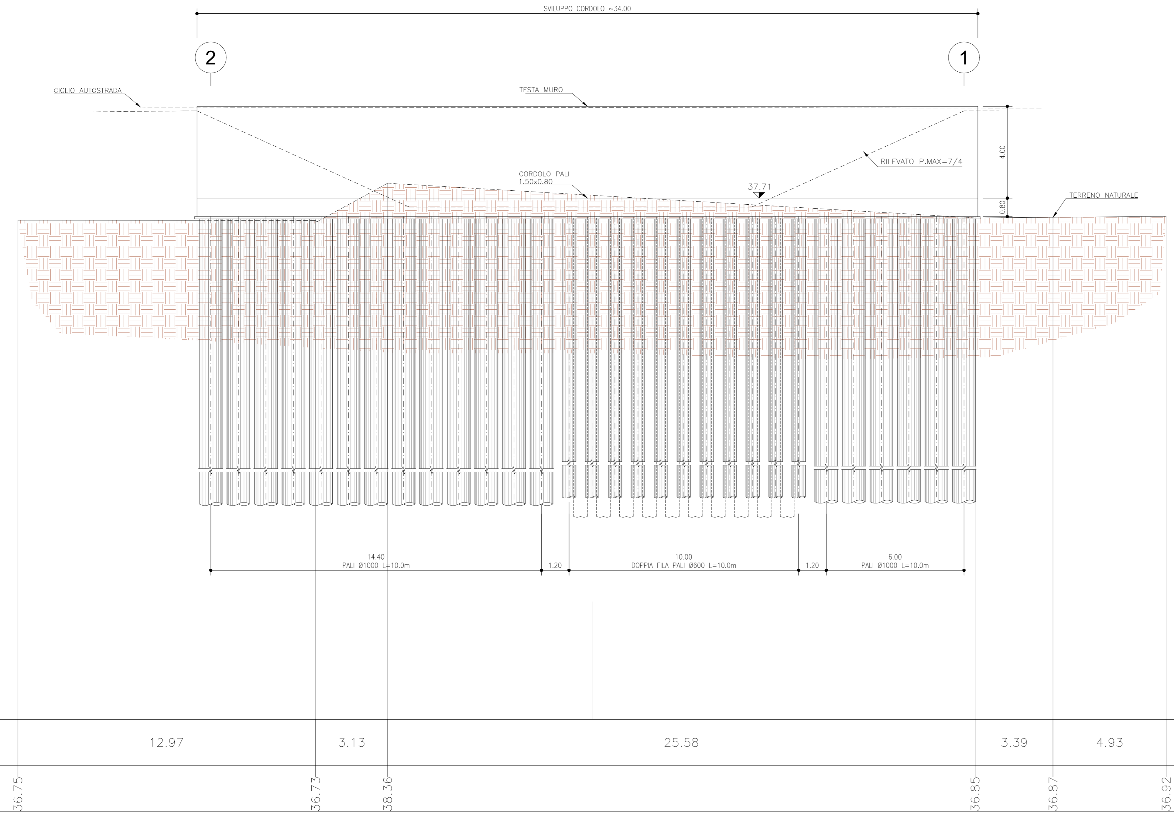
SVILUPPATA PARATIA DI PALI MS 038 1:100
