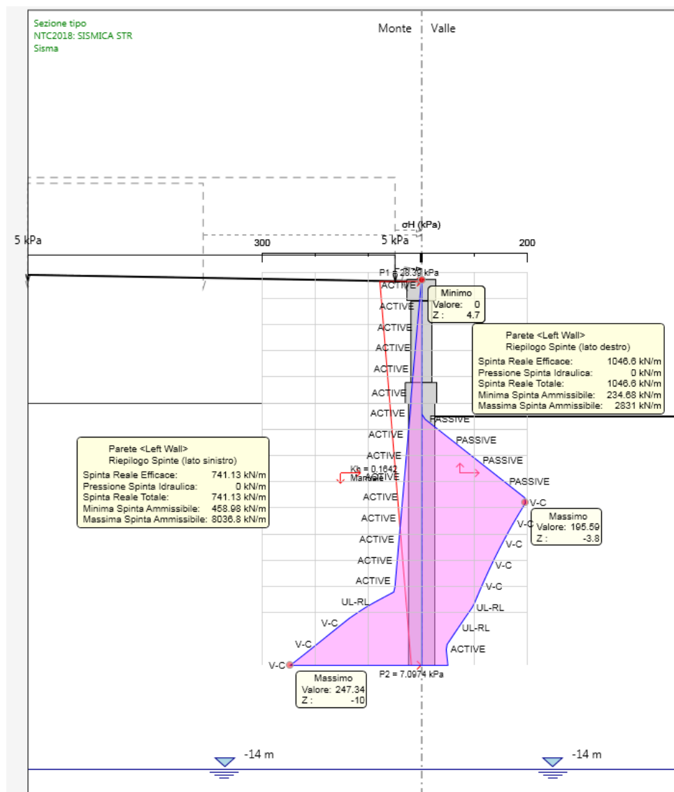
Figura 12-2. Riepilogo spinte fase 7 (sisma) – combinazione SLV
