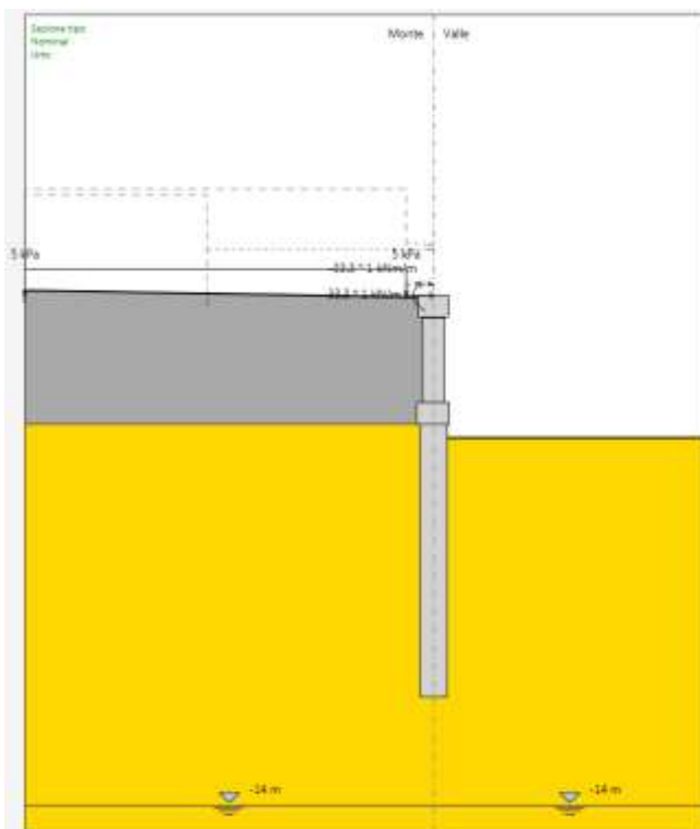
Figura 10-6 Carichi esterni agenti in caso di urto
