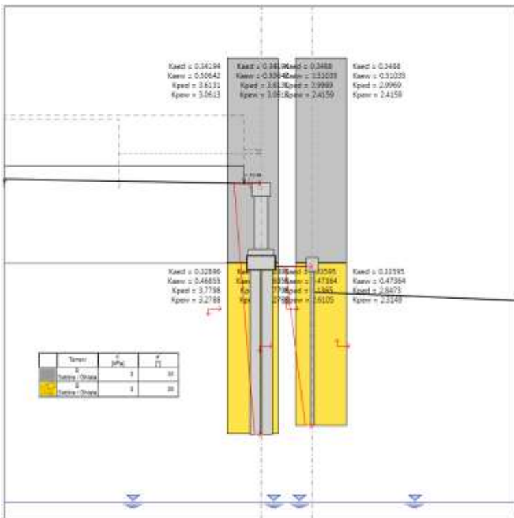
Figura 7-3 Coefficienti di spinta nella combinazione SLV
