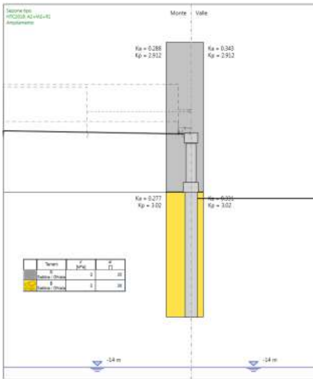
Figura 10-3 Coefficienti di spinta nella combinazione SLU-GEO
