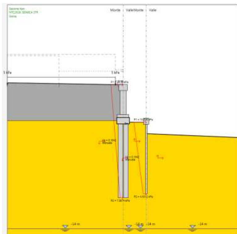
Figura 7-7. Diagramma di carico applicato al muro in condizioni sismiche
