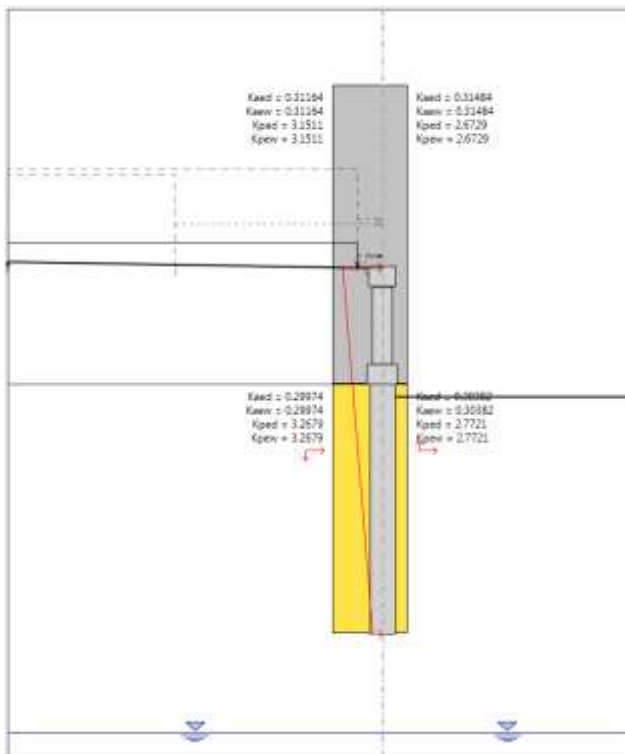
Figura 10-4 Coefficienti di spinta nella combinazione SLV
