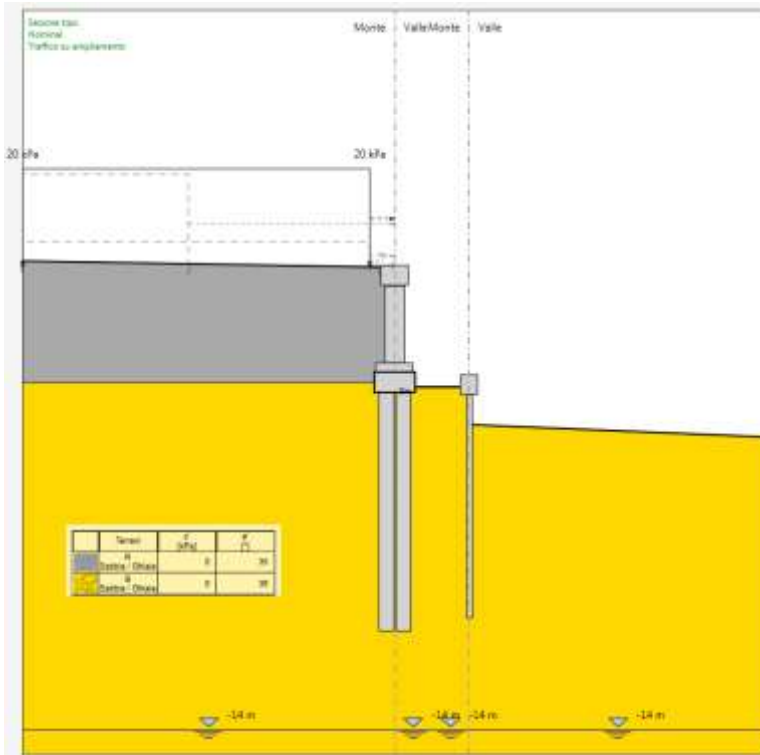
Figura 7-4 Carico esterno agente in presenza di traffico
