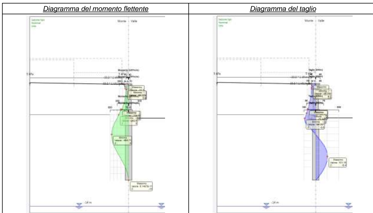
Figura 11-3. Sollecitazioni nelle strutture nella combinazione ECC
