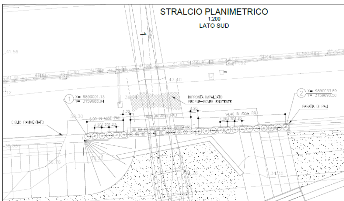
Figura 1-1. Pianta Muro MS038
