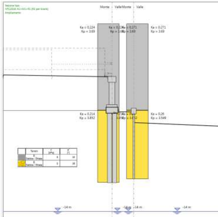
Figura 7-1. Coefficienti di spinta nelle combinazioni SLE e SLU-STR
