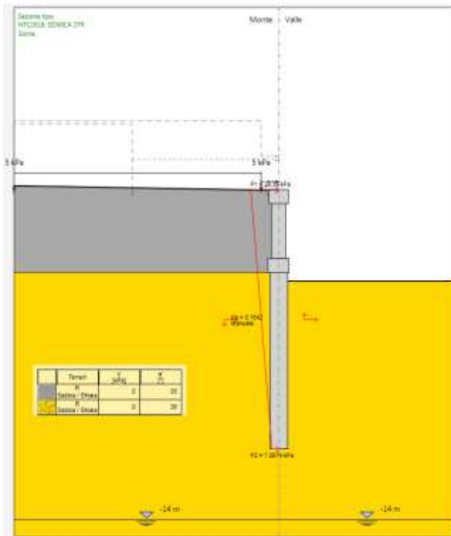
Figura 10-8. Diagramma di carico applicato al muro in condizioni sismiche
