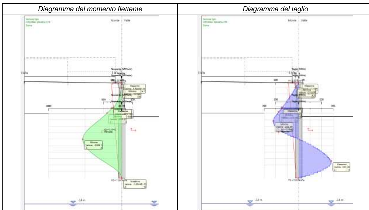
Figura 11-4. Sollecitazioni nelle strutture nella combinazione SLV (sisma)
