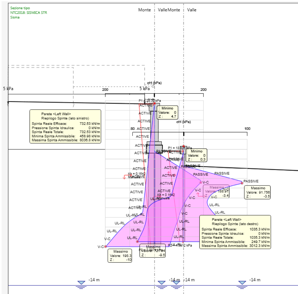
Figura 9-2. Riepilogo spinte fase 7 (sisma) – combinazione SLV
