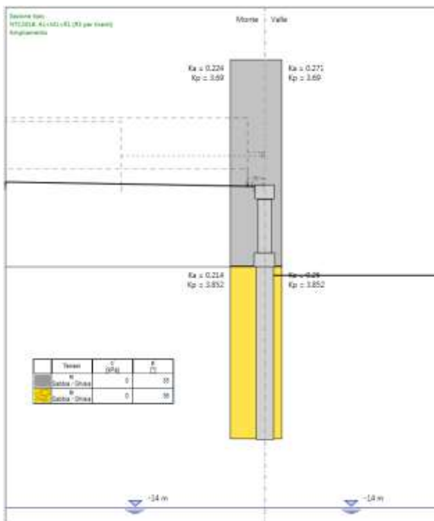
Figura 10-2. Coefficienti di spinta nelle combinazioni SLE e SLU-STR
