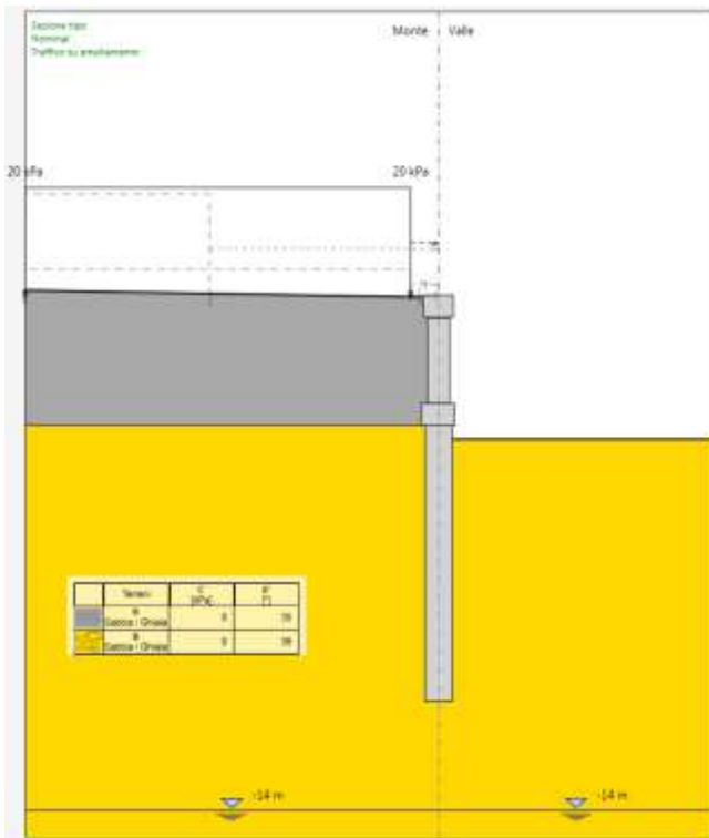
Figura 10-5 Carico esterno agente in presenza di traffico
