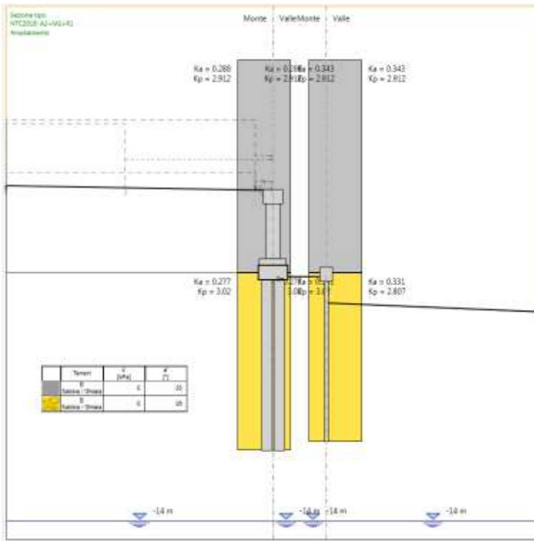
Figura 7-2 Coefficienti di spinta nella combinazione SLU-GEO
