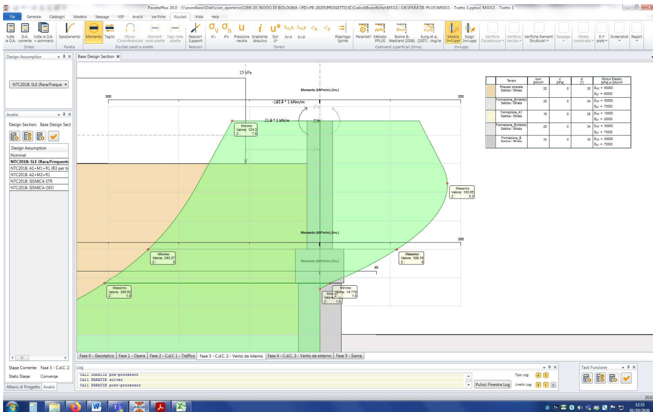
Figura n.10.14 – Momento flettente - Inviluppo SLE-QP
