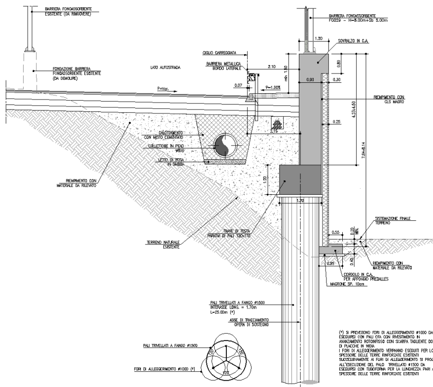
Figura 1-2. Sezione tipo opera di sostegno MS011 – Tratto con pali eseguiti da rilevato provvisorio
