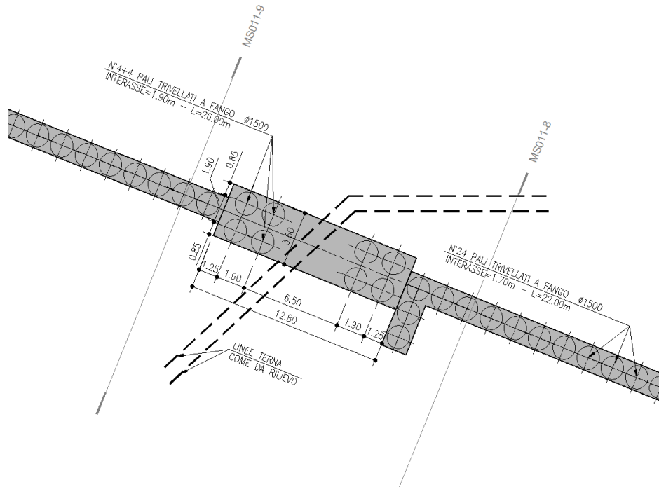
Figura 1-3 – Opera di scavalco linea TERNA esistente - Pianta
