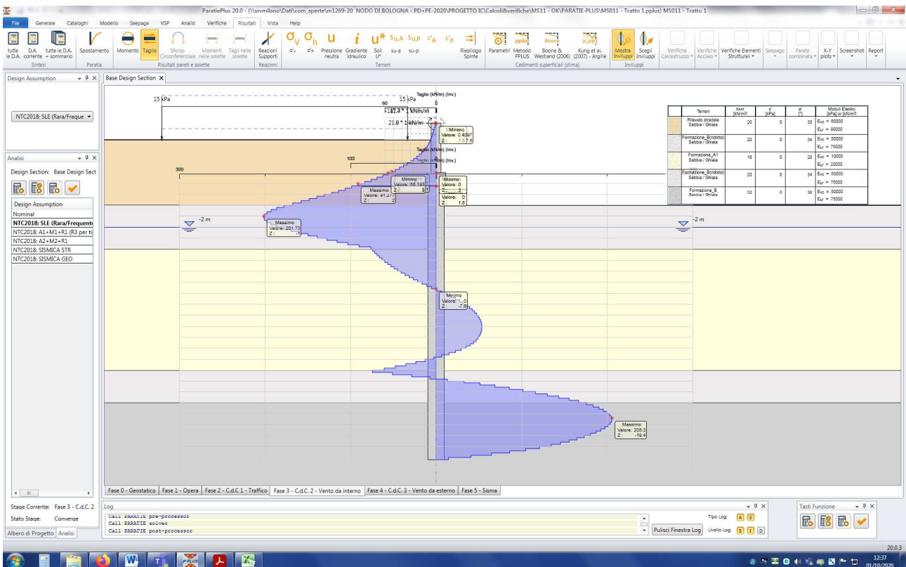
Figura n. 10.13 – Azione di taglio - Inviluppo SLV
