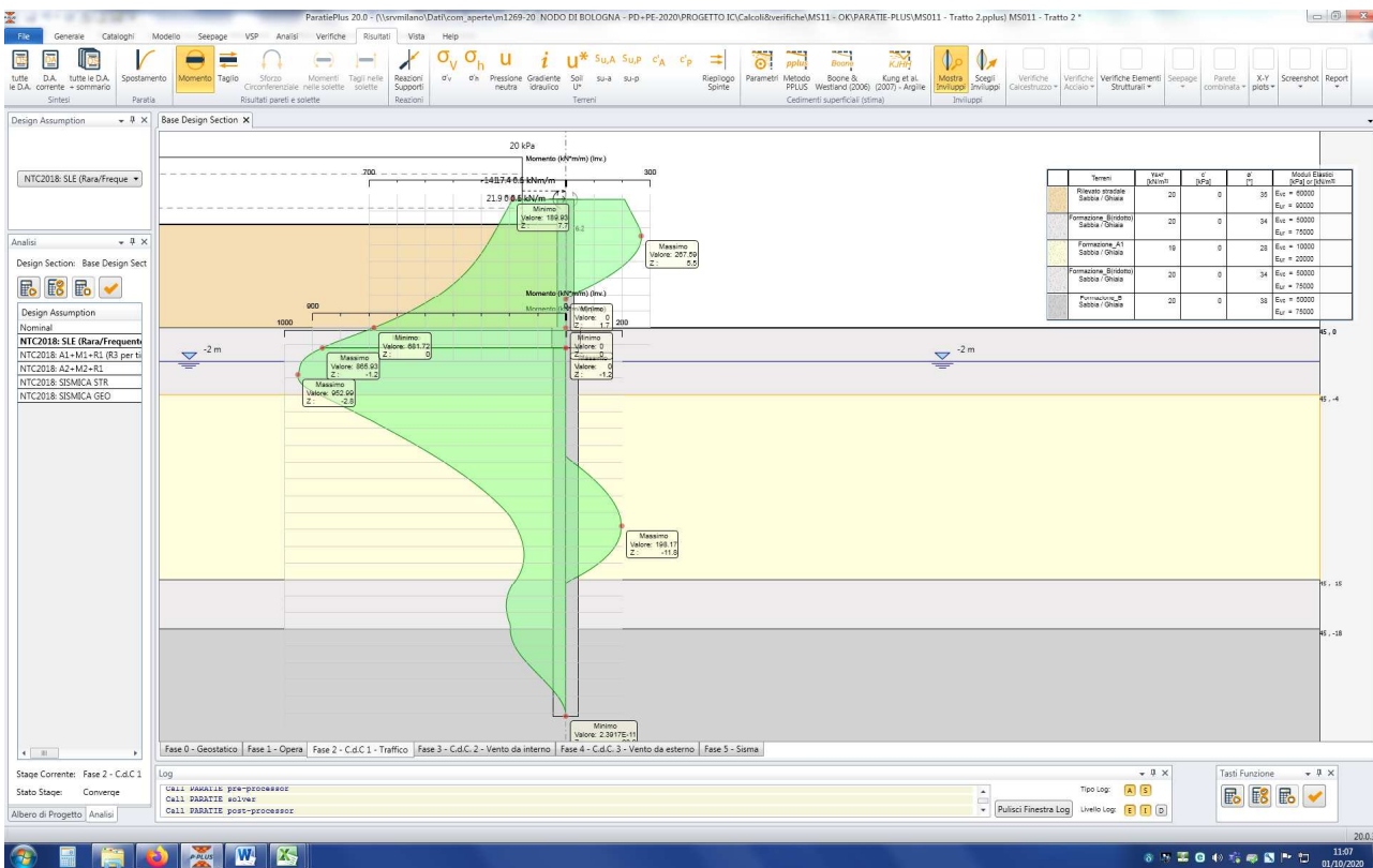
Figura n.8.10 – Momento flettente - Involuppo SLU
