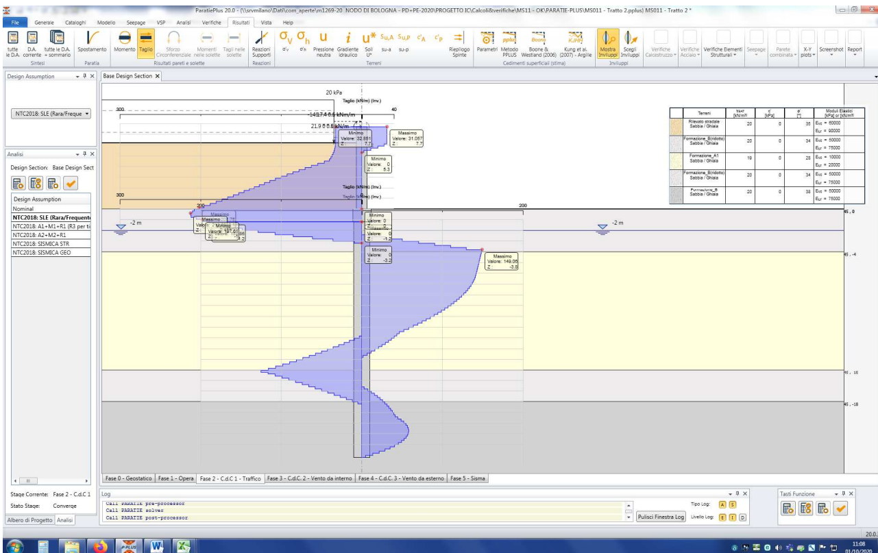
Figura n.8.11 – Azione di taglio - Involuppo SLU
