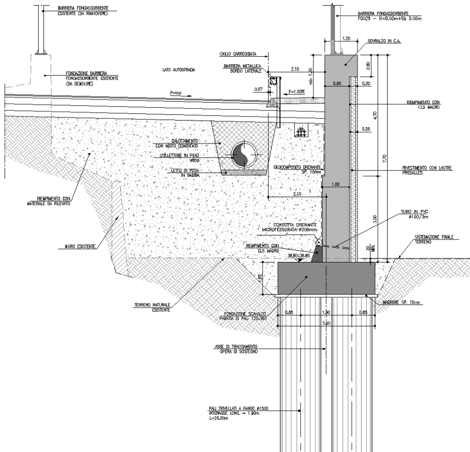
Figura 1-4 - Opera di scavalco linea TERNA esistente – Sezione in corrispondenza dei pali
