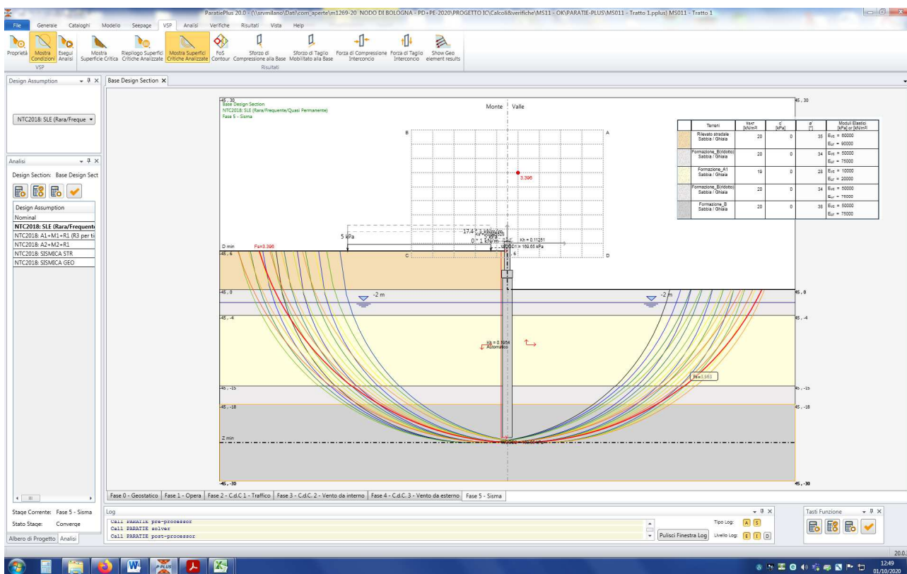
Figura n. 11.2 – Analisi di stabilità – Configurazione finale – Verifica sismica
