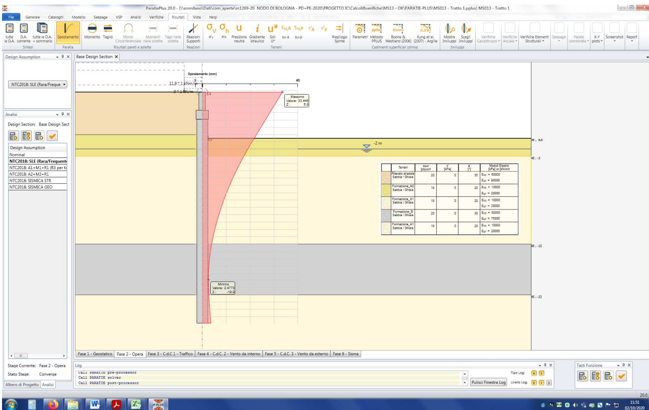
Figura n.10.7 – Spostamenti fase 2
