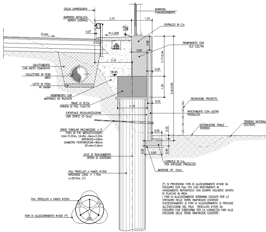
Figura n.1.1 – Sezione tipologica tratto eseguito da rilevato provvisorio
