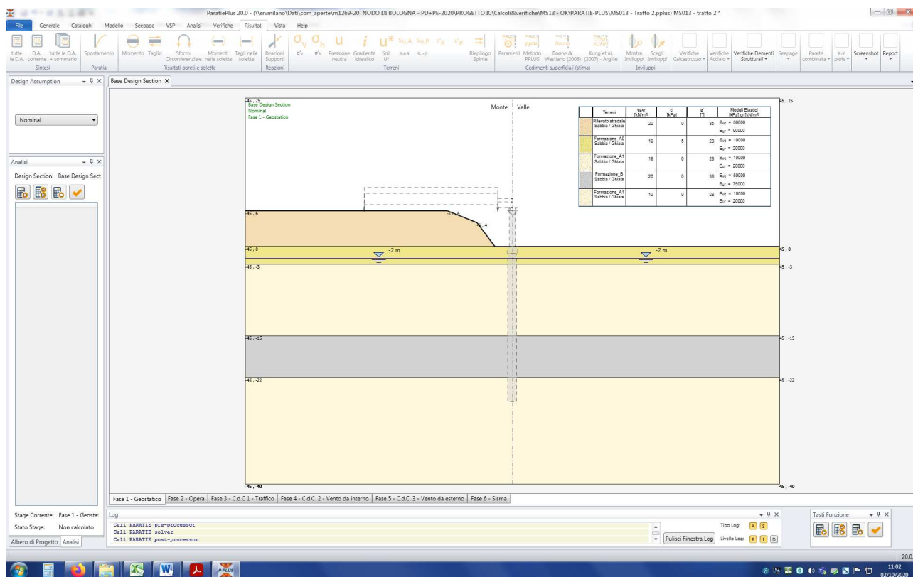
Figura n.8.1 - FASE 1 - Realizzazione del rilevato stradale esistente
