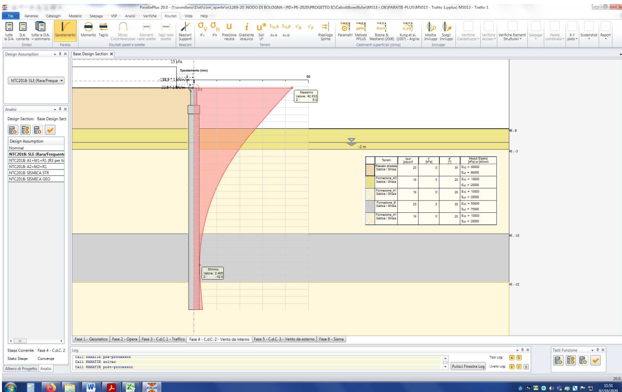
Figura n.10.8 – Spostamenti fase 4
