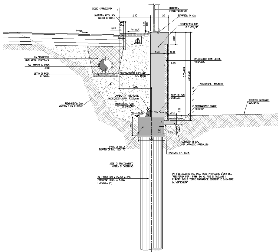
Figura n.1.2 – Sezione tipologica tratto eseguito da piano campagna
