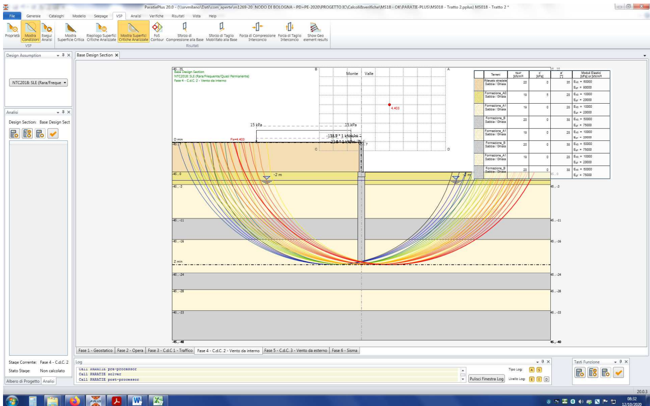
Figura n.11.1 – Analisi di stabilità – Configurazione finale – Verifica statica
