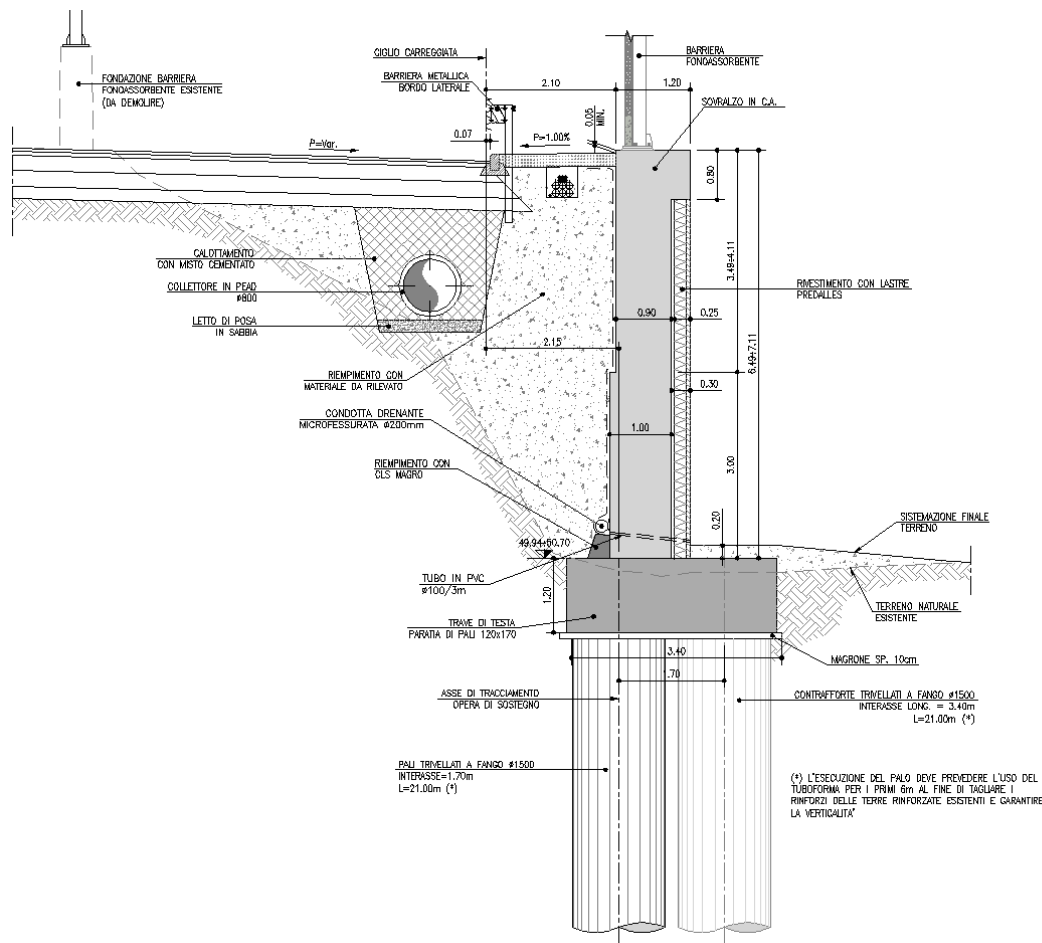
Figura n.1.2 – Sezione tipologica – Tratto eseguito da piano campagna
