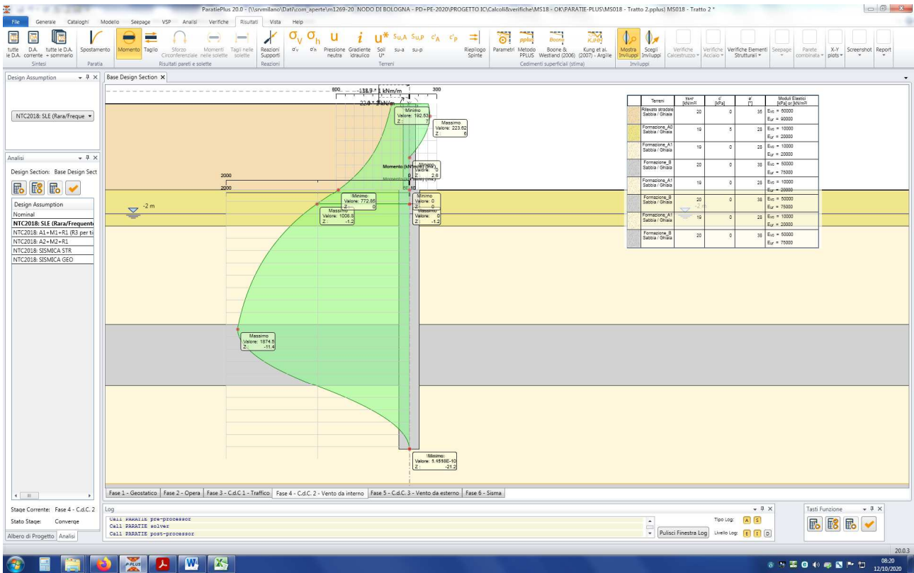
Figura n. 10.10 – Momento flettente - Inviluppo SLU
