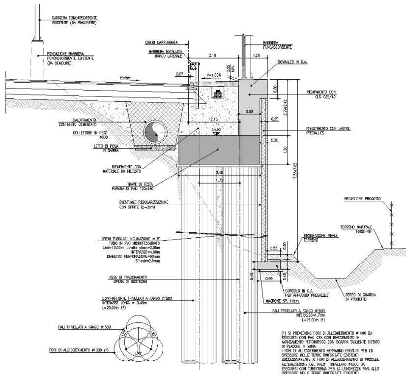
Figura n.1.1 – Sezione tipologica – Tratto eseguito da rilevato provvisorio
