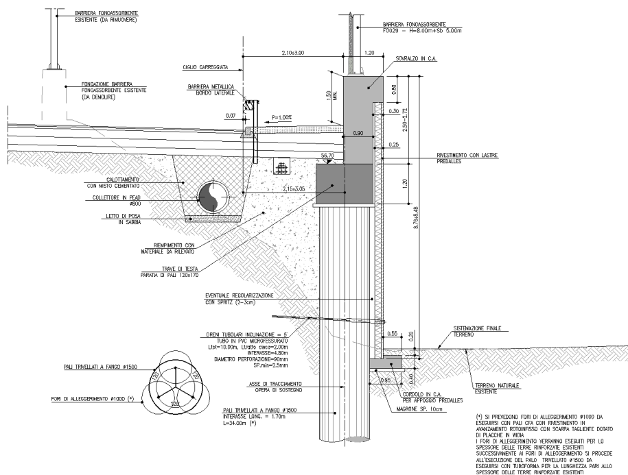
Figura 1-1. Sezione tipo opera di sostegno MS021 – Tratto 1
