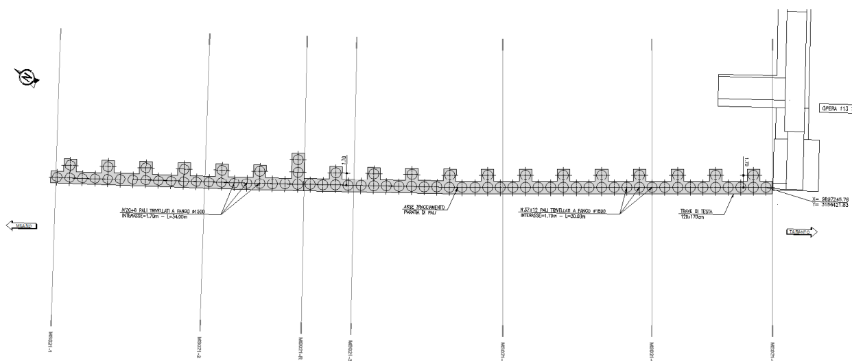
Figura 1-3. Pianta "contrafforti"
