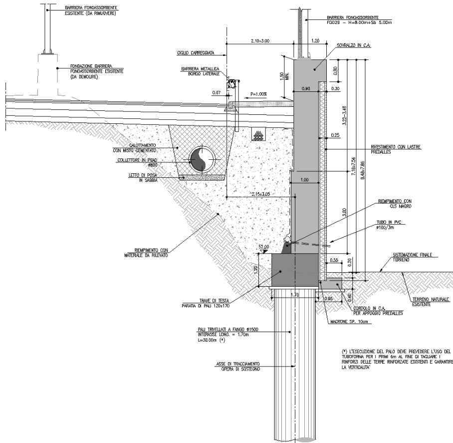
Figura 1-2. Sezione tipo opera di sostegno MS021 – Tratto 2
