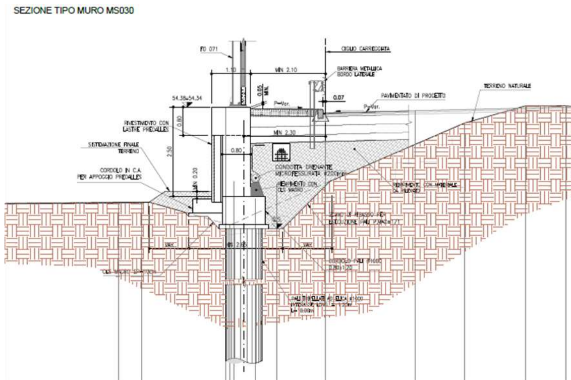
Figura 1-1. Sezione tipo opera di sostegno MS030
