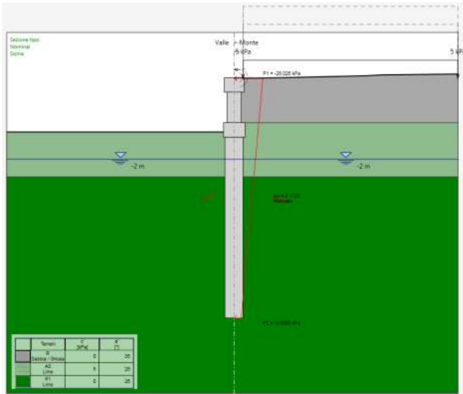
Figura 7-8. Diagramma di carico applicato al muro in condizioni sismiche
