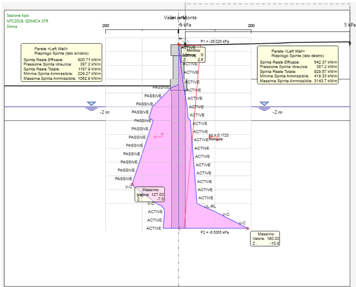
Figura 9-2. Riepilogo spinte fase 6 (sisma) – combinazione SLV
