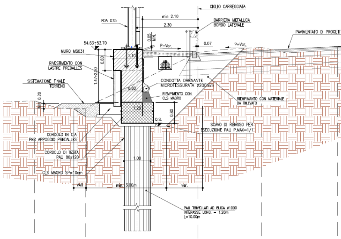
Figura 1-1. Sezione tipo opera di sostegno MS031
