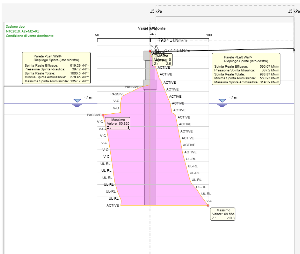
Figura 9-1. Riepilogo spinte fase 5 (vento dominante) – combinazione A2+M2+R1
