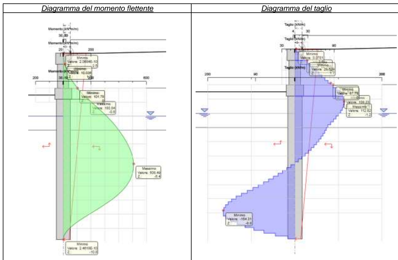
Figura 8-5. Sollecitazioni nelle strutture nella combinazione SLV (sisma)
