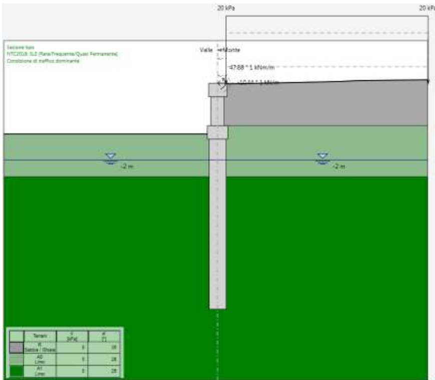
Figura 7-5 Carichi esterni agenti sul muro in condizioni di traffico dominante
