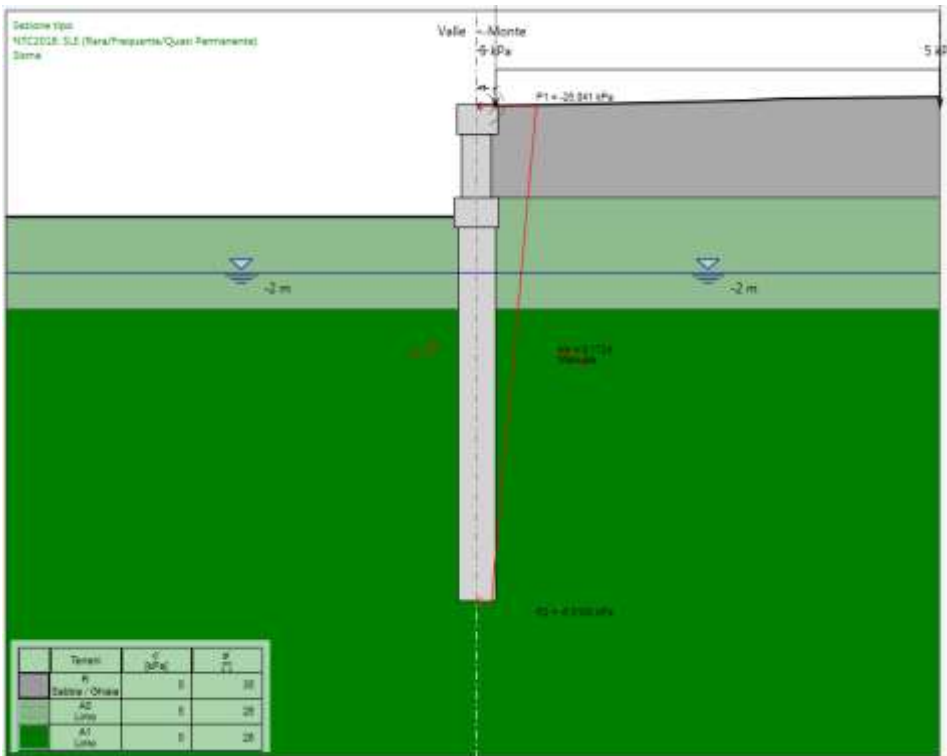
Figura 7-8. Diagramma di carico applicato al muro in condizioni sismiche
