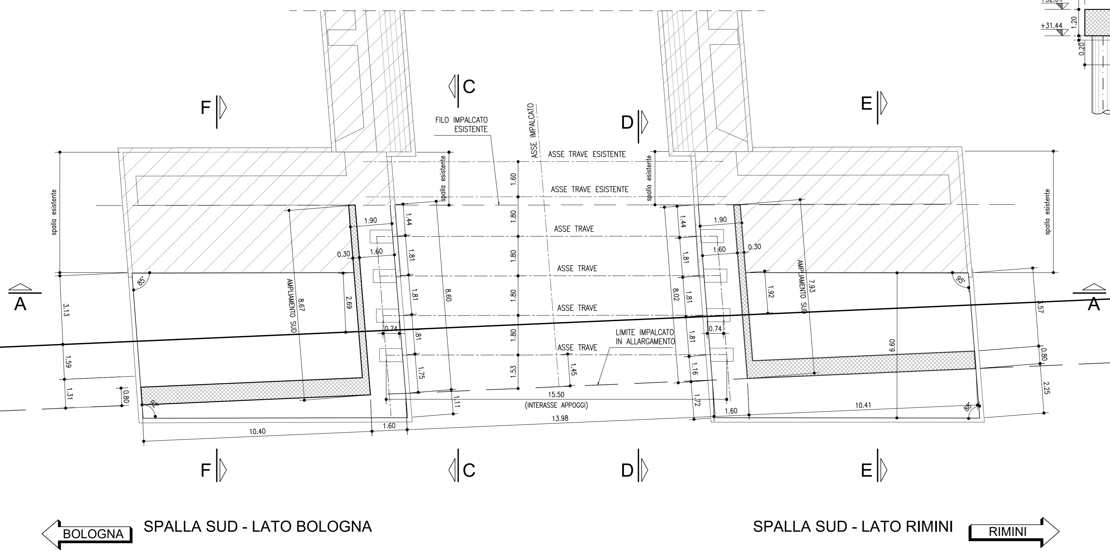
PIANTA SPALLE E MURI D'ALA CARREGGIATA SUD Scala 1:100
