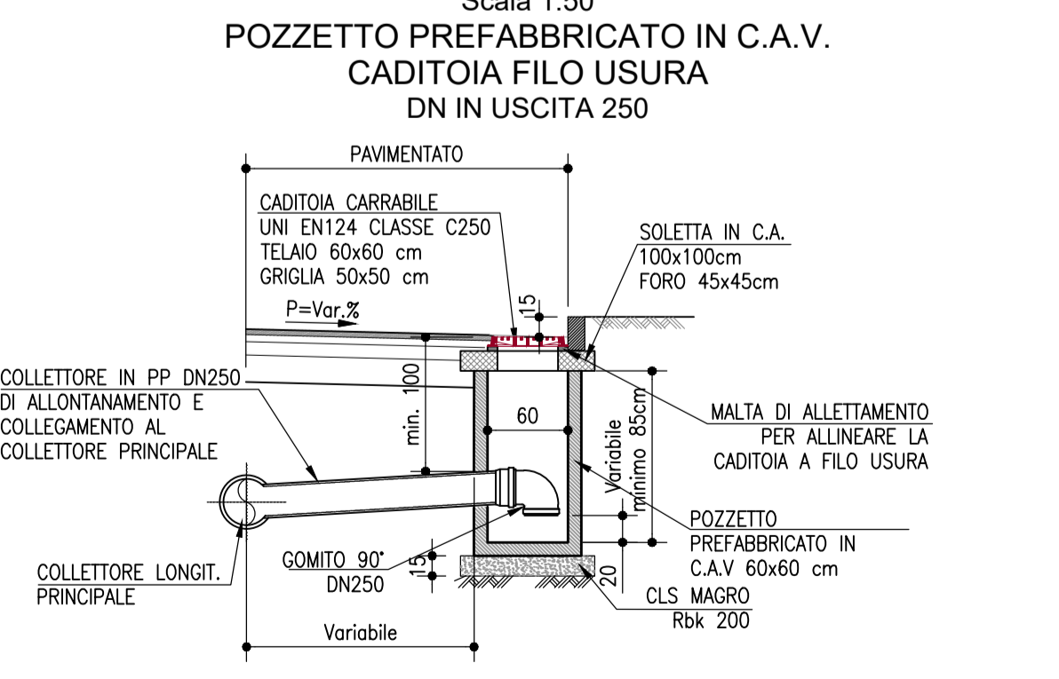
PARTICOLARI IDRAULICI
