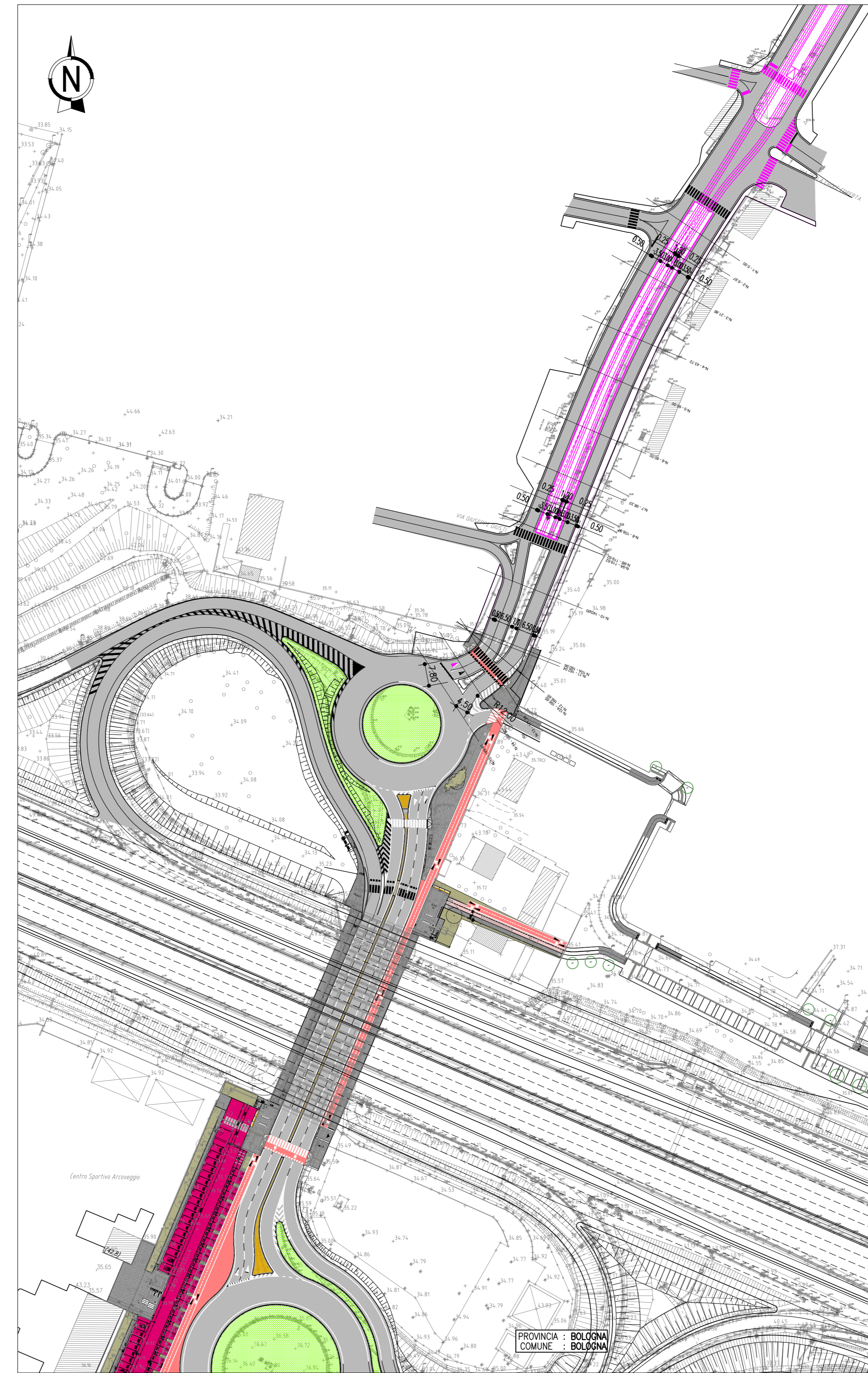
PLANIMETRIA DI PROGETTO - ROTATORIA 3 - RAMO NORD 1:1000
