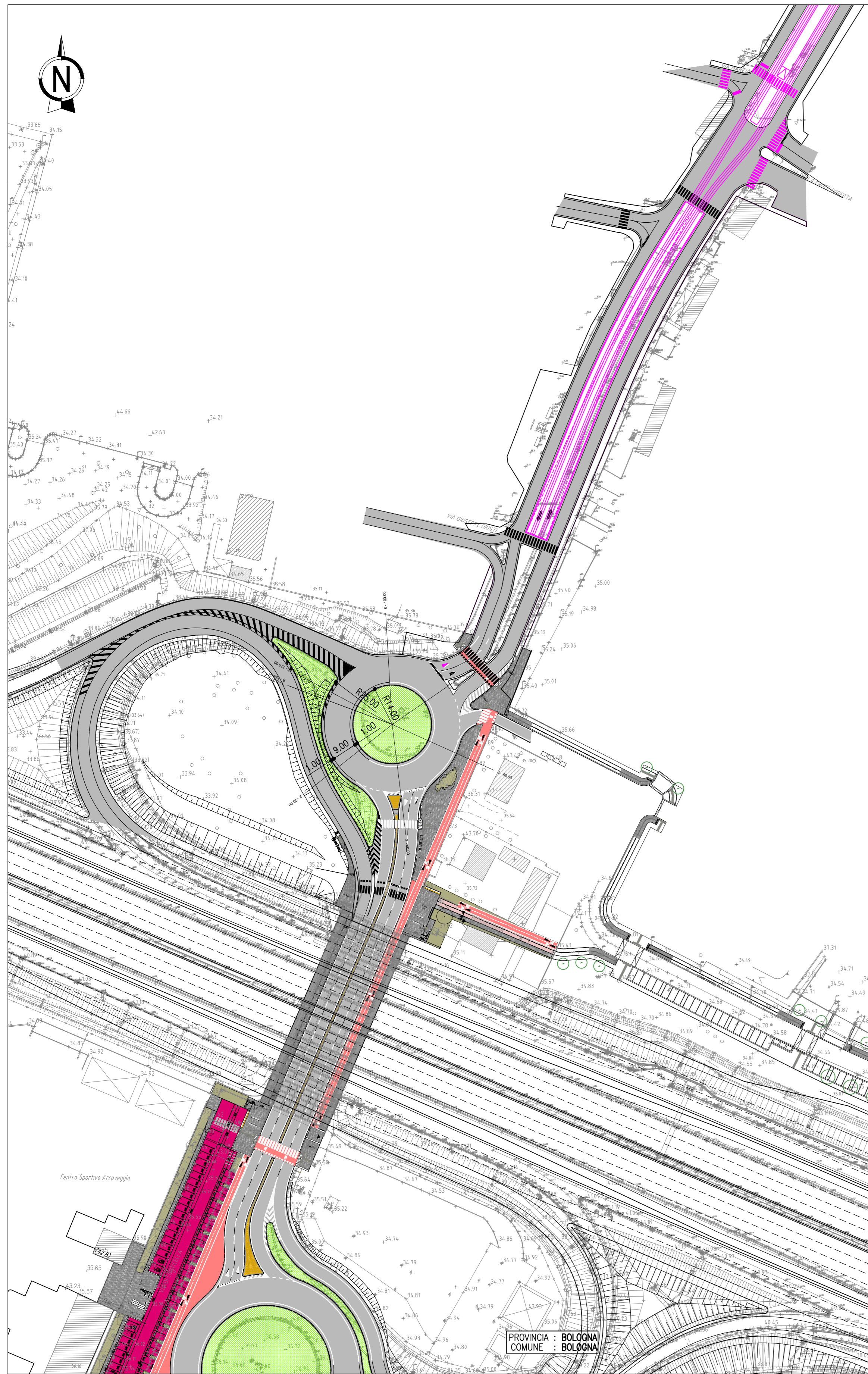
PLANIMETRIA DI PROGETTO - ROTATORIA 3 1:1000
