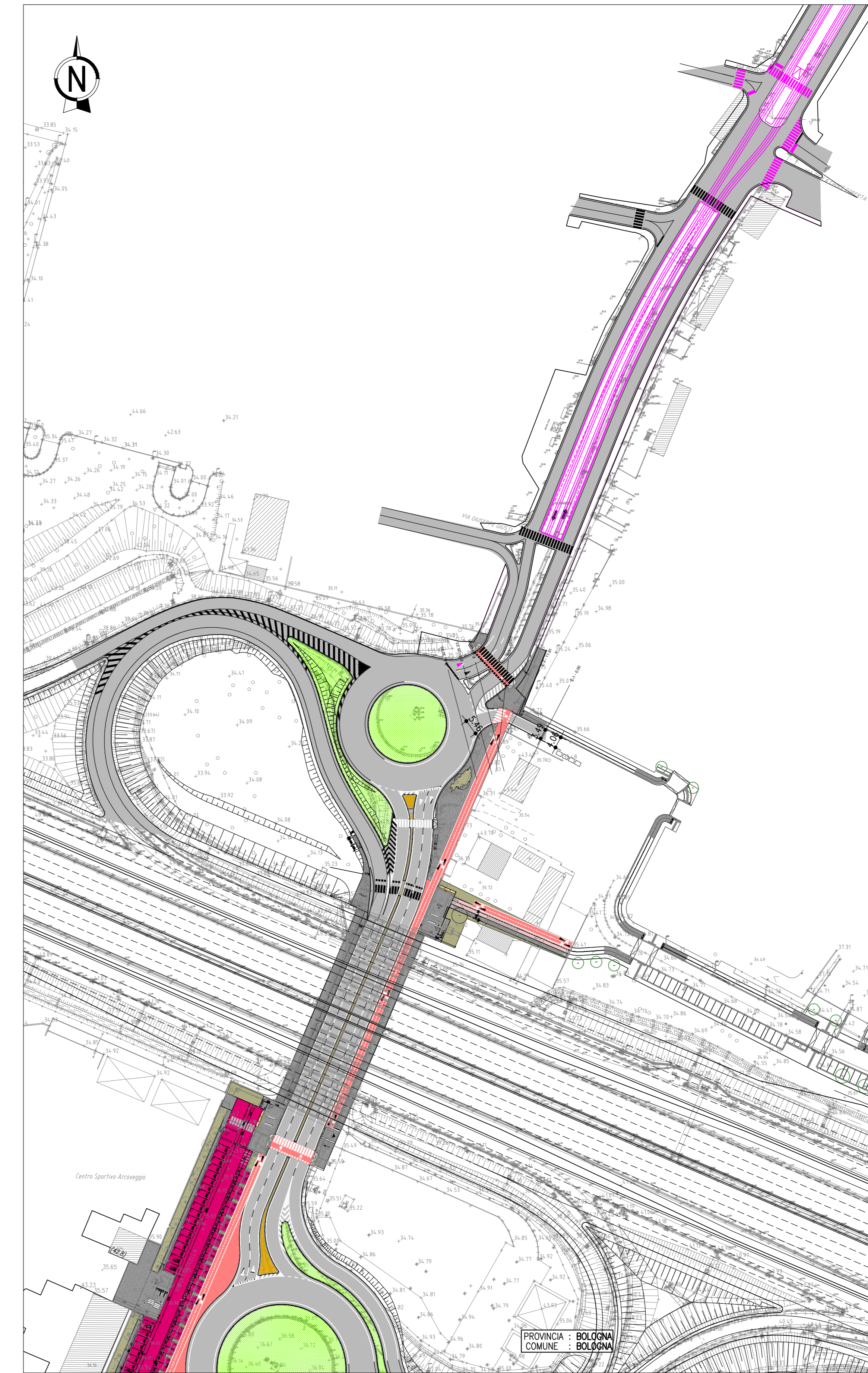
PLANIMETRIA DI PROGETTO - ROTATORIA 3 - RAMO EST 1:1000
