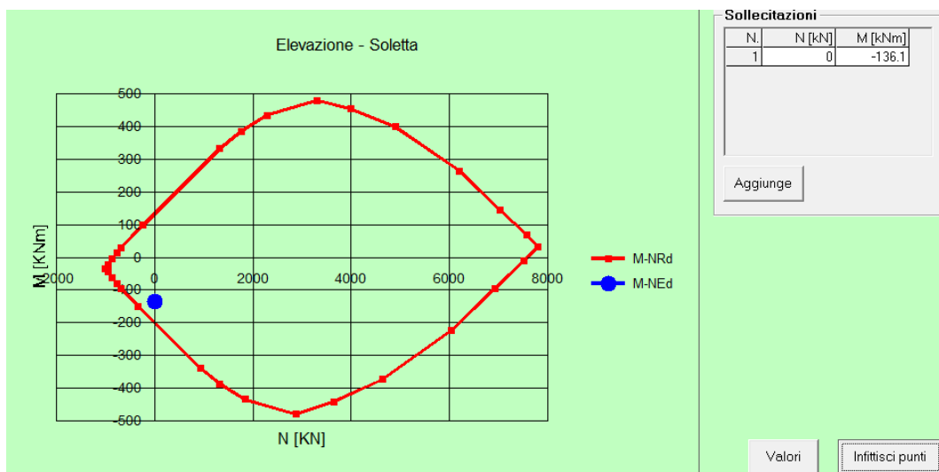
Figura 8.11: Dominio M-N - Momento Negativo
