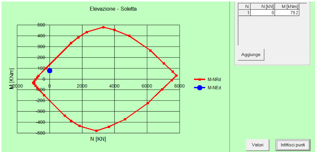
Figura 8.13: Dominio M-N - Momento Positivo
