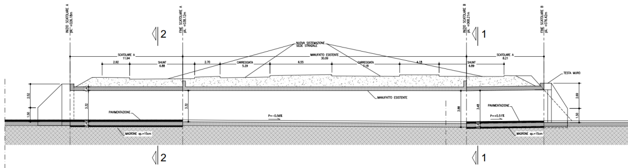
Figura 1.2: Sezione longitudinale
