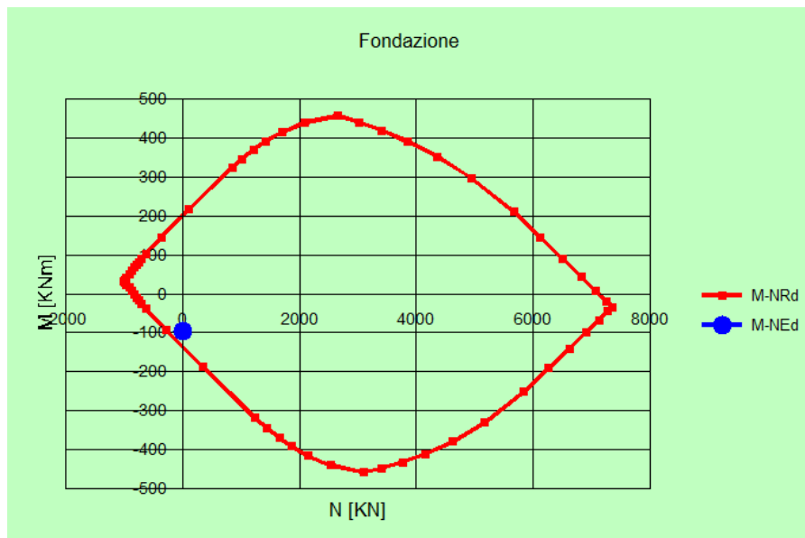
Figura 8.8: Momento resistente fondazione – Momento Negativo
