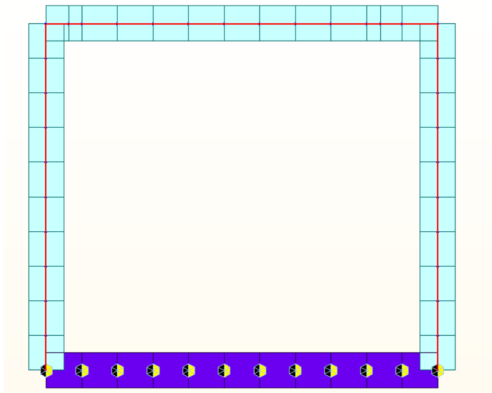
Figura 12 Vincoli applicati al modello a elementi finiti dello scatolare
