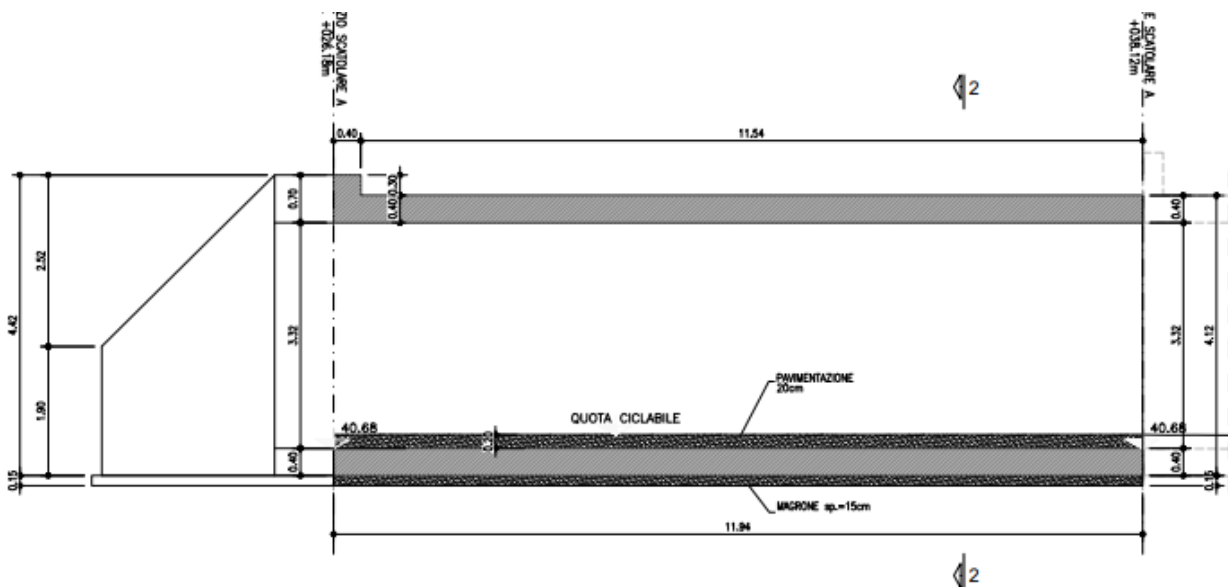
Figura 1.3: Sottopasso A
