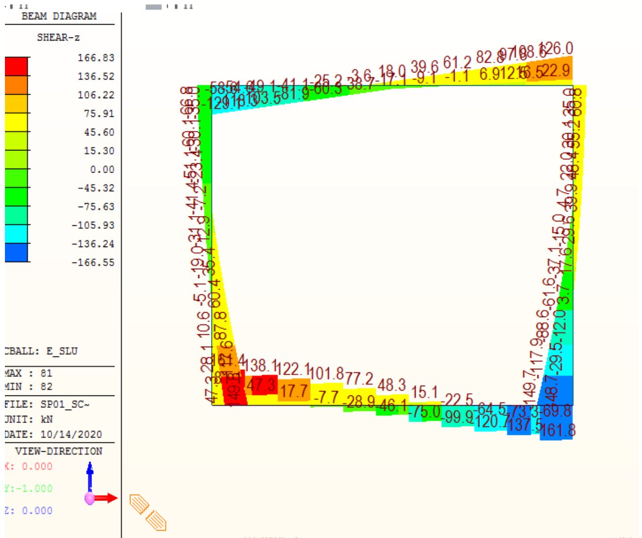
Figura 7.2: Comb.SLU – Taglio
