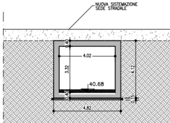
Figura 1.5: Scatolare A - Sezione trasversale
