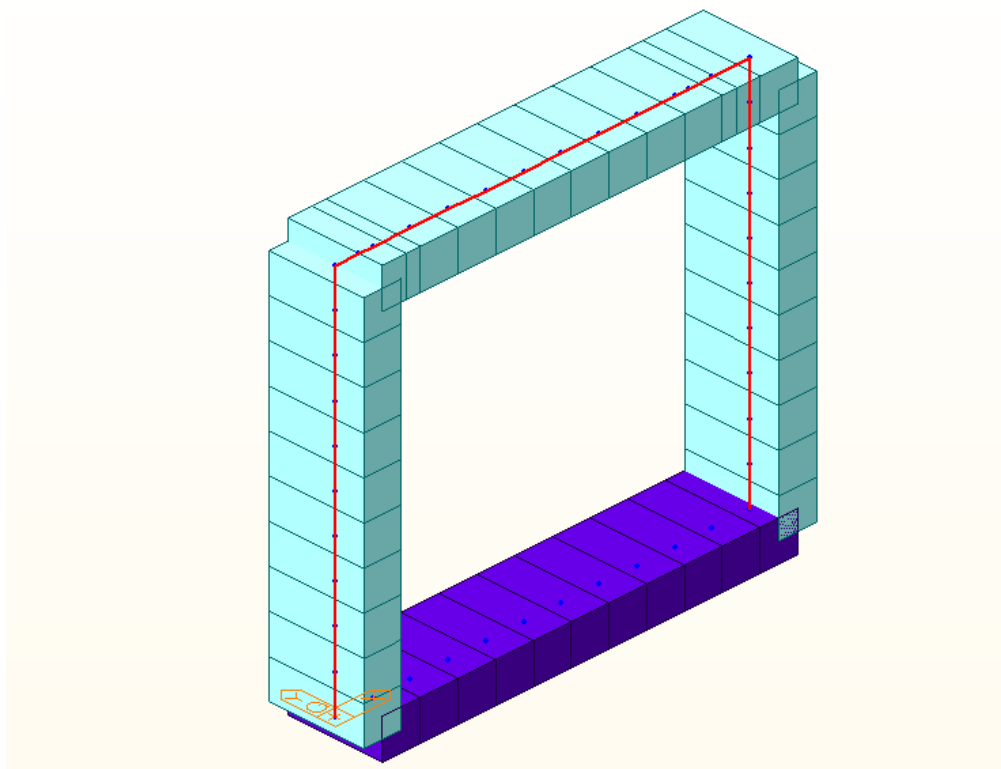
Figura 9 - Modello F.E.M struttura
