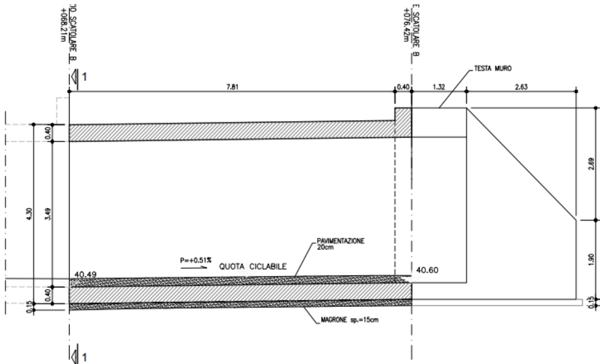
Figura 1.4: Sottopasso B
