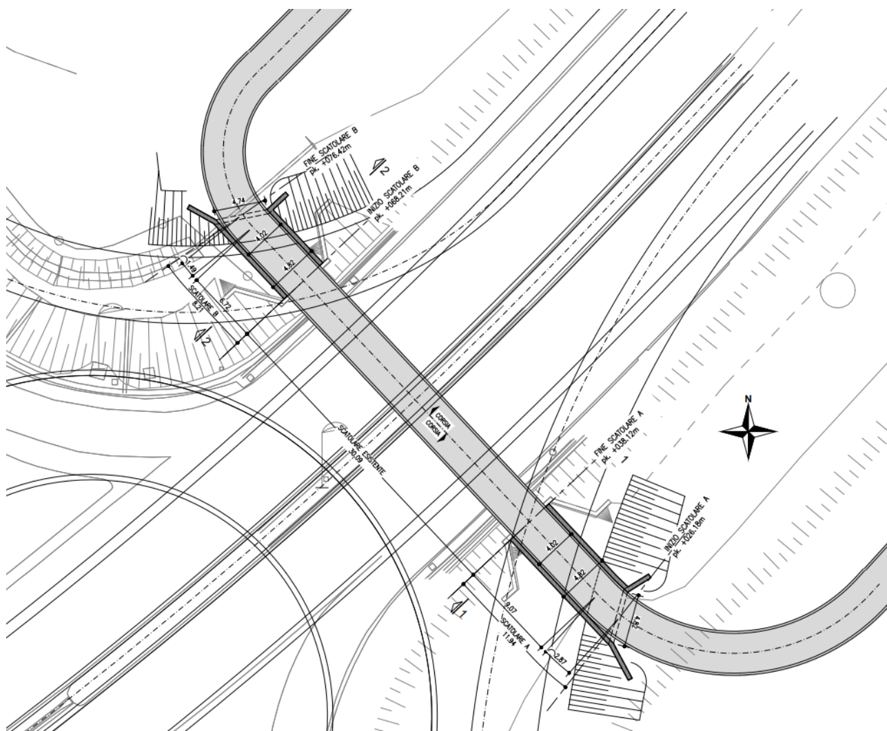
Figura 1.1: Planimetria
