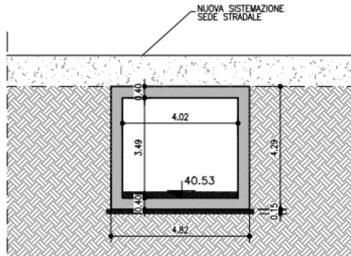
Figura 1.6: Scatolare B - Sezione trasversale
