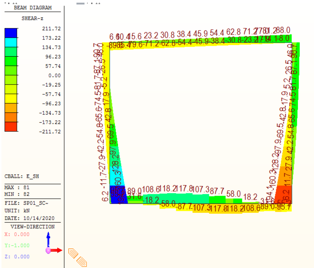
Figura 7.4: Comb.SLV – Taglio
