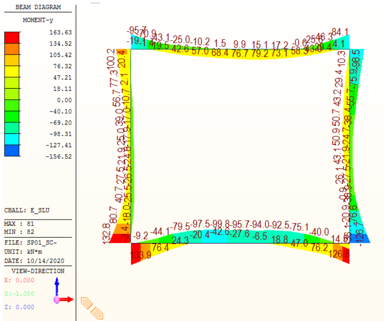
Figura 7.1: Comb.SLU – Momento
