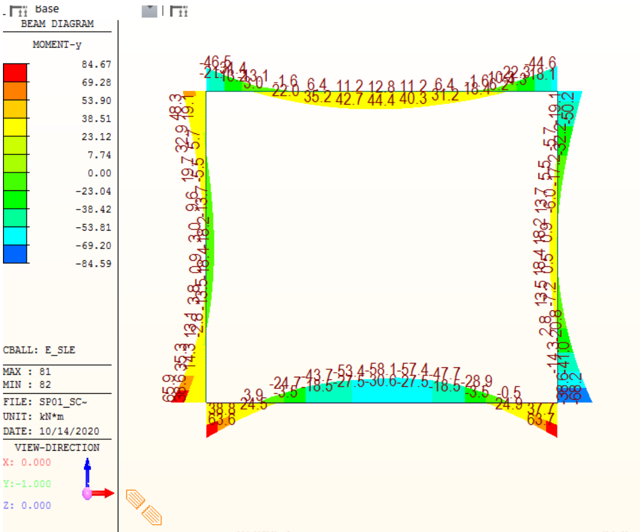
Figura 7.5: Comb.SLE - Momento
