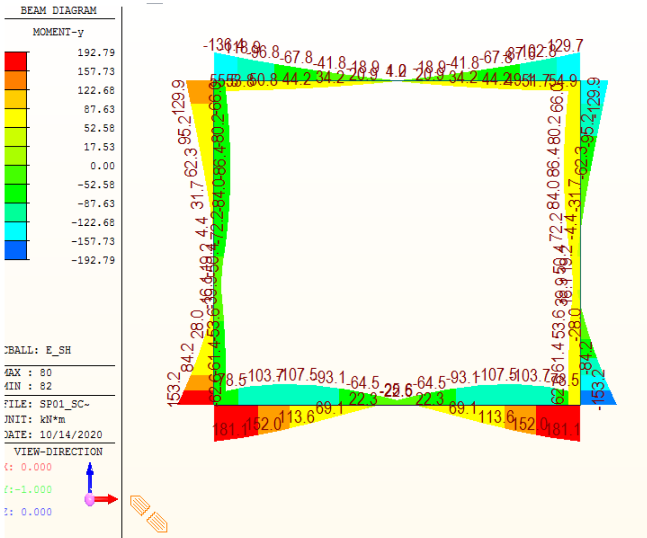
Figura 7.3: Comb.SLV - Momento
