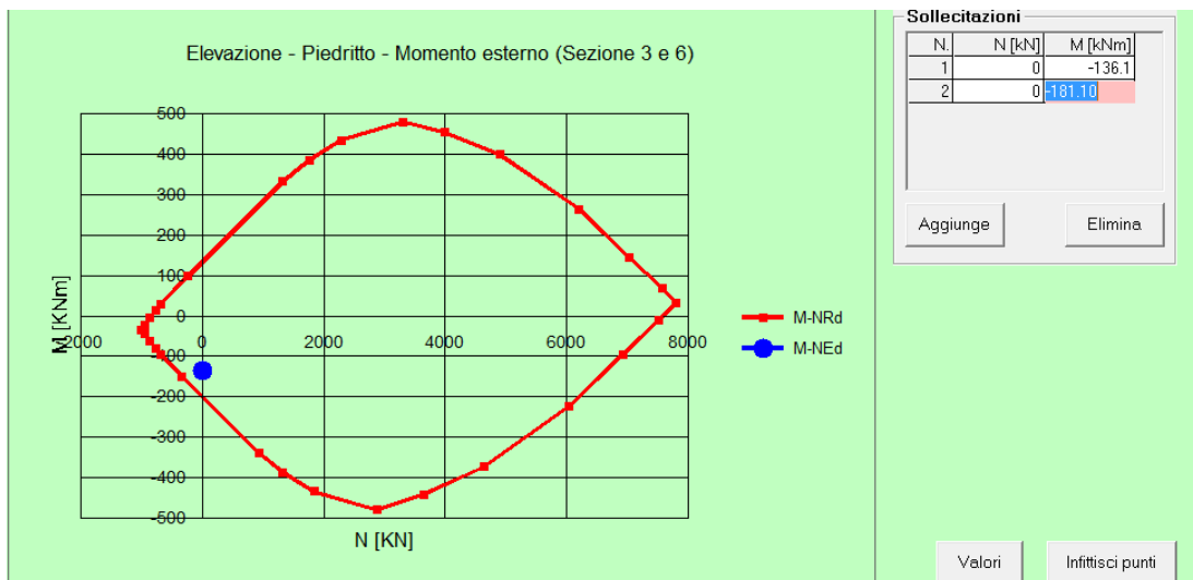
Figura 8.14: Momento resistente – Piedritti
