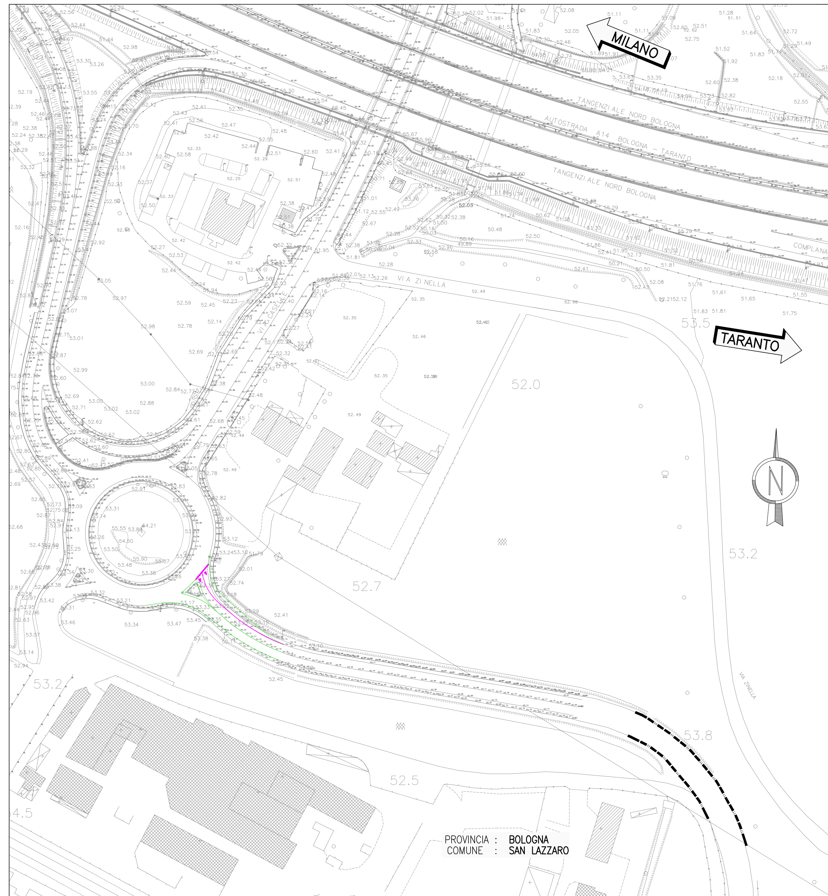
ROTATORIA RO010: PLANIMETRIA DELLE RIMOZIONI
