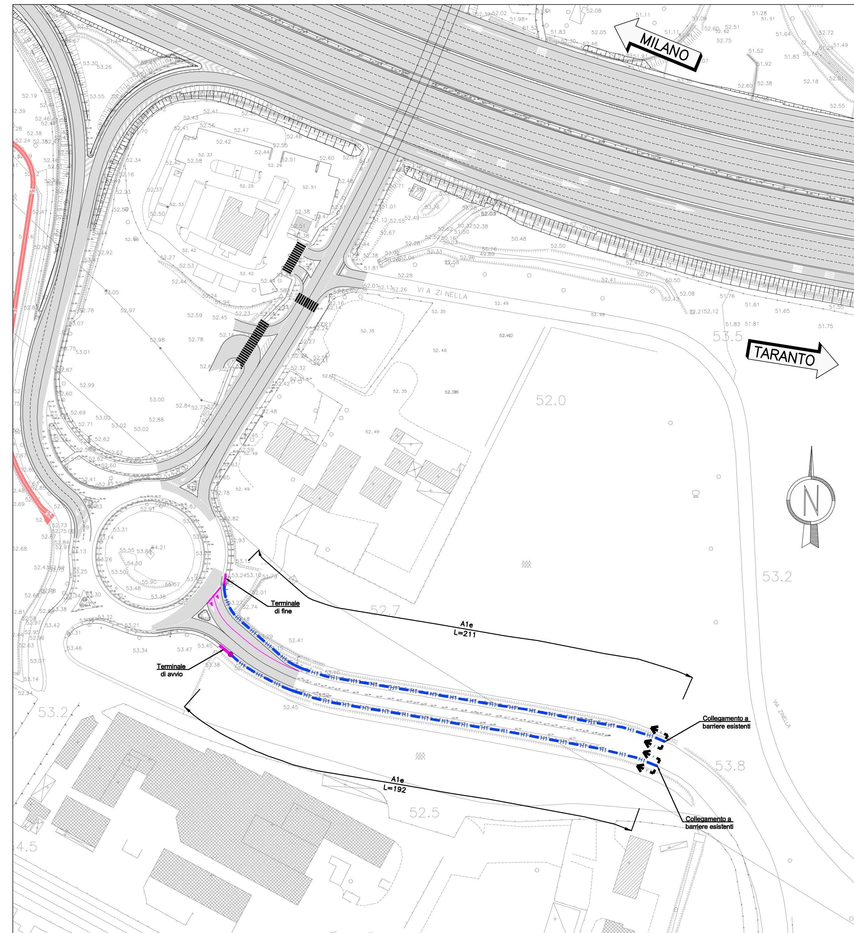
ROTATORIA RO010: PLANIMETRIA DI PROGETTO
