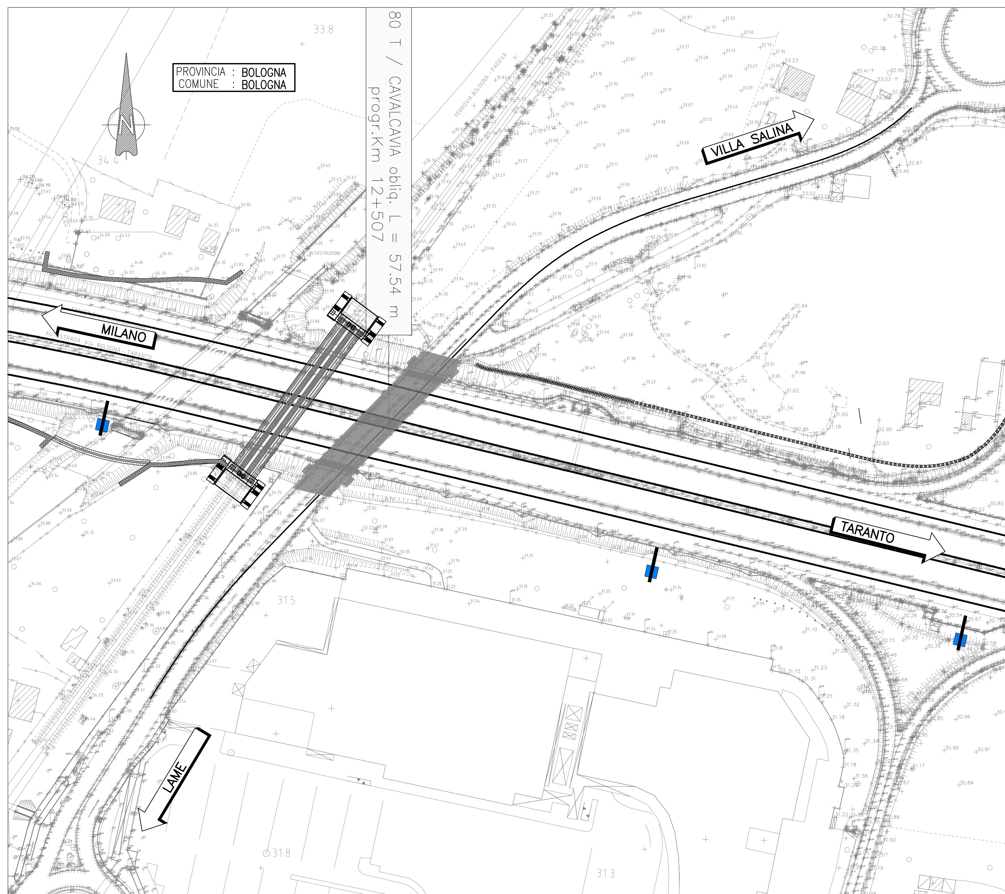
PLANIMETRIA DI TRACCIAMENTO - scala 1:1000
