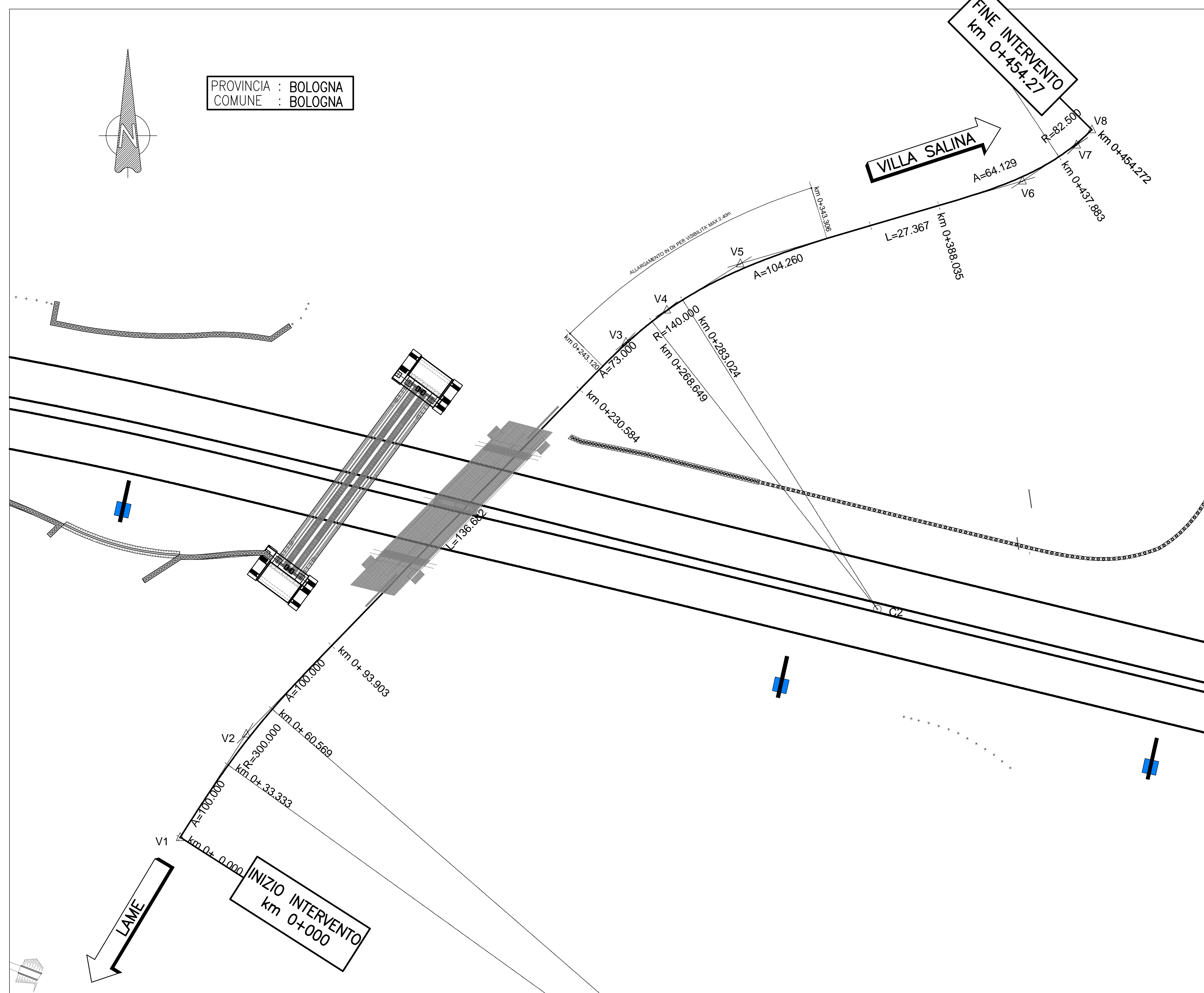
PLANIMETRIA DI TRACCIAMENTO - scala 1:1000
