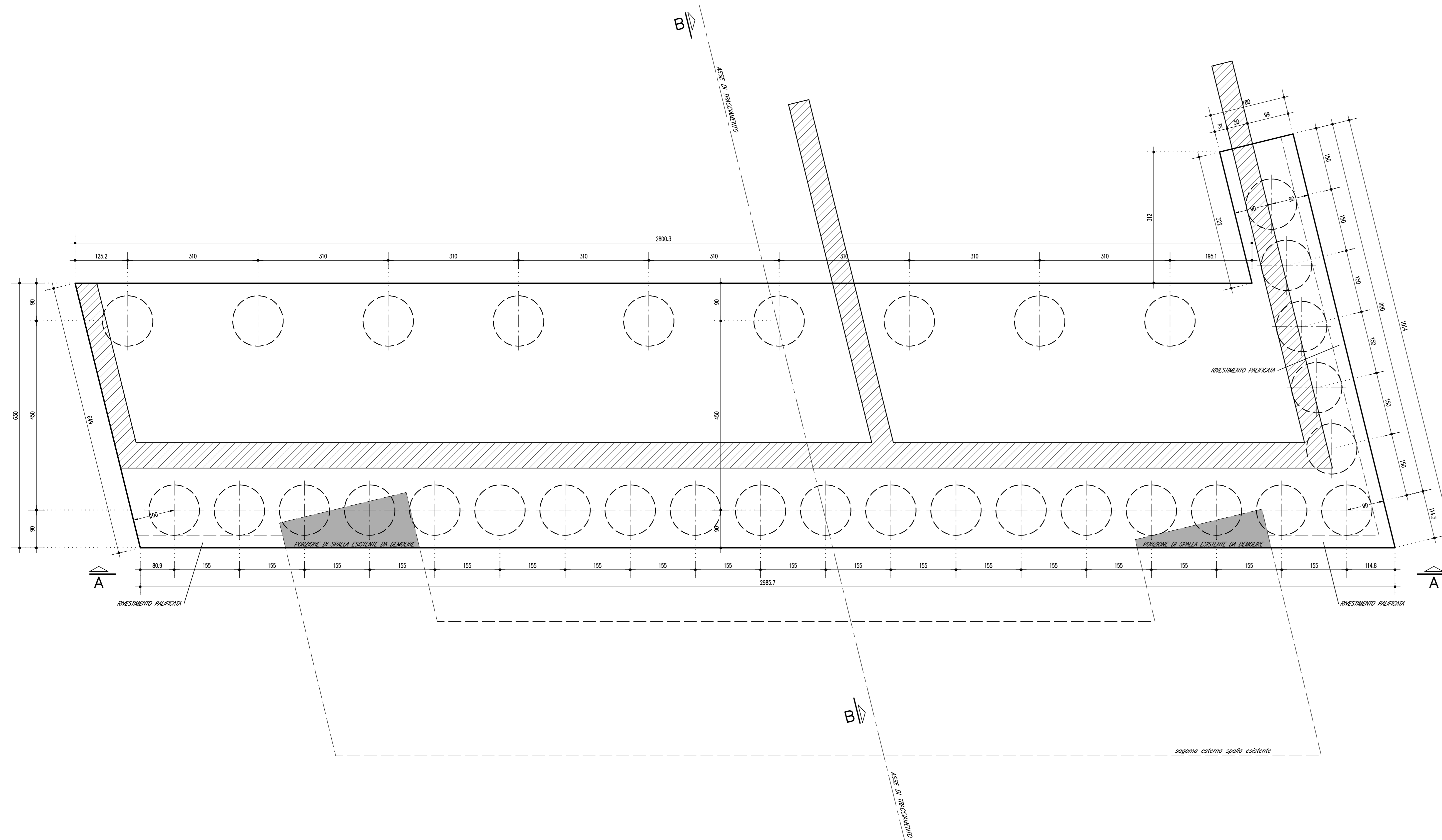
PIANTA FONDAZIONE E SPICCATO ELEVAZIONE 1:50 (n.33 PALI Ø120cm L=30,00m)
