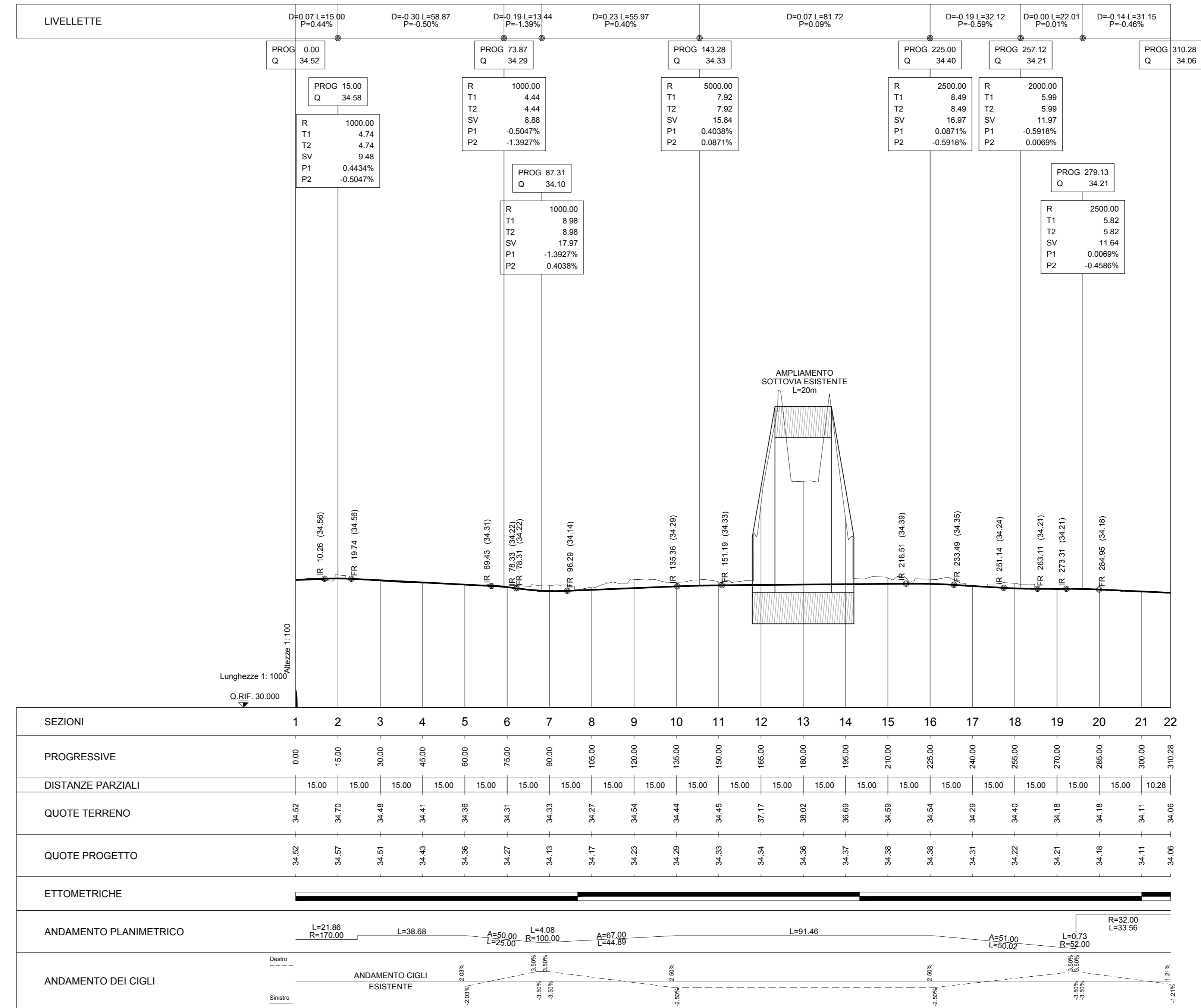
PROFILO LONGITUDINALE - ADEGUAMENTO VIA COLOMBO - ASSE EST 1:1000
