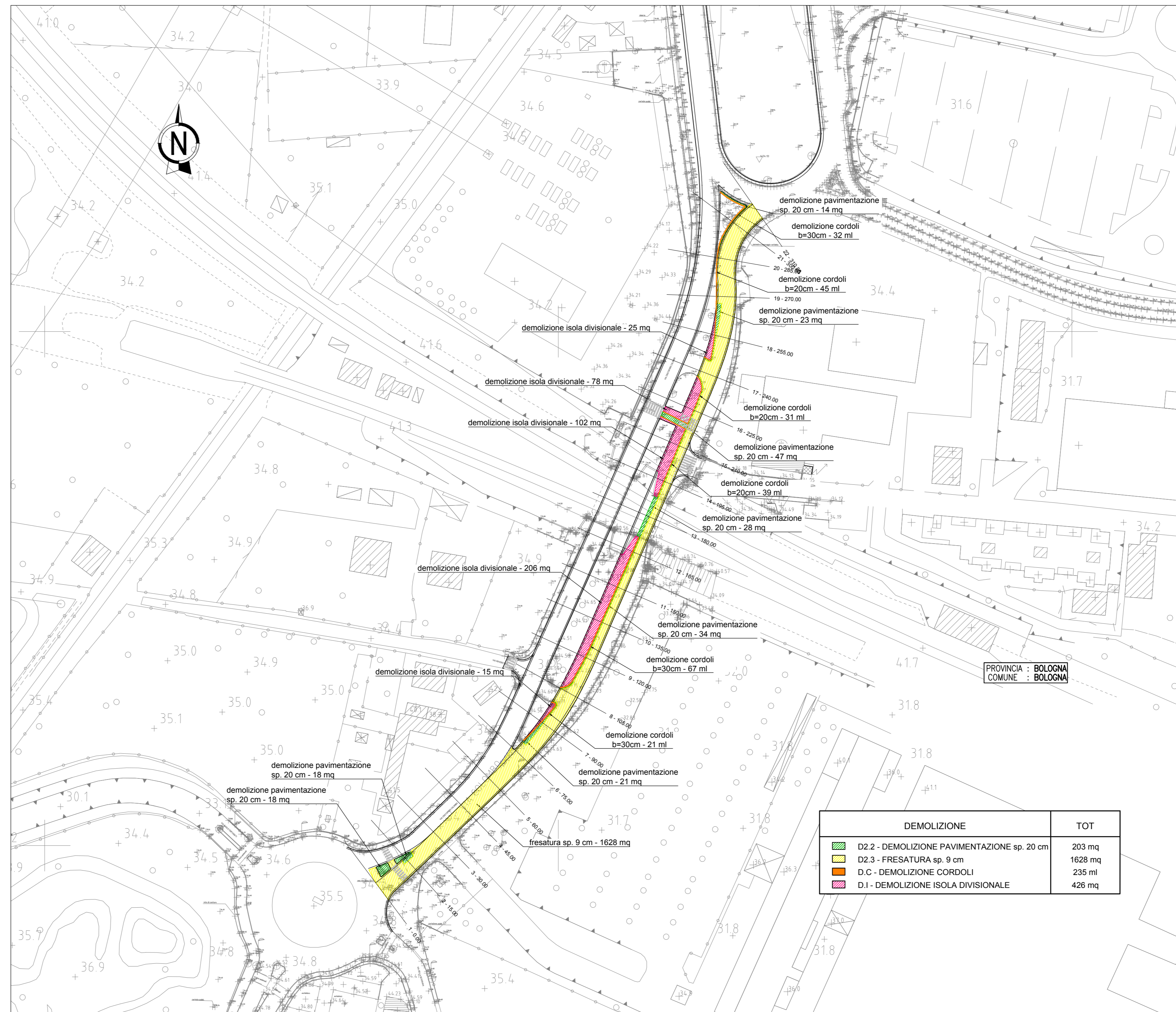
PLANIMETRIA DELLE DEMOLIZIONI - ADEGUAMENTO VIA COLOMBO - ASSE EST 1:1000
