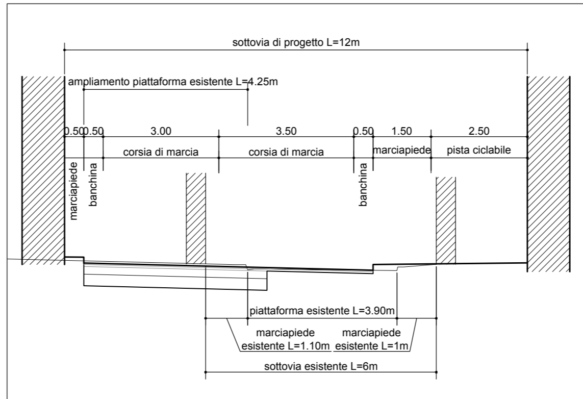
SEZIONE TIPOLOGICA DI PROGETTO B-B 1:100
