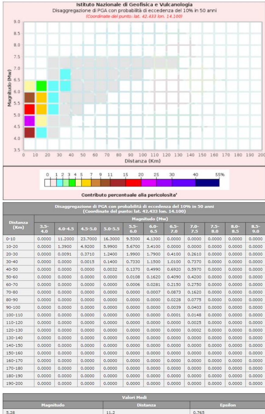
Fig. 2.13: Disaggregazione del valore di a(g) con probabilità di eccedenza del 10% in 50 anni, per il valore massimo di pericolosità atteso nel comune di Spoltore.
