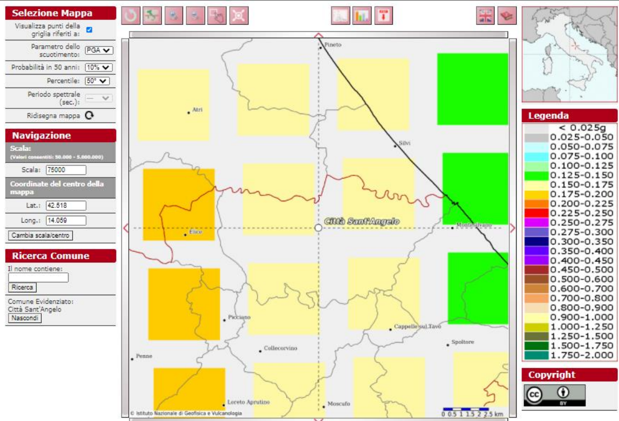
Fig. 2.8: Mappa di pericolosità sismica del comune di Città Sant'Angelo.
