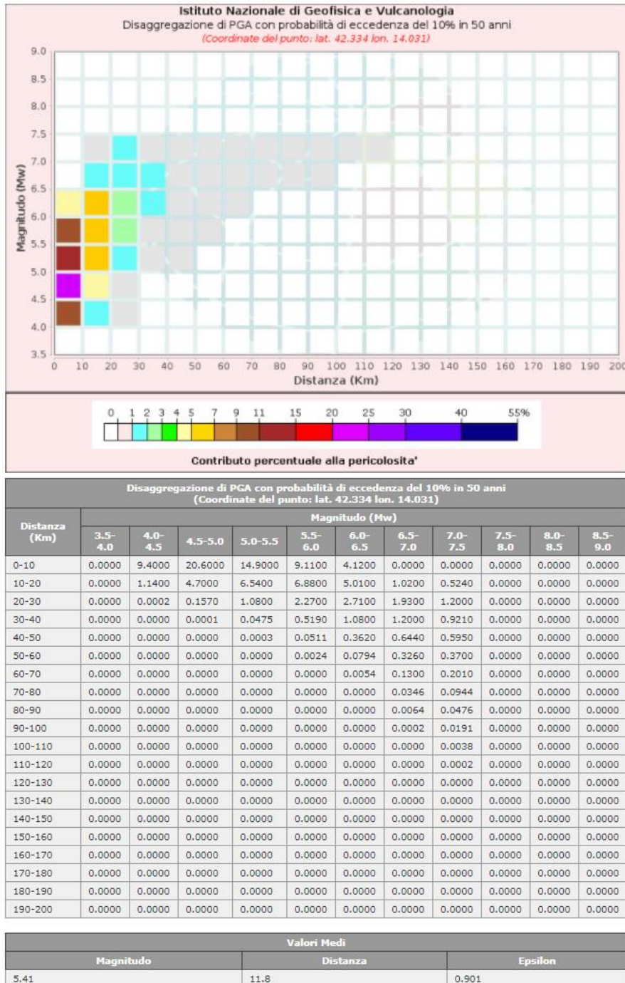
Fig. 2.23: Disaggregazione del valore di a(g) con probabilità di eccedenza del 10% in 50 anni, per il valore massimo di pericolosità atteso nel comune di Rosciano.
