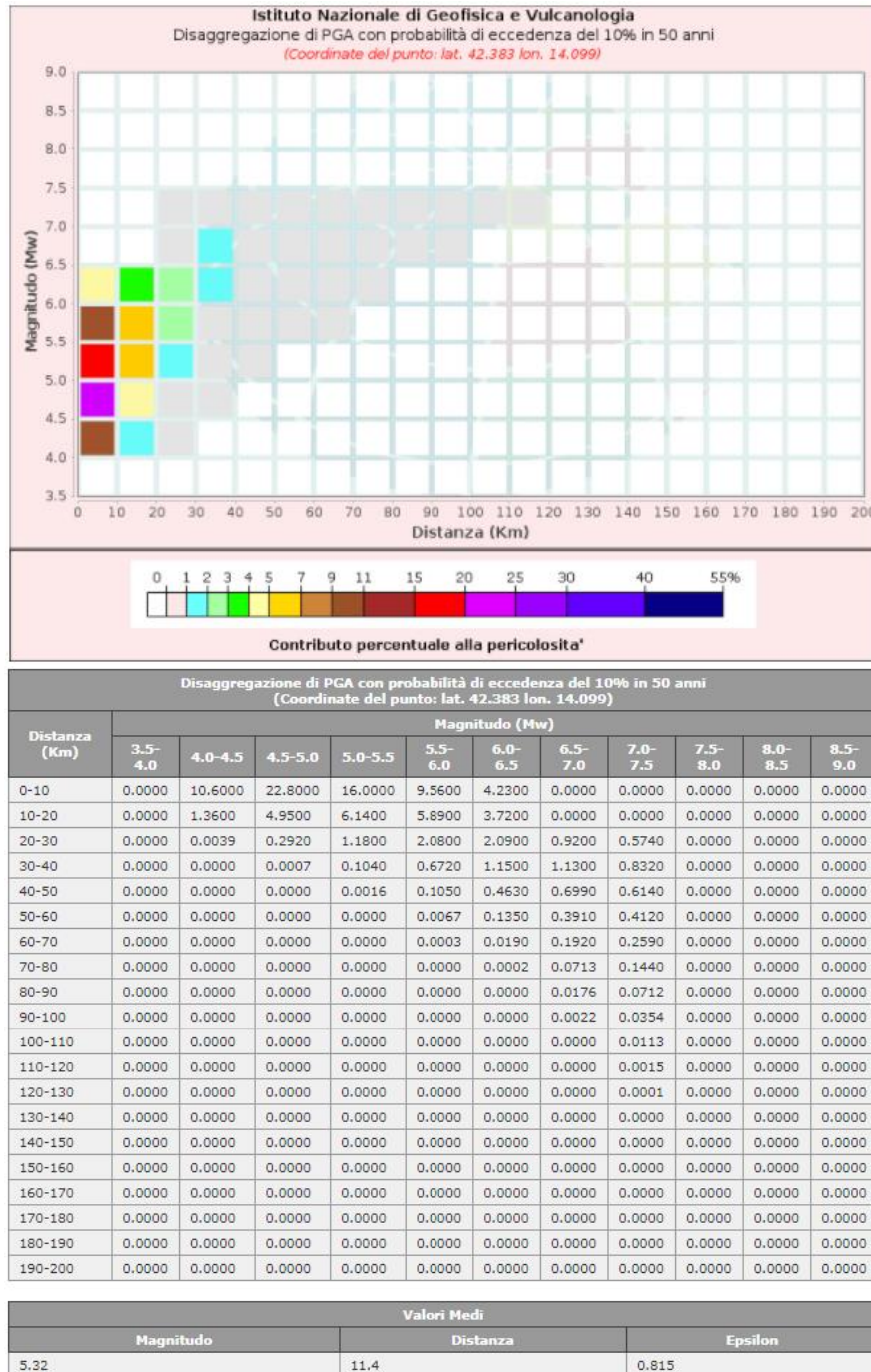
Fig. 2.19: Disaggregazione del valore di a(g) con probabilità di eccedenza del 10% in 50 anni, per il valore massimo di pericolosità atteso nel comune di Cepagatti.
