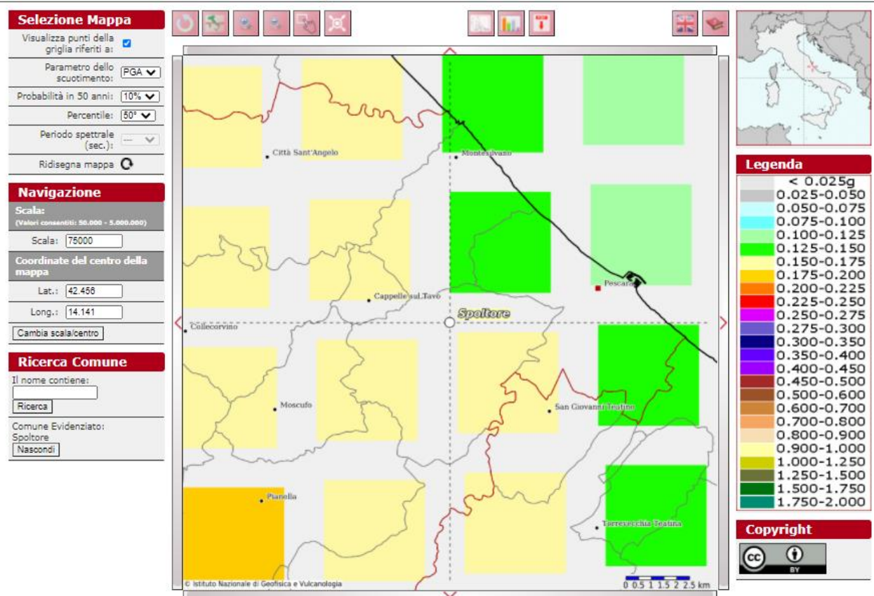
Fig. 2.12: Mappa di pericolosità sismica del comune di Spoltore.
