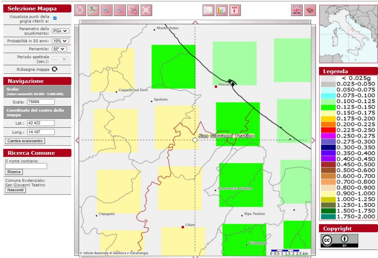
Fig. 2.16: Mappa di pericolosità sismica del comune di San Giovanni Teatino.
