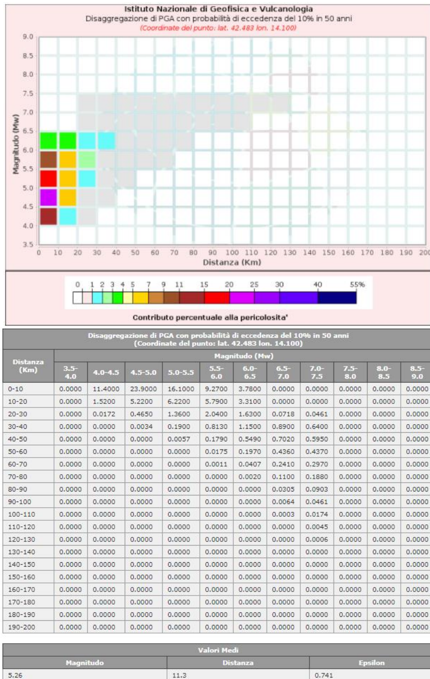
Fig. 2.11: Disaggregazione del valore di a(g) con probabilità di eccedenza del 10% in 50 anni, per il valore massimo di pericolosità atteso nel comune di Montesilvano.
