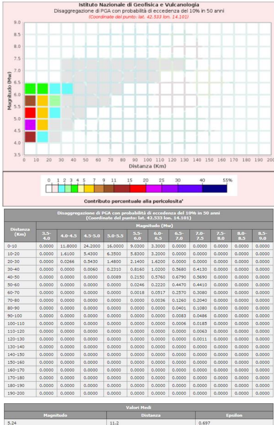
Fig. 2.9: Disaggregazione del valore di a(g) con probabilità di eccedenza del 10% in 50 anni, per il valore massimo di pericolosità atteso nel comune di Città Sant'Angelo.
