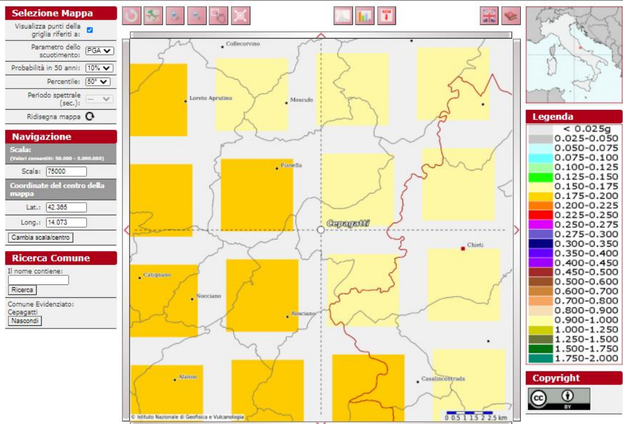
Fig. 2.18: Mappa di pericolosità sismica del comune di Cepagatti.
