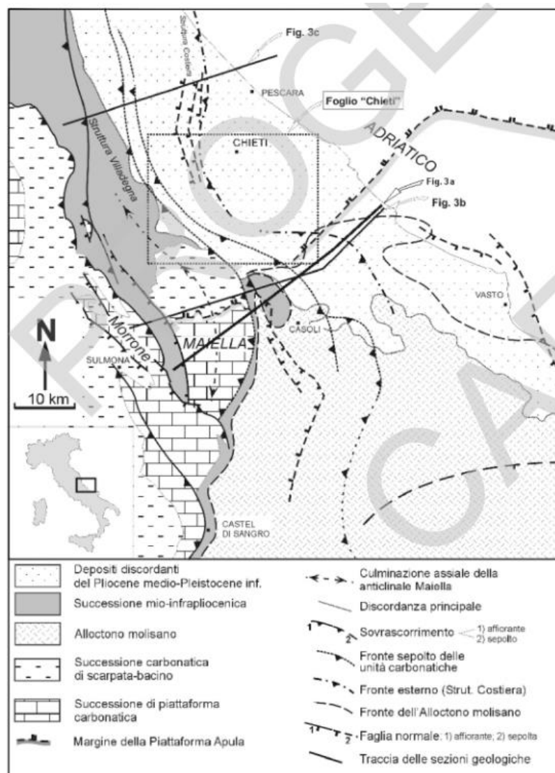
Fig. 2.1 Schema strutturale del settore esterno Abruzzese
