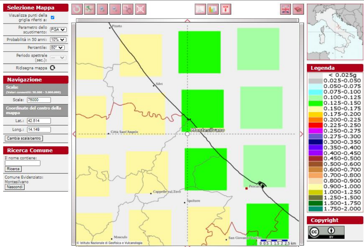
Fig. 2.10: Mappa di pericolosità sismica del comune di Montesilvano.
