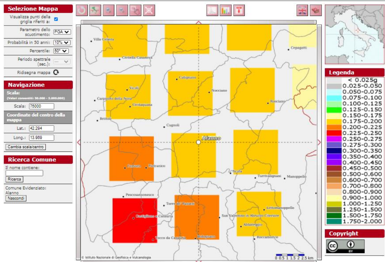
Fig. 2.24: Mappa di pericolosità sismica del comune di Alanno.
