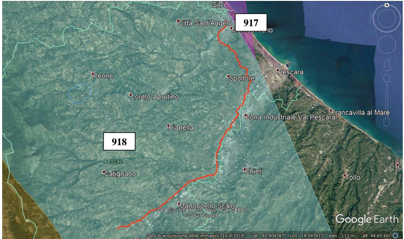
Fig. 2.29: Zonazione sismogenetica ZS9. In rosso il tracciato in progetto.
