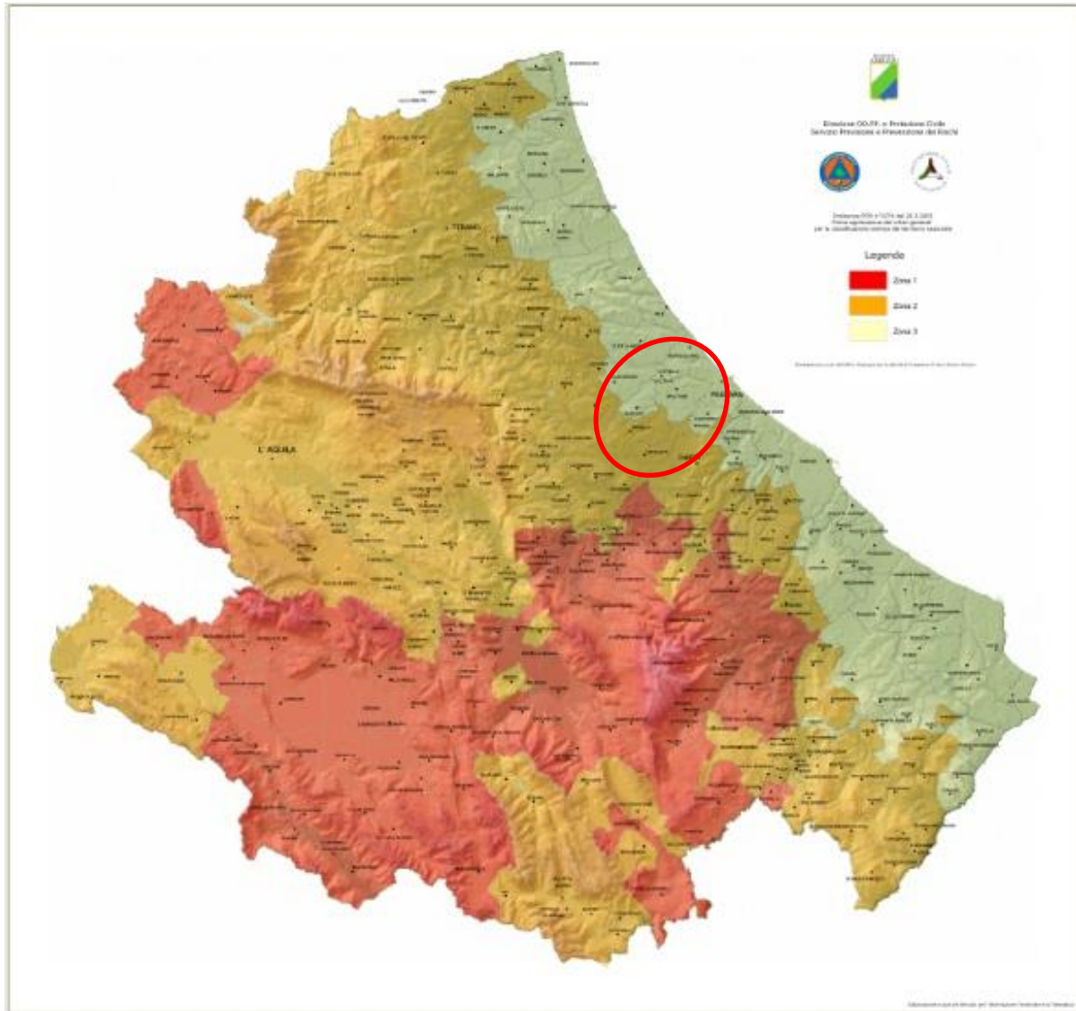
Fig. 2.6: Classificazione sismica della Regione Abruzzo in base all'Ordinanza del Presidente del Consiglio dei Ministri n. 3274 del 20 marzo 2003 – Delibera della Giunta Regionale n. 438 del 29 Marzo 2003.
