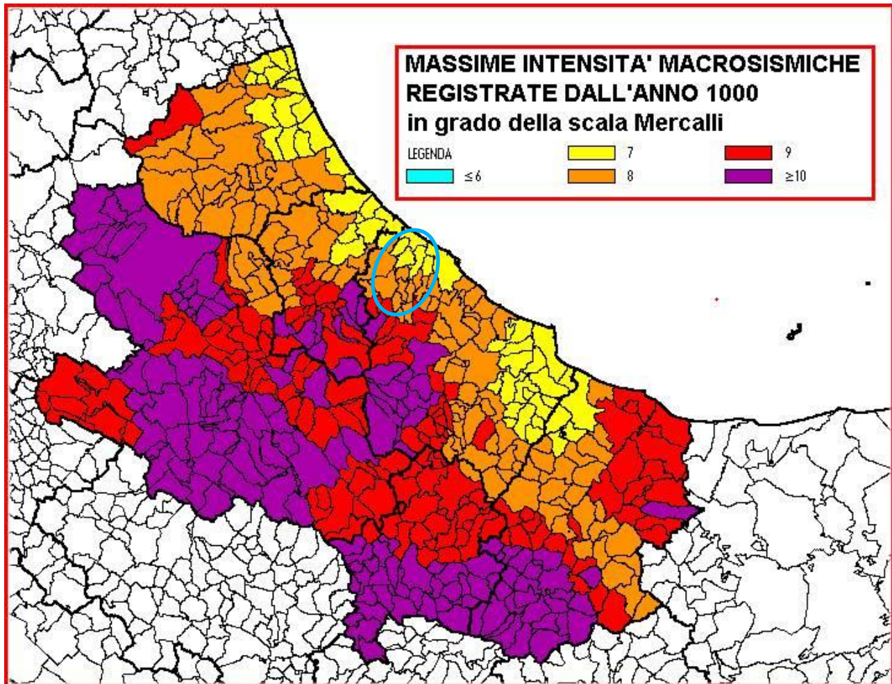
Fig. 2.27: Massime intensità sismiche (MCS) riscontrate nel territorio abruzzese e molisano.
