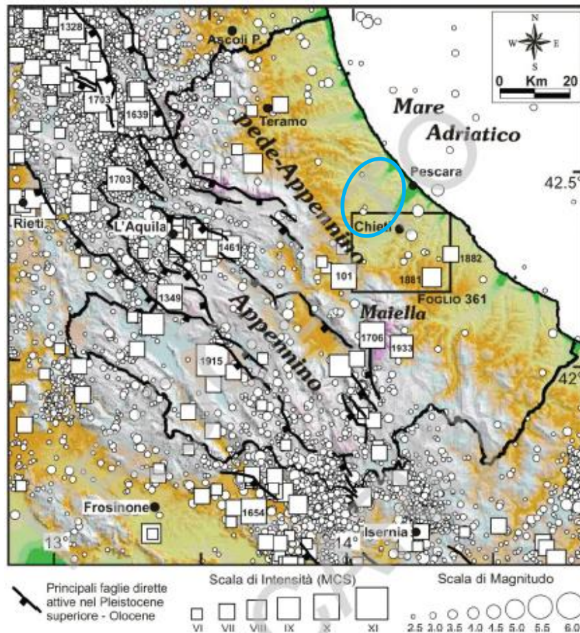
Fig. 2.26: Epicentri dei terremoti storici relativi al periodo 216 a.c. – 1992 (quadrati) e dei terremoti strumentali (cerchi) dal 1983 al 2003, con riportate le faglie attive nell'area appenninica.
