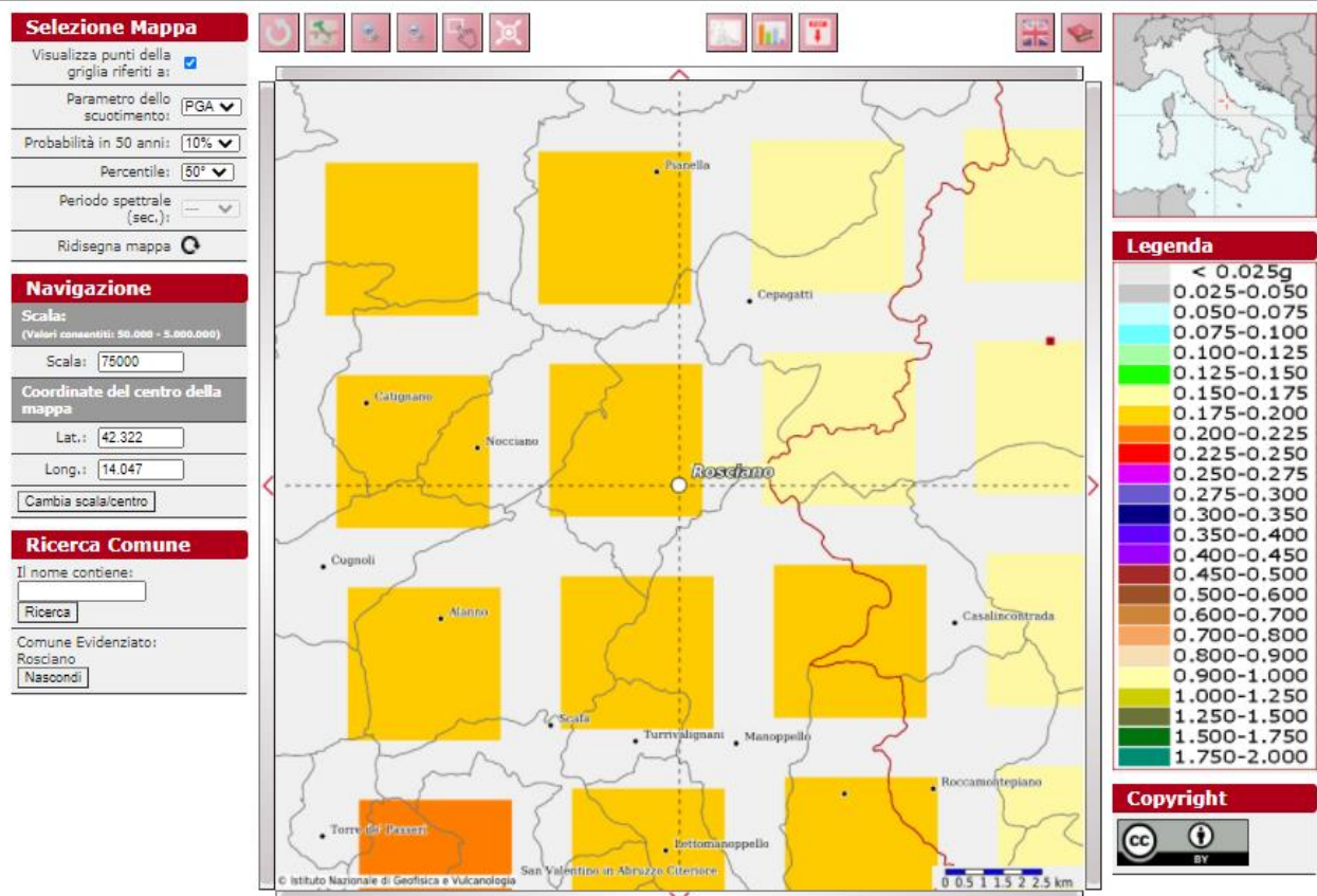
Fig. 2.22: Mappa di pericolosità sismica del comune di Rosciano.
