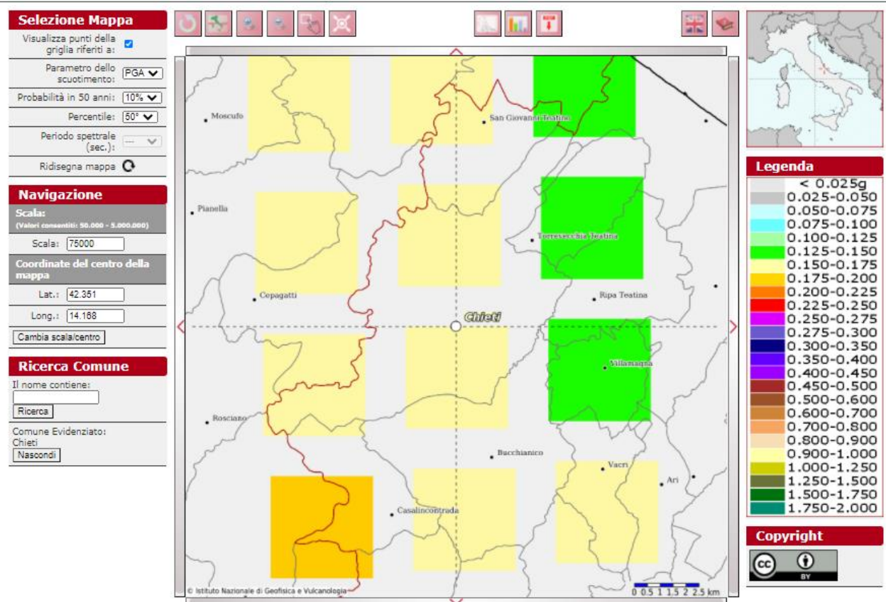
Fig. 2.20: Mappa di pericolosità sismica del comune di Chieti.
