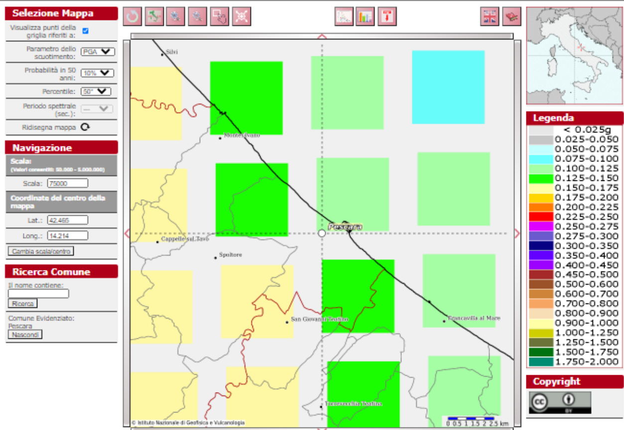
Fig. 2.14: Mappa di pericolosità sismica del comune di Pescara.
