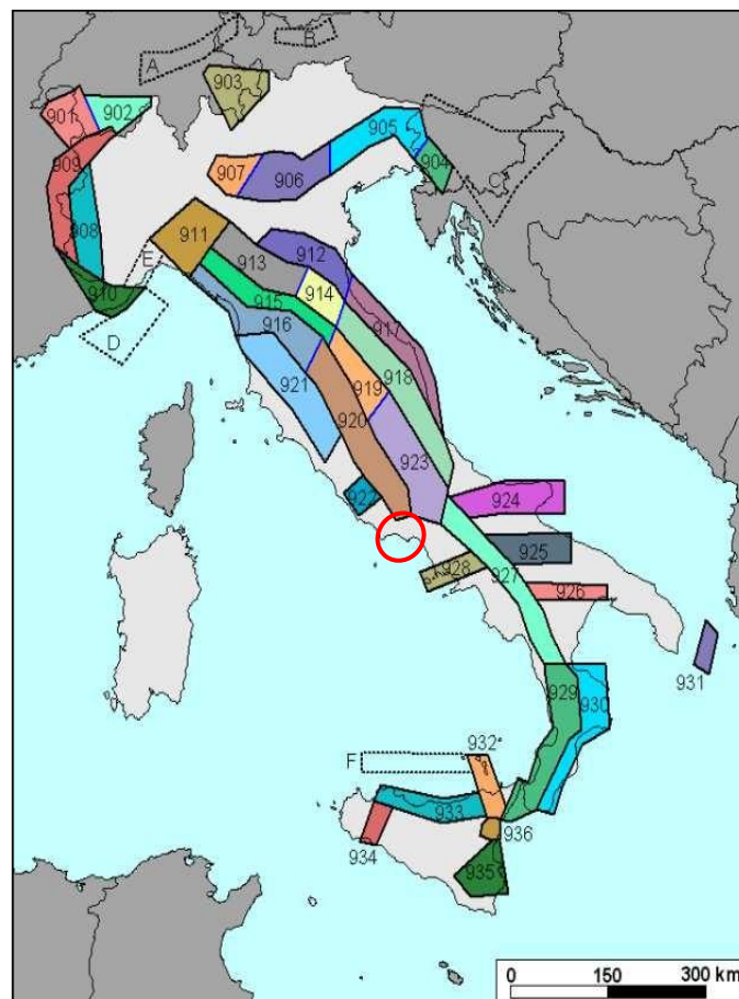
Fig. 2.28: Zonazione sismogenetica ZS9.
