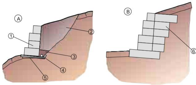
Fig. 10.1 - Struttura di sostegno in gabbioni.
