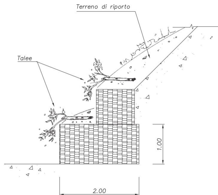
Fig. 10.6: Ricostruzione spondale con gabbioni interrati
