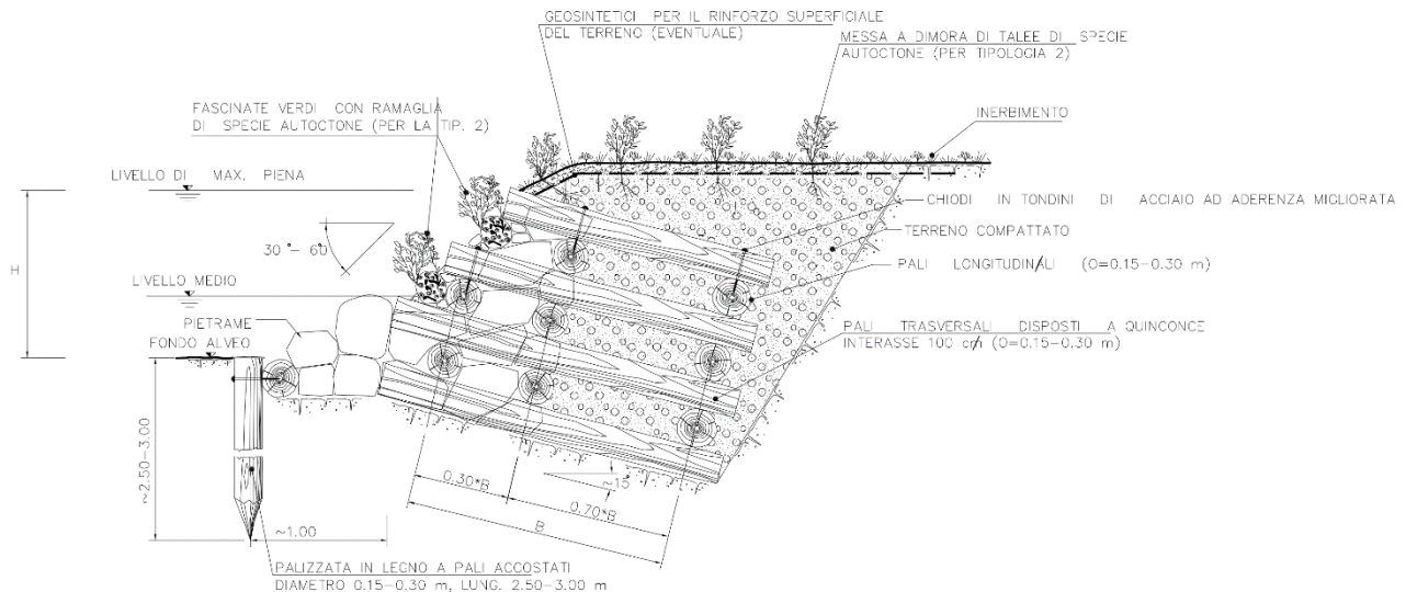
Fig. 10.7: Muro cellulare in legname e pietrame.
