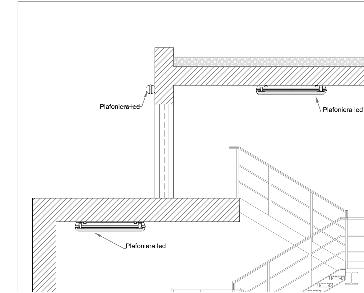
Tipologico illuminazione interni 1:50
