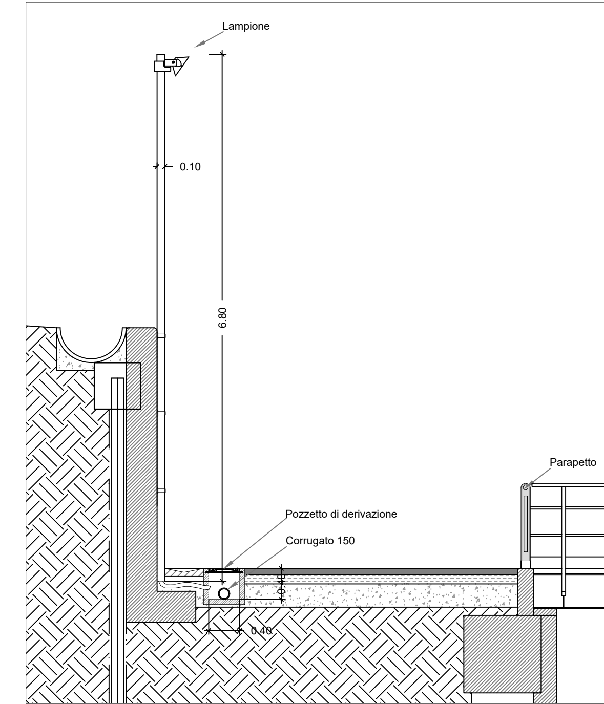
Tipologico illuminazione strada 1:50
