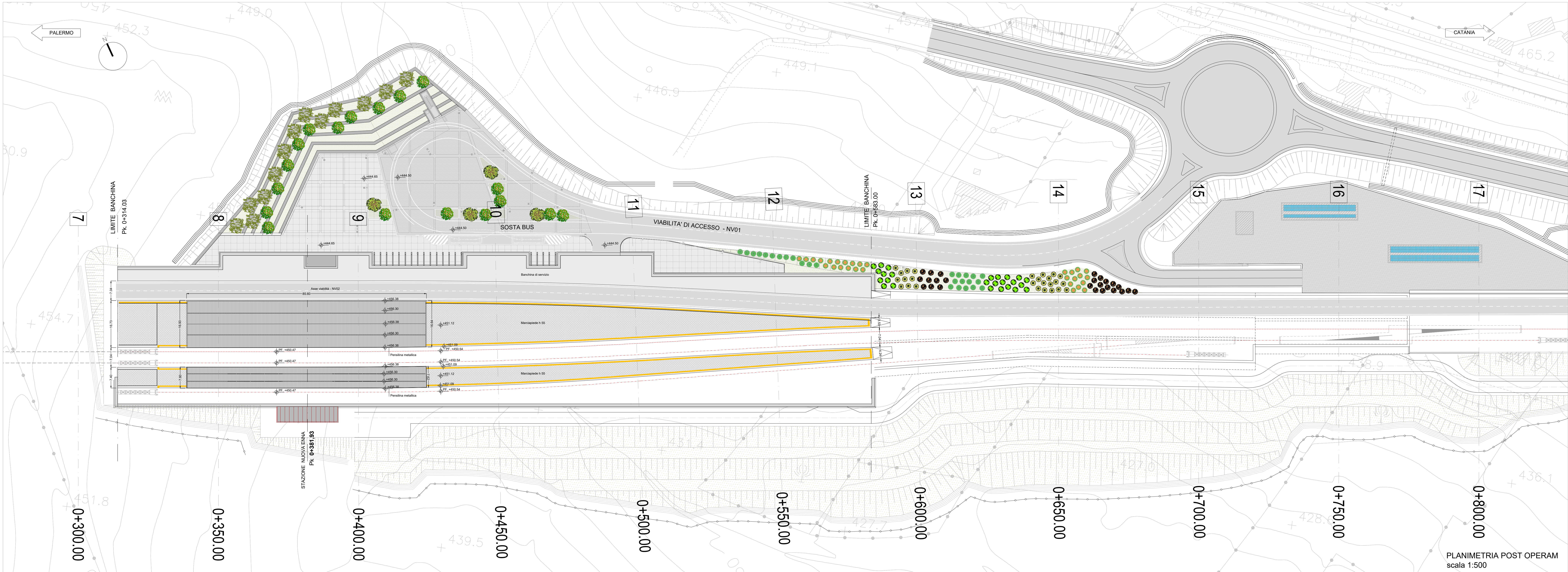
PLANIMETRIA ANTE OPERAM scala 1:500
