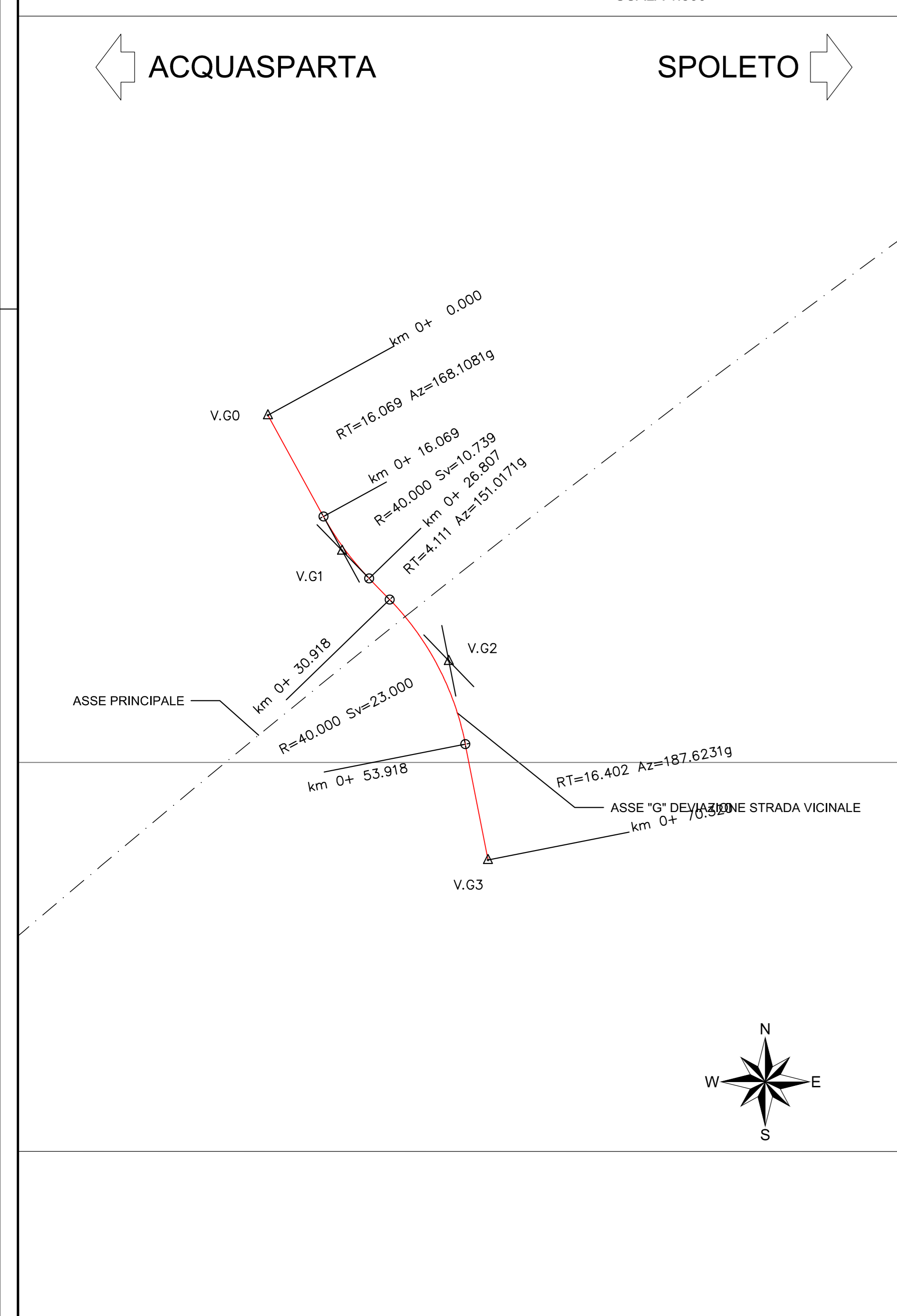
PLANIMETRIA DI TRACCIAMENTO SCALA 1:500
