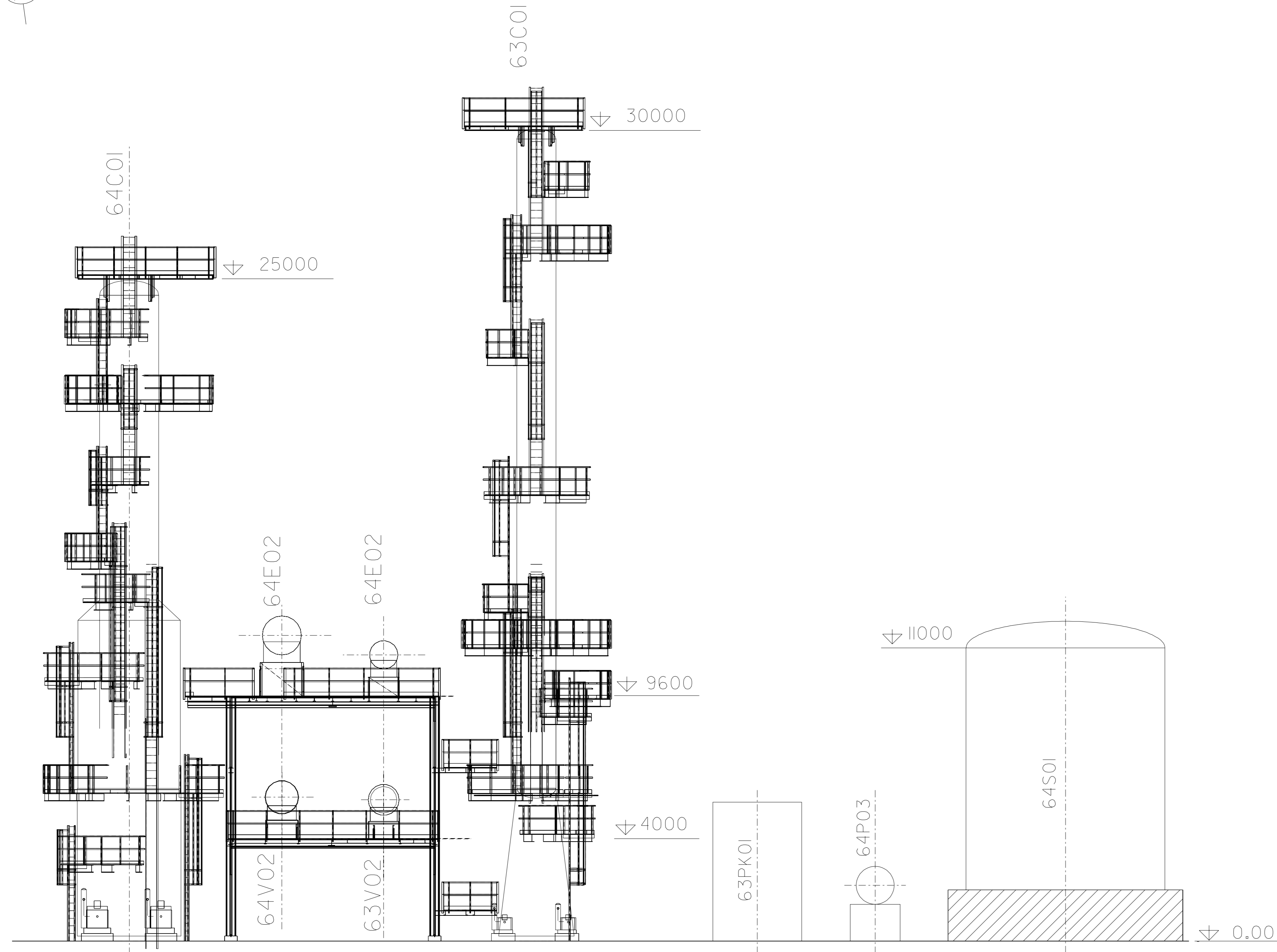
SEZIONE A-A
