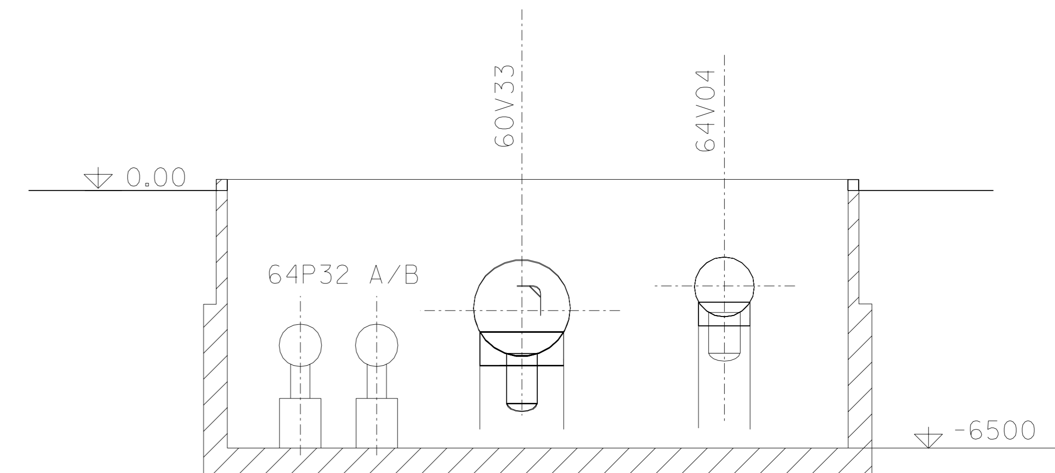
SEZIONE C-C
