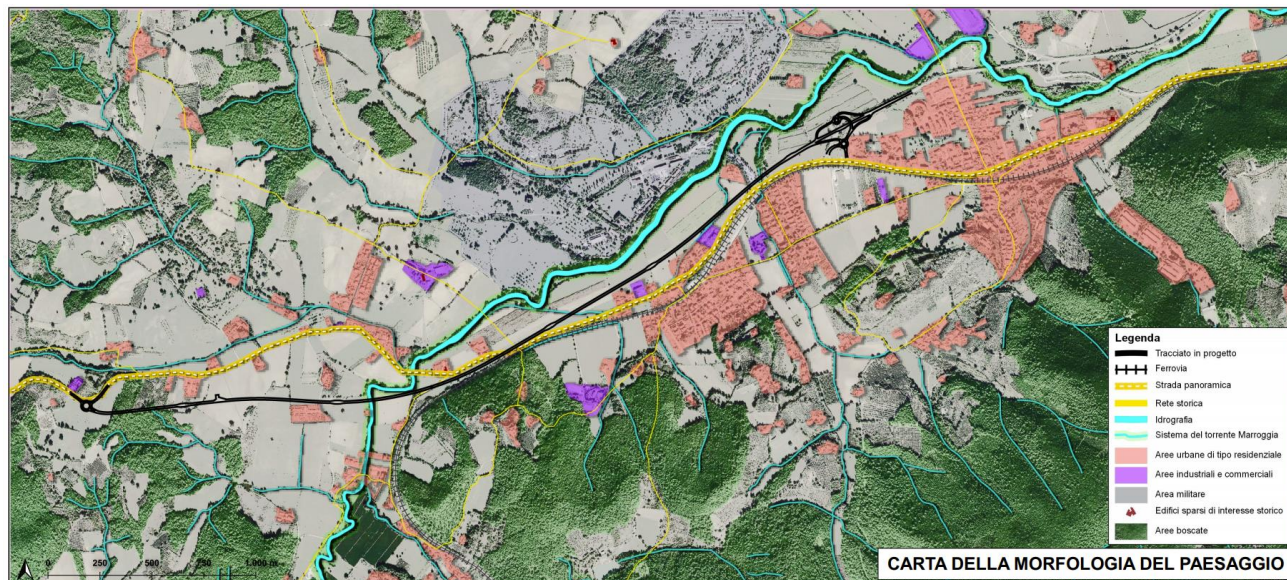
Figura 6 – Carta della morfologia del paesaggio
