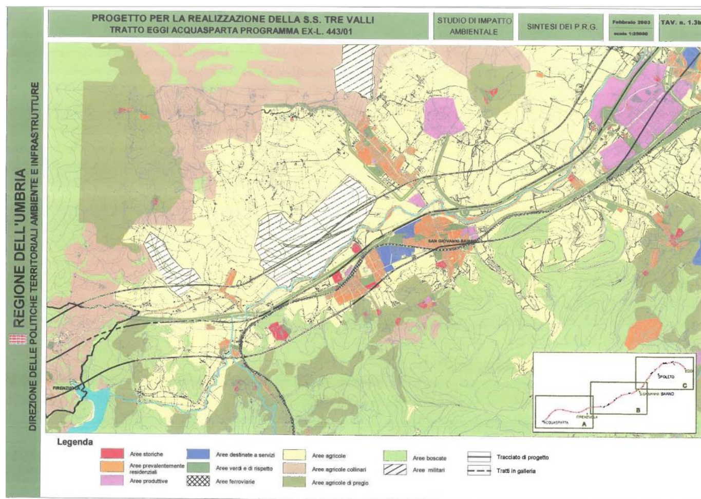
Figura 7 - Estratto dal SIA 2003 – Sintesi dei PRG
