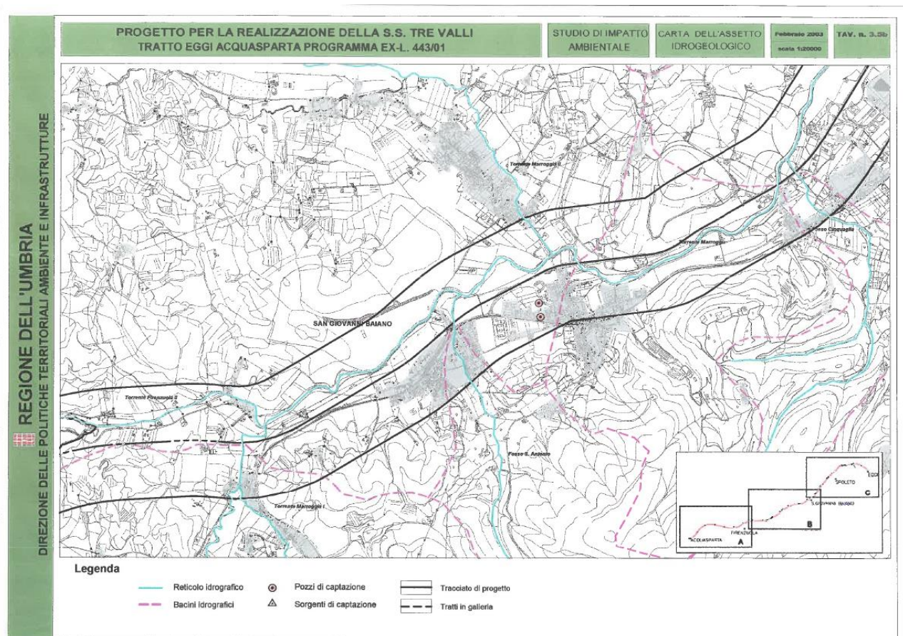
Figura 8 - Estratto dal SIA 2003 – Carta dell'assetto idrogeologico
