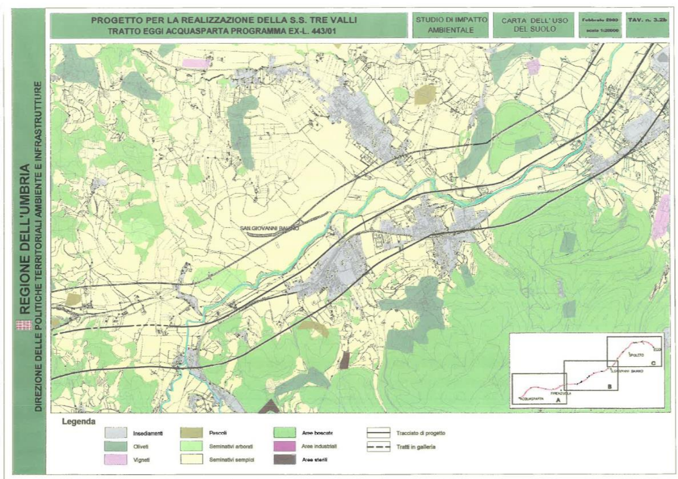
Figura 9 - Estratto dal SIA 2003 – Carta dell’uso del suolo
