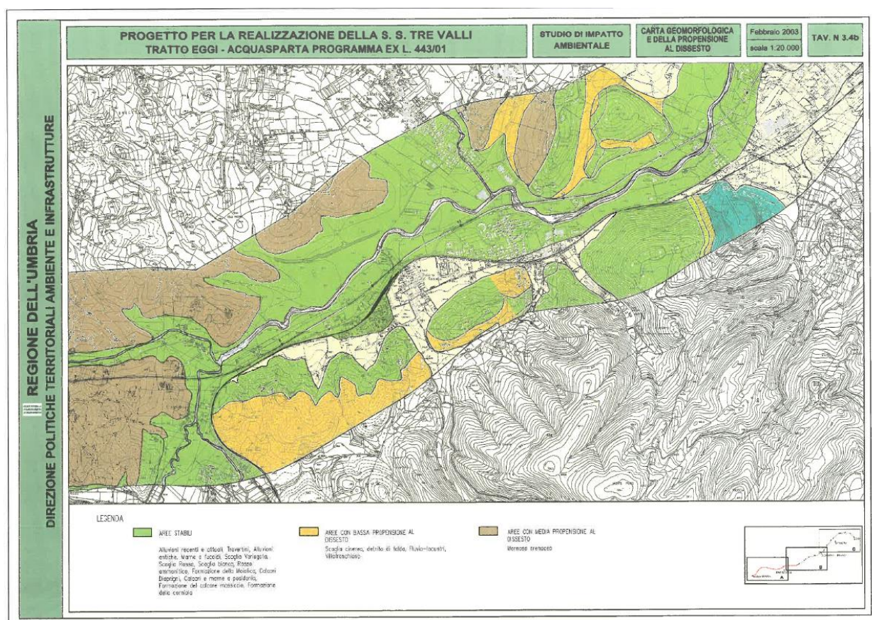
Figura 5 - Estratto dal SIA 2003 – Carta geomorfologica e della propensione al dissesto
