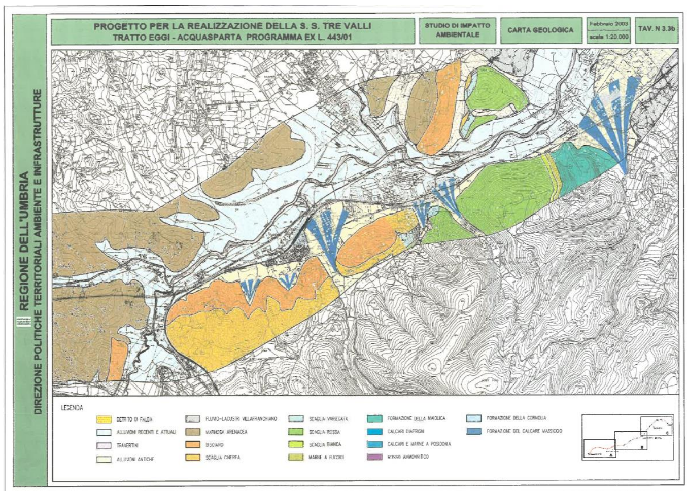
Figura 4 - Estratto dal SIA 2003 – Carta geologica
