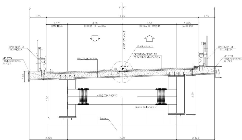
Figura 13 - Sezione Trasversale dell'impalcato del Viadotto Marroggia 1.
