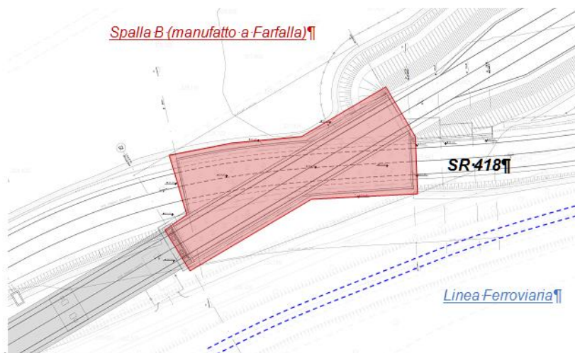
Figura 16 - Planimetria della Spalla B del Viadotto Marroggia 1.
