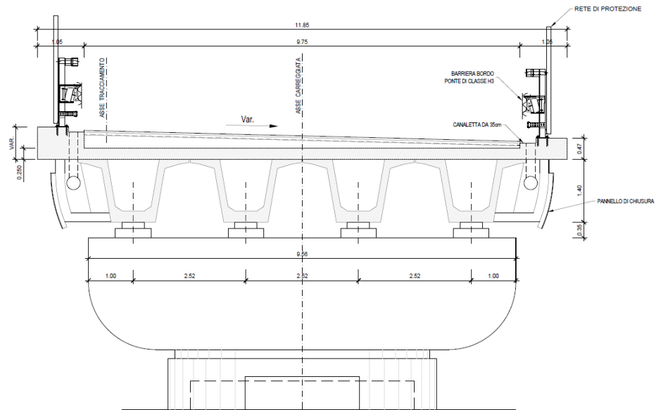
Figura 18 - Sezione Tipo Impalcato Viadotto Molino Vecchio.
