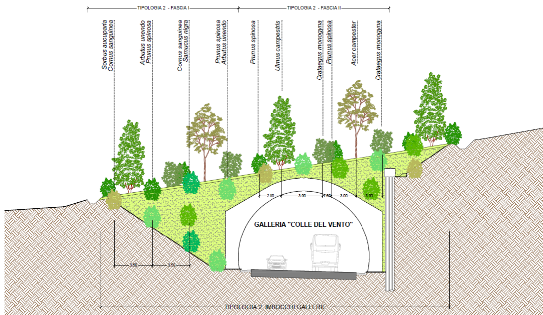
Figura 10 - Sezione trasversale Galleria artificiale Colle del Vento.
