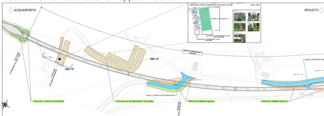
Figura 11 - Planimetria con l'evidenza delle opere di mitigazione ambientale del Viadotto Marroggia.
