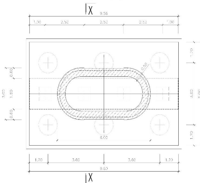
Figura 19: Sezione pila tipo A
