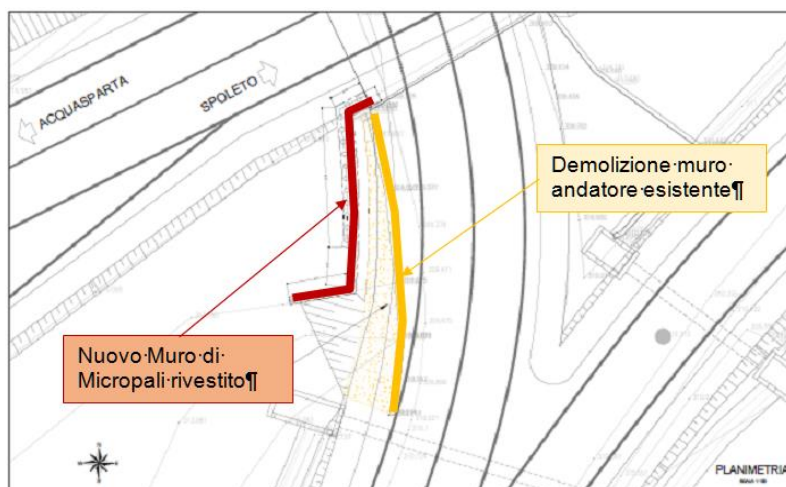
Figura 22 - Stralcio Planimetrico dello Svincolo di Baiano con l'evidenza della porzione del muro da demolire e del nuovo da costruire.
