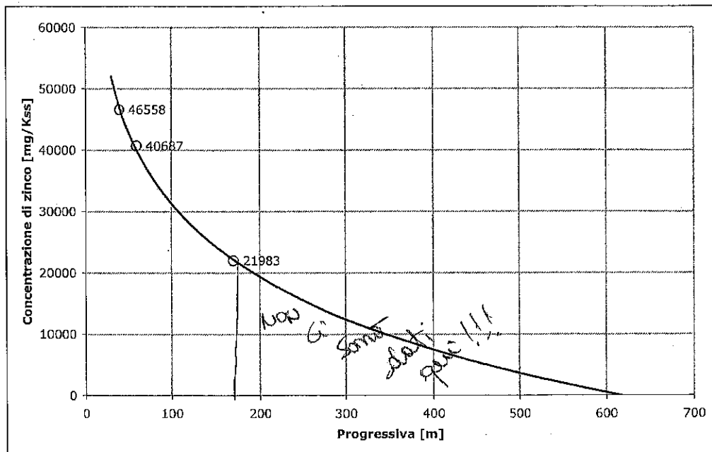
Figura 3- Profilo dell'andamento delle concentrazione di zinco verso valle
