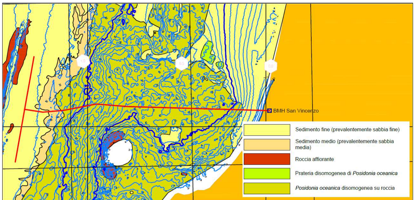
Figura 2.2.1: Dettaglio dell'attraversamento del posidonieto da parte del cavo di elettrodo in località La Torraccia nel comune di San Vincenzo (rilievi SSS e MBEAM survey marina preliminare, Terna 2020)
