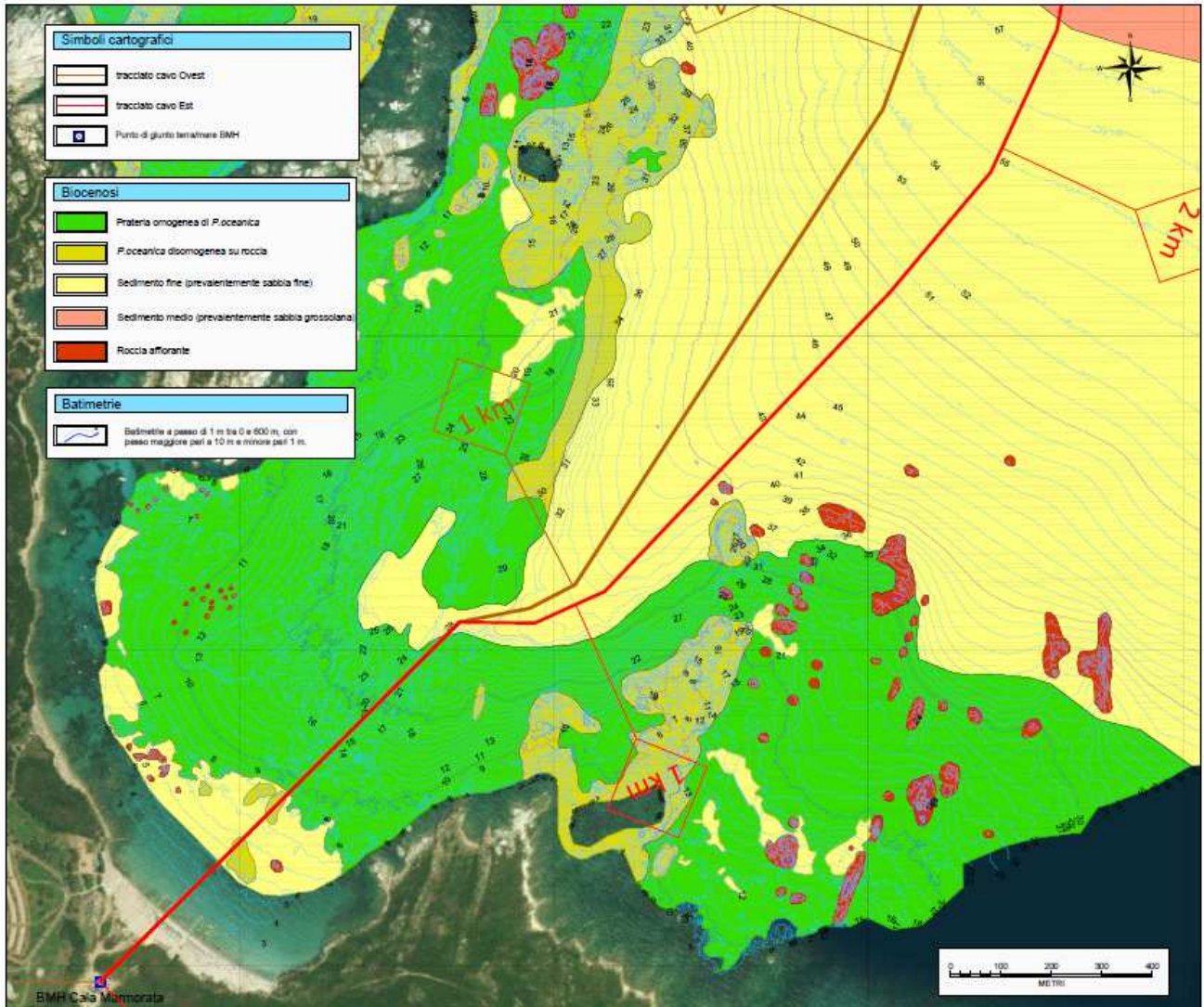
Figura 2.3.1: Dettaglio dell'attraversamento del posidonieto da parte di cavi di polo a Cala Marmorata, nel comune di Santa Teresa (rilievi SSS e MBEAM survey marina preliminare, Terna 2020)
