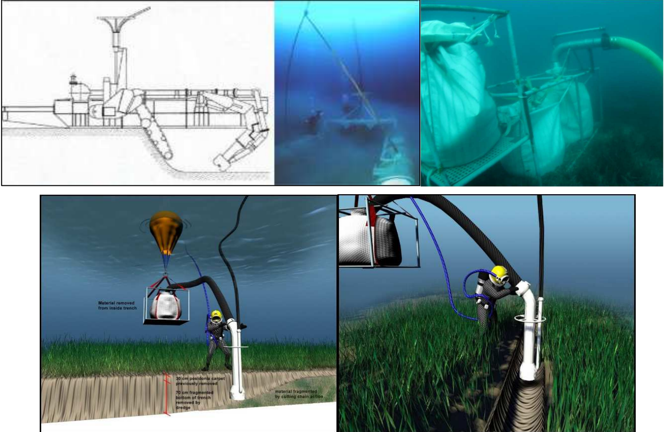
Figura 4.1: Macchina per il trenching a galleggiamento controllato, strumento per l’aspirazione e raccolta del materiale movimentato
