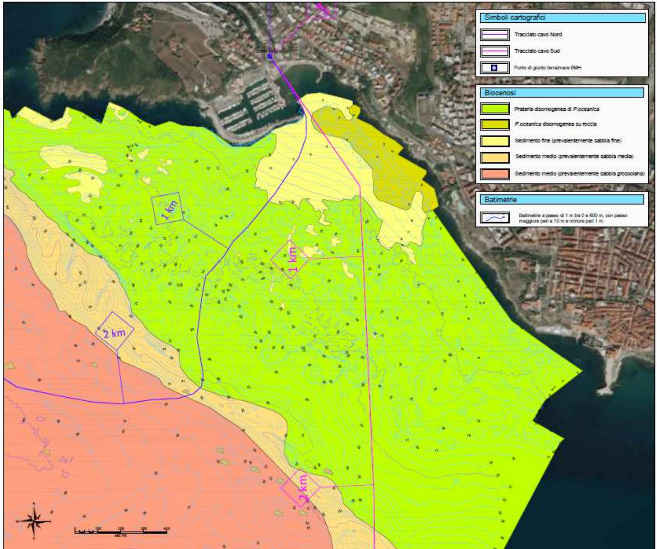
Figura 2.1.1: Dettaglio dell'attraversamento del posidonieto all'approdo di Salivoli (rilievi SSS e MBEAM survey marina preliminare, Terna 2020)
