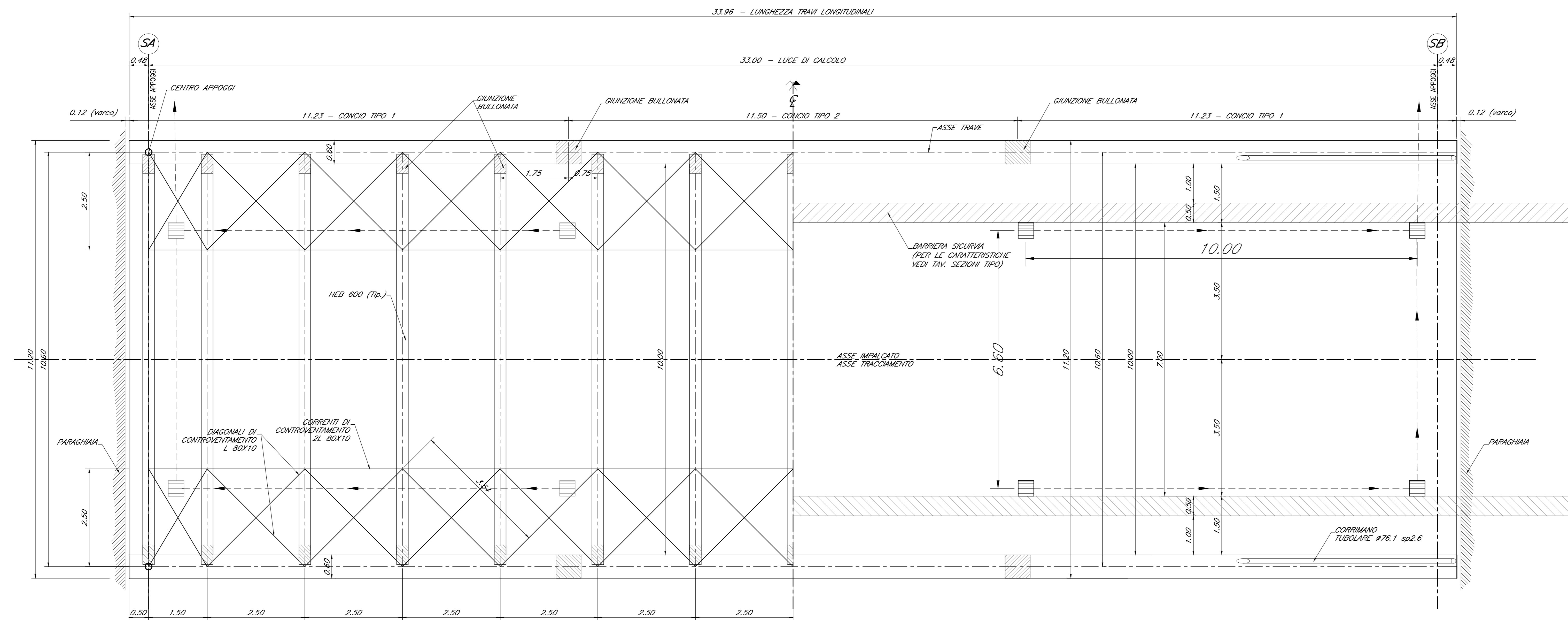
1/2 PIANTE INFERIORE SCALA 1:50
