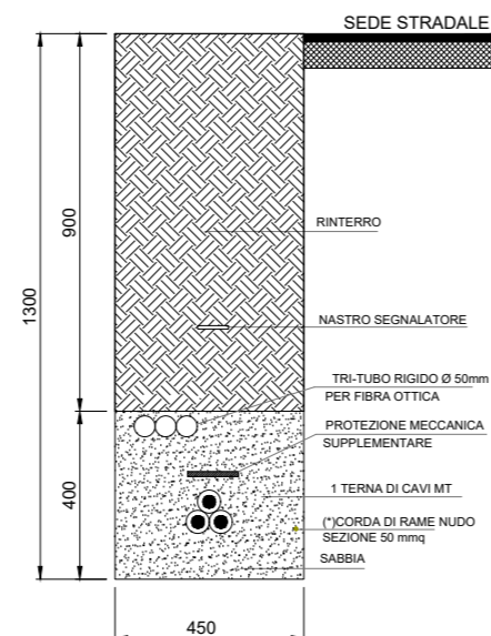
SEZIONE C-C CAVIDOTTO MT INTERRATO - 1 TERNA DI CAVI PERCORSO IN BANCHINA STRADA VICINALE/COMUNALE
