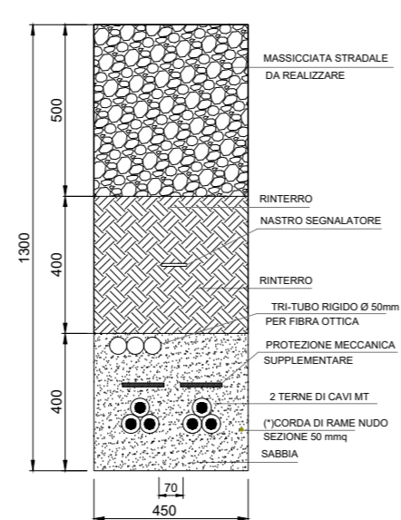
SEZIONE G-G CAVIDOTTO MT INTERRATO - 3 TERNE DI CAVI PERCORSO STRADA DI CANTIERE
