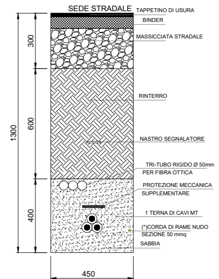
SEZIONE I-I CAVIDOTTO MT INTERRATO - 1 TERNA DI CAVI PERCORSO SOTTO VICINALE/COMUNALE
