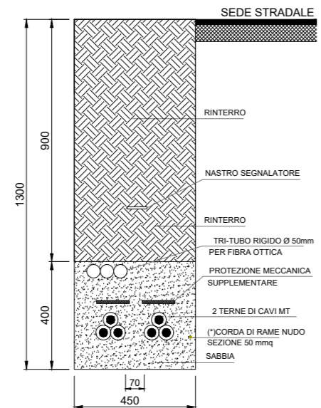
SEZIONE F-F CAVIDOTTO MT INTERRATO - 2 TERNE DI CAVI PERCORSO IN BANCHINA STRADA PROVINCIALE
