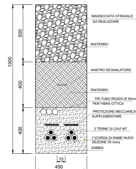
SEZIONE D-D CAVIDOTTO MT INTERRATO - 2 TERNE DI CAVI PERCORSO STRADA DI CANTIERE
