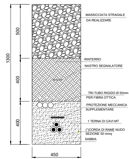
SEZIONE A-A CAVIDOTTO MT INTERRATO - 1 TERNA DI CAVI PERCORSO STRADA DI CANTIERE
