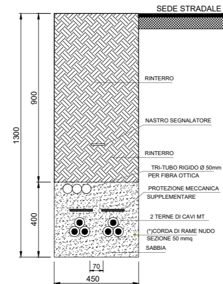
SEZIONE H-H CAVIDOTTO MT INTERRATO - 2 TERNE DI CAVI PERCORSO IN BANCHINA STRADA VICINALE/COMUNALE
