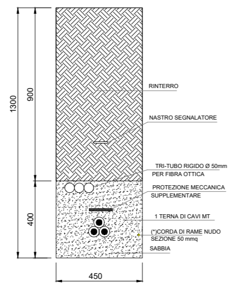
SEZIONE B-B CAVIDOTTO MT INTERRATO - 1 TERNA DI CAVI PERCORSO IN TERRENO
