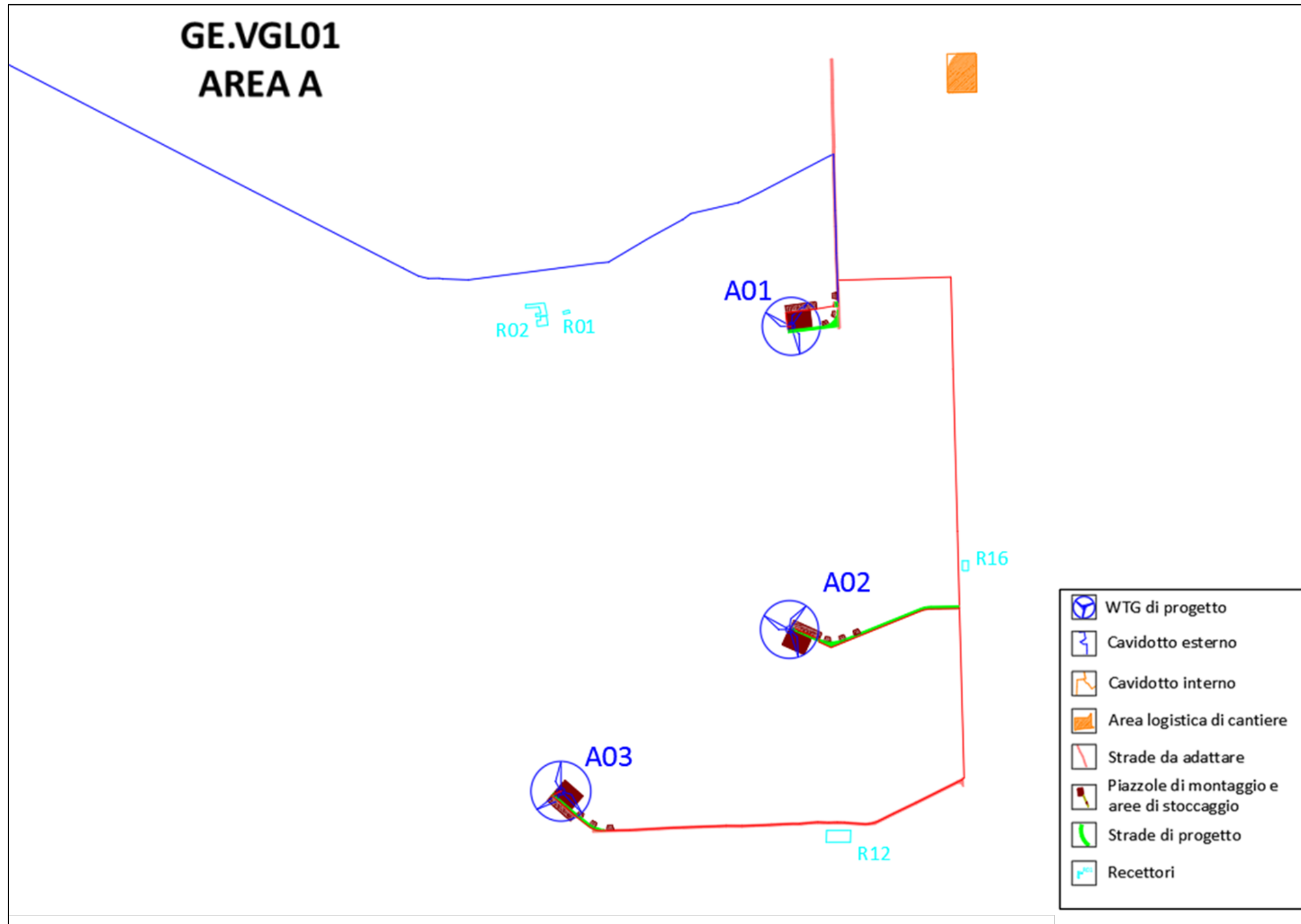
Figura 4: Inquadramento della viabilità di cantiere e delle aree di lavoro fisse e mobili – AREA A.
