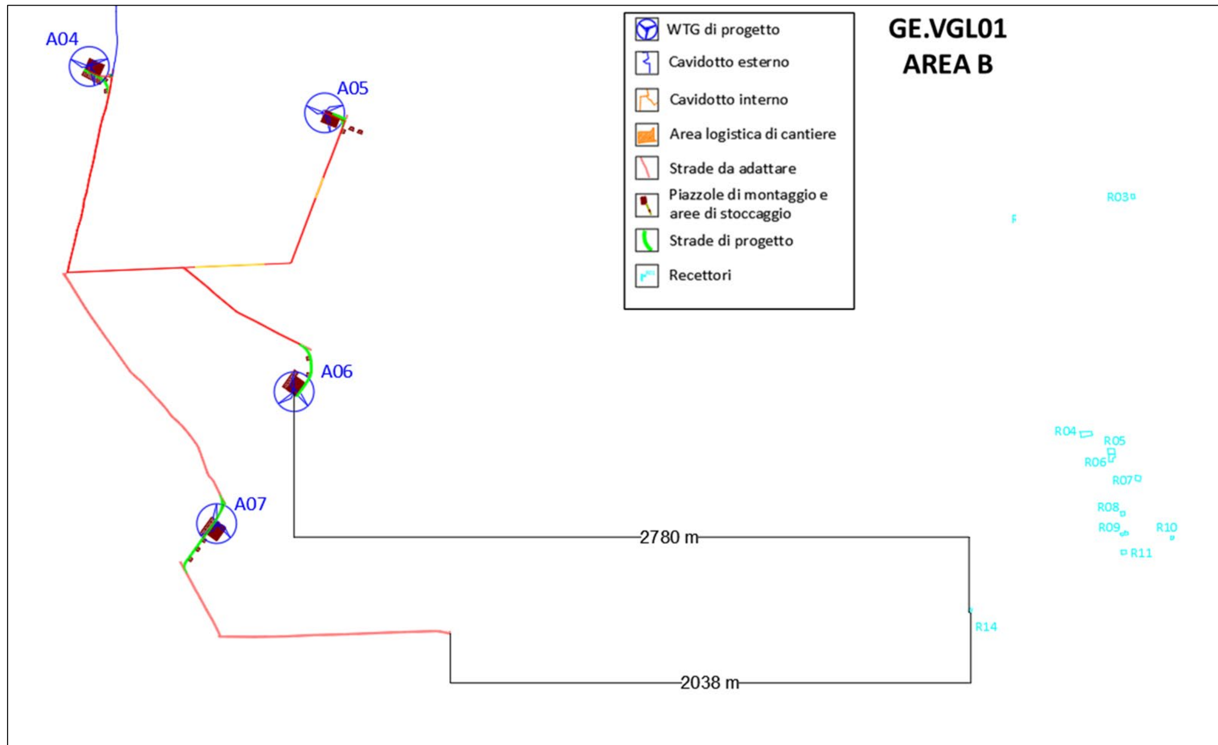
Figura 5: Inquadramento della viabilità di cantiere e delle aree di lavoro fisse e mobili con evidenza della distanza intercorrente tra il recettore R14, la turbina più prossima e la strada di cantiere più vicina da realizzare – AREA B.
