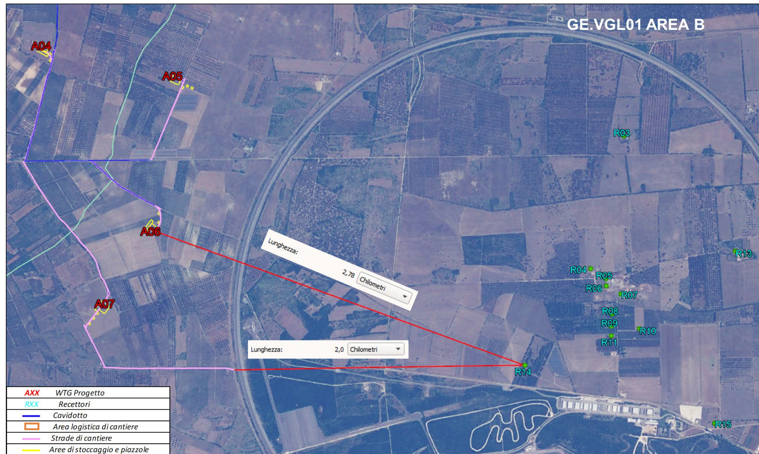
Figura 3: inquadramento territoriale dell'Area B dei recettori relativi su orto foto piana estratta da Google Earth ed evidenza della distanza intercorrente tra il recettore R14, la turbina più prossima e la strada di cantiere più vicina da realizzare.
