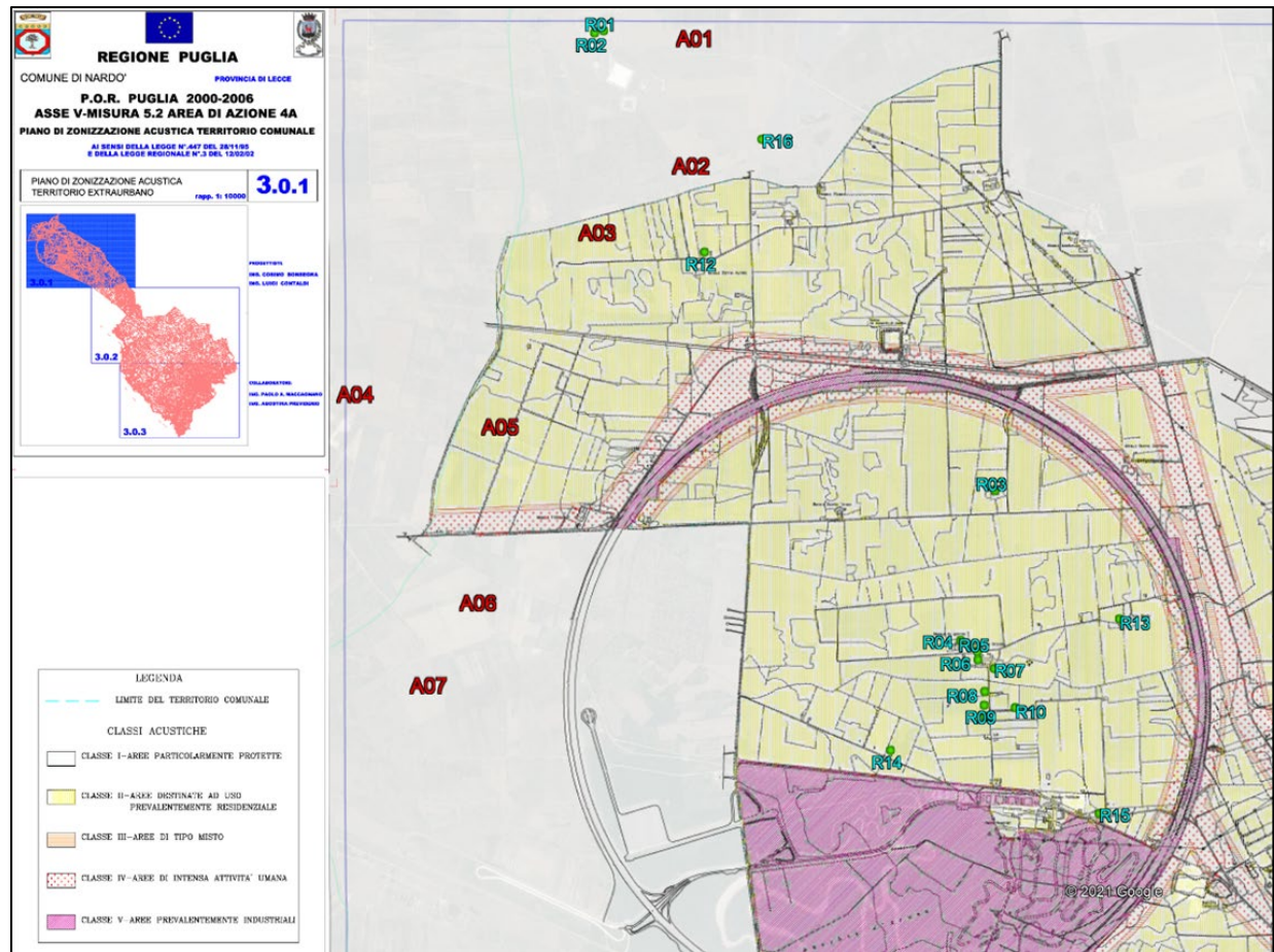
Figura 7: Stralcio del PZA del comune di Nardò con evidenza della disposizione del layout di impianto e dei recettori sensibili considerati nell'analisi.
