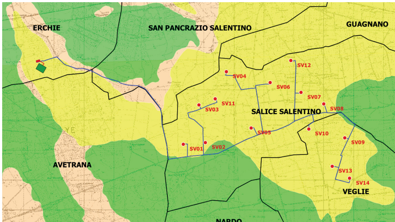
Figura 4: – Stralcio della litologia dell'area di studio (Carta Idrogeomorfologica: www.sit.puglia.it )
