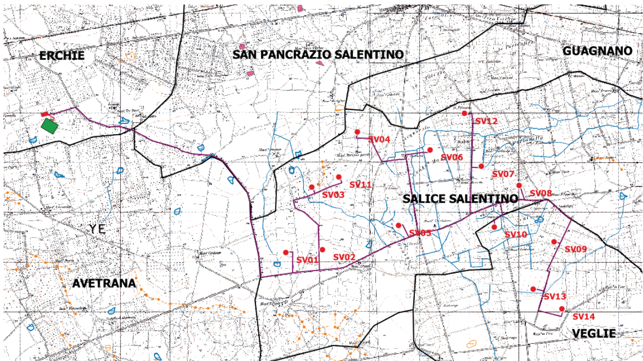
Figura 5: - Stralcio della Carta Idrogeomorfologica ( www.sit.puglia.it )
