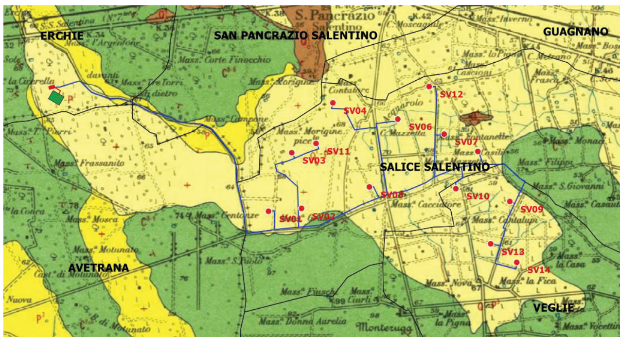
Figura 3: - Stralcio della Carta Geologica scala 1:100.000 Foglio n° 203 "Brindisi" con ubicazione dell'area di studio
