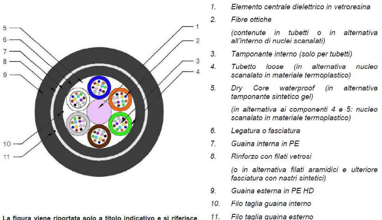
Fig.: Sezione tipo del cavo ottico
