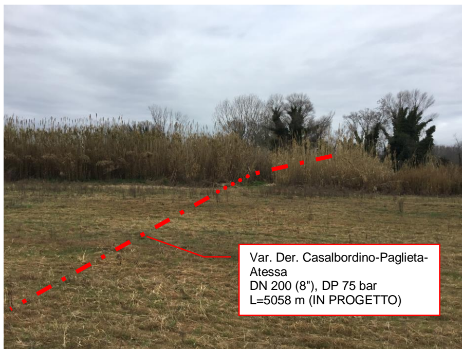
Foto n.12 – Var. Der. Casalbordino-Paglieta-Atessa DN 200 (8"), DP 75 bar (in progetto) con attraversamento fosso
