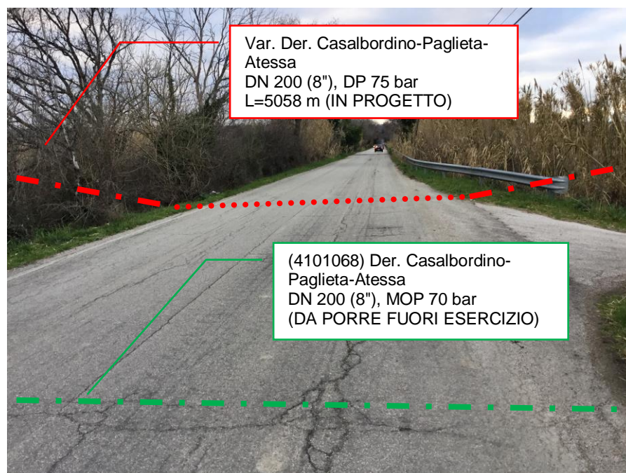
Foto n.8 – Vista metanodotto in progetto con attraversamento strada e metanodotto da porre fuori esercizio
