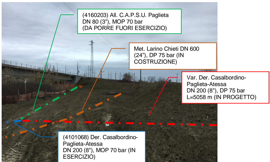
Foto n.14 – Metanodotti in progetto e da porre fuori esercizio
