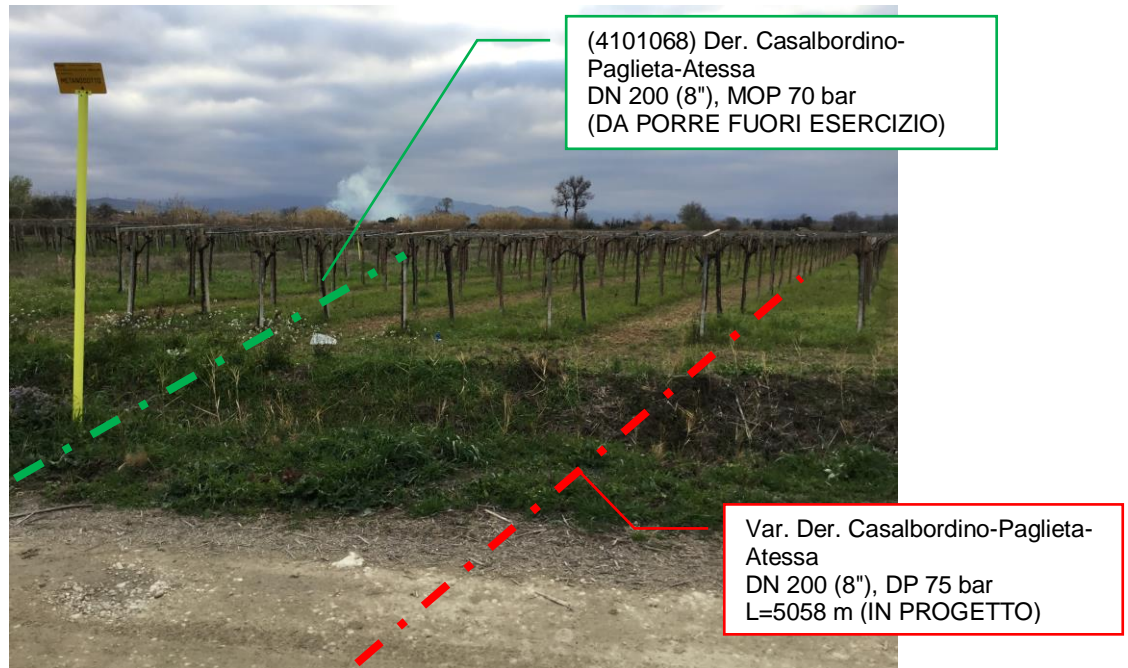
Foto n.7 – Panoramica metanodotti in progetto e da porre fuori esercizio
