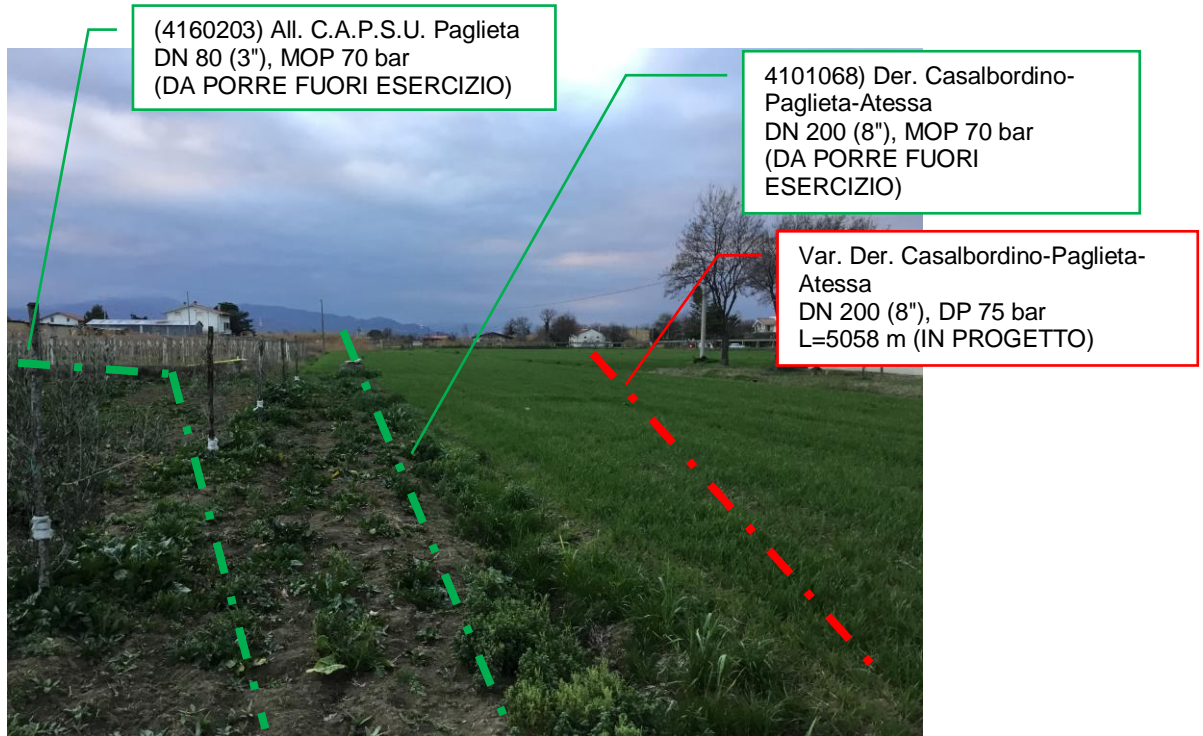
Foto n.9 – Panoramica metanodotto in progetto e metanodotti da porre fuori esercizio
