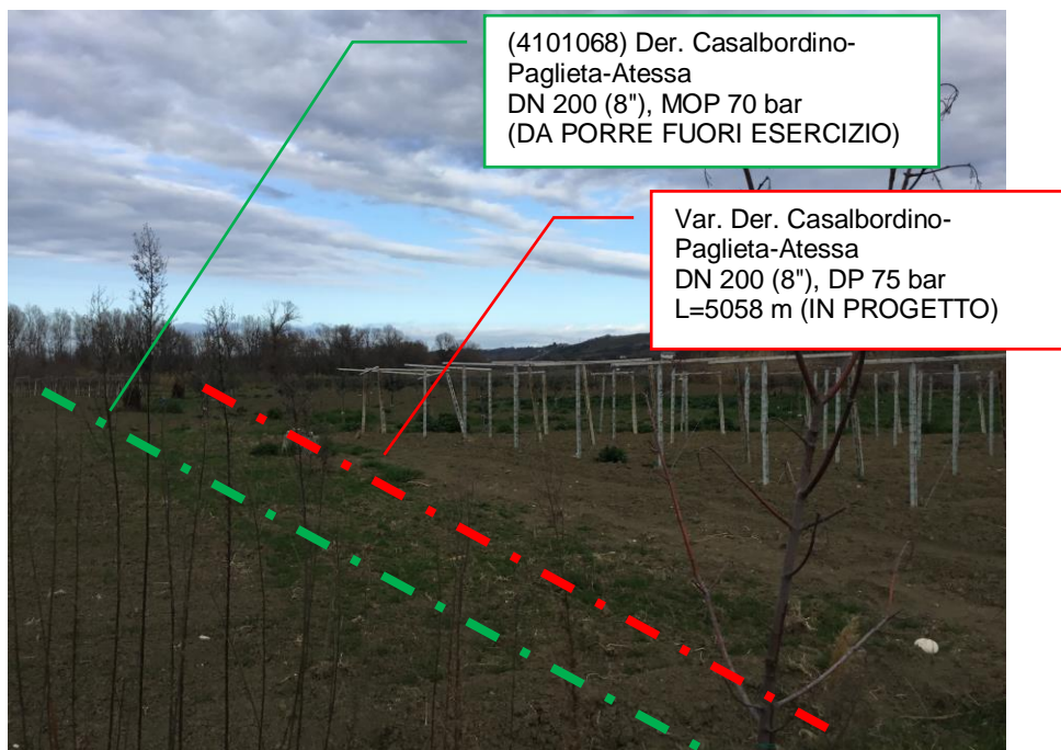
Foto n.5 – Vista metanodotto in progetto e metanodotto da porre fuori esercizio
