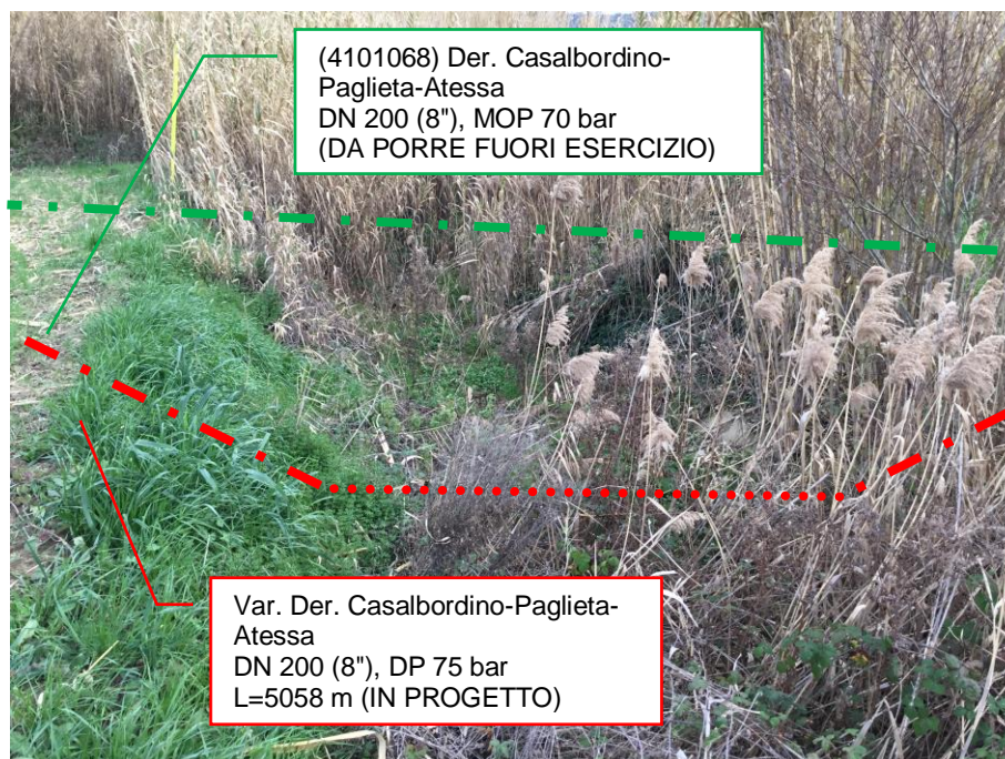
Foto n.6 – Vista metanodotto in progetto con attraversamento fosso e metanodotto da porre fuori esercizio
